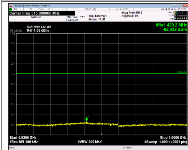
41(2555-2655)-41(2555-2655)-10MHz-20MHz-16QAM-16 QAM-40295-40439-1RB#0-1RB#99-30~1000MHz-PASS
