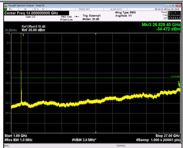
41(2555-2655)-41(2555-2655)-10MHz-20MHz-16QAM-16Q AM-40295-40439-1RB#0-1RB#99-1000~27000MHz-PASS
