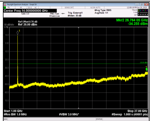
41(2555-2655)-41(2555-2655)-15MHz-10MHz-QPSK-QPS K-40315-40435-1RB#74-ORB#0-1000~27000MHz-PASS
