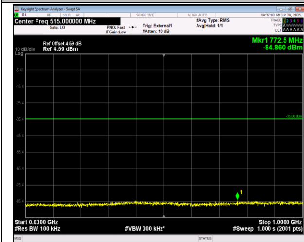
41(2555-2655)-41(2555-2655)-10MHz-20MHz-QPSK-QP SK-40295-40439-1RB#49-ORB#0-30~1000MHz-PASS
