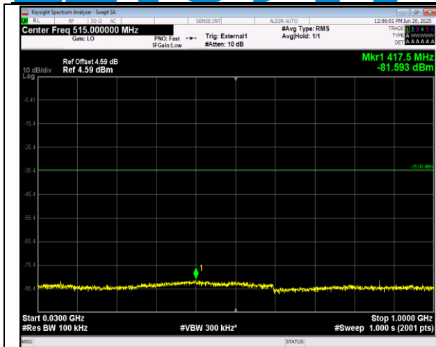
41(2555-2655)-41(2555-2655)-15MHz-10MHz-QPSK-QP SK-40315-40435-75RB#0-50RB#0-30~1000MHz-PASS
