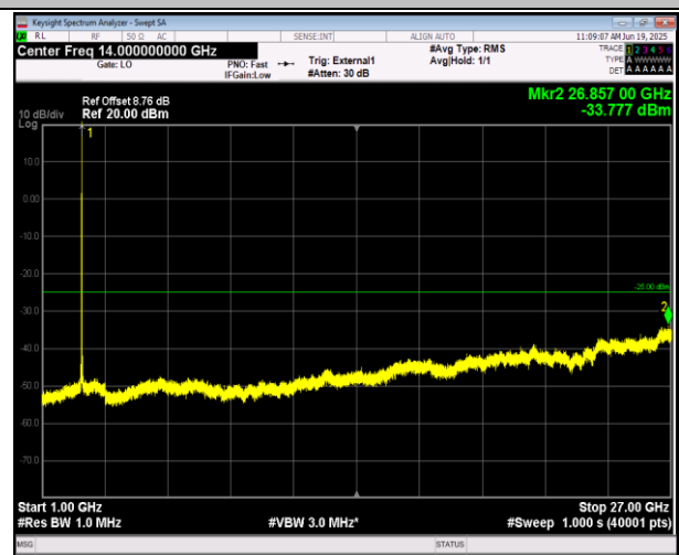
41(2555-2655)-41(2555-2655)-10MHz-15MHz-QPSK-QPS K-41045-41165-50RB#0-75RB#0-1000~27000MHz-PASS
