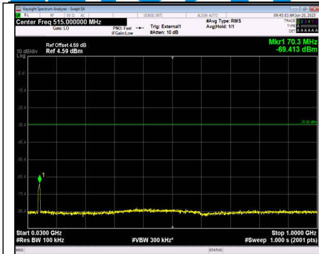
41(2555-2655)-41(2555-2655)-15MHz-10MHz-QPSK-QP SK-40315-40435-1RB#0-ORB#0-30~1000MHz-PASS
