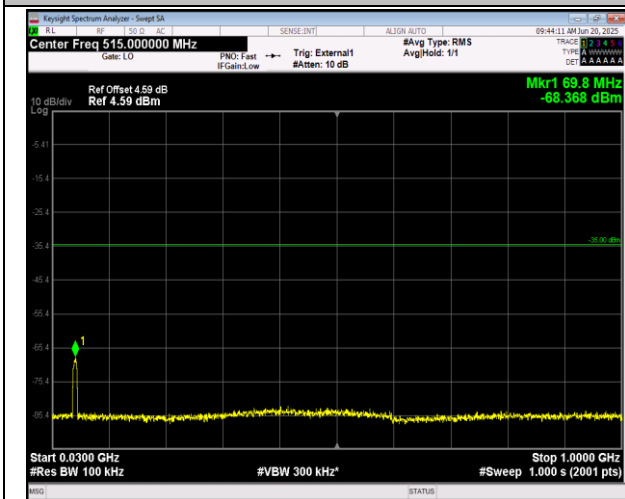
41(2555-2655)-41(2555-2655)-10MHz-20MHz-16QAM-16 QAM-40996-41140-1RB#0-ORB#0-30~1000MHz-PASS
