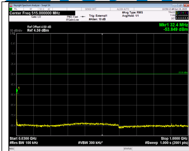
41(2555-2655)-41(2555-2655)-10MHz-15MHz-QPSK-QP SK-40669-40789-1RB#0-1RB#74-30~1000MHz-PASS
