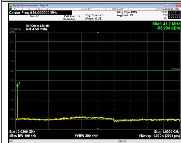
41(2555-2655)-41(2555-2655)-10MHz-15MHz-QPSK-QP SK-40669-40789-50RB#0-75RB#0-30~1000MHz-PASS
