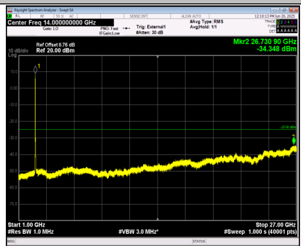
41(2555-2655)-41(2555-2655)-15MHz-10MHz-16QAM-16Q AM-40315-40435-1RB#0-0RB#0-1000~27000MHz-PASS
