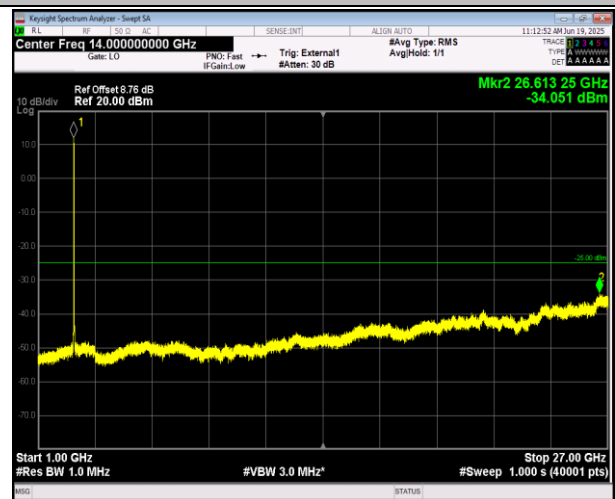
41(2555-2655)-41(2555-2655)-10MHz-15MHz-16QAM-16Q AM-41045-41165-1RB#0-ORB#0-1000~27000MHz-PASS
