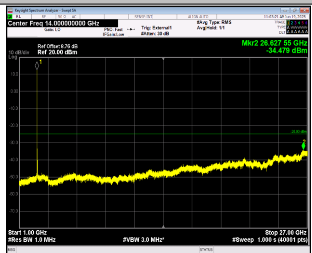
41(2555-2655)-41(2555-2655)-10MHz-15MHz-QPSK-QPS K-40669-40789-1RB#49-0RB#0-1000~27000MHz-PASS
