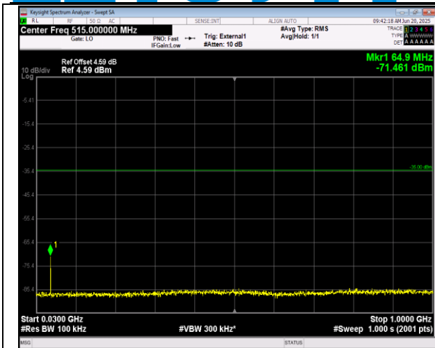
41(2555-2655)-41(2555-2655)-10MHz-20MHz-QPSK-QP SK-40996-41140-1RB#49-ORB#0-30~1000MHz-PASS
