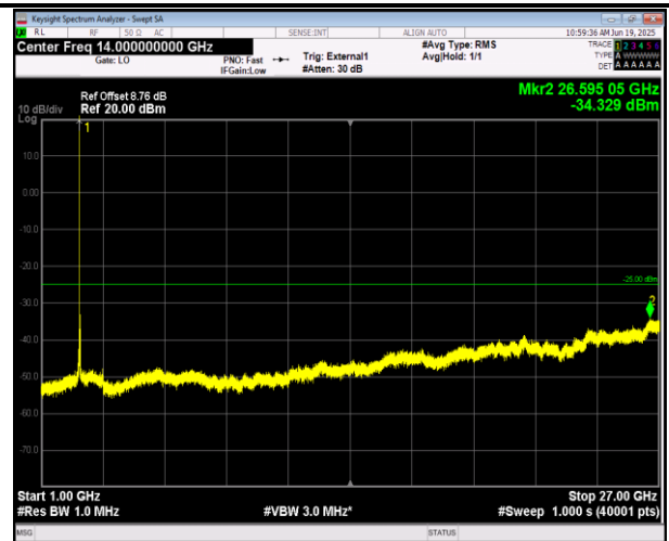
41(2555-2655)-41(2555-2655)-10MHz-15MHz-QPSK-QPS K-40669-40789-1RB#0-1RB#74-1000~27000MHz-PASS
