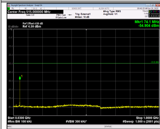
41(2555-2655)-41(2555-2655)-10MHz-20MHz-QPSK-QP SK-40996-41140-50RB#0-100RB#0-30~1000MHz-PASS
