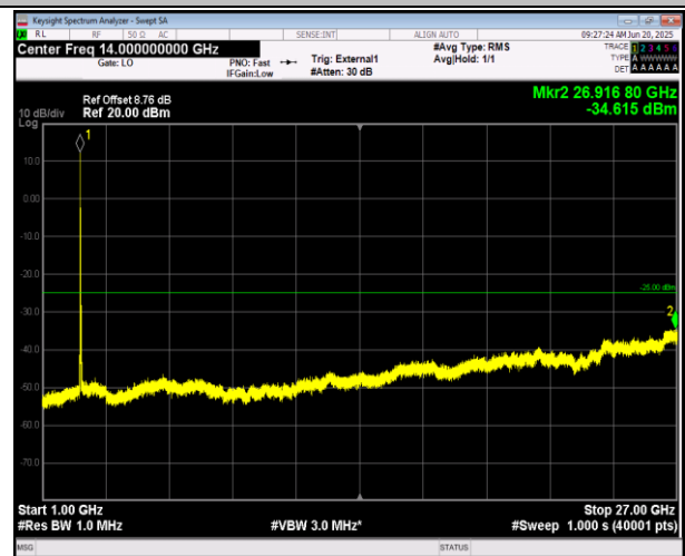
41(2555-2655)-41(2555-2655)-10MHz-20MHz-QPSK-QPS K-40295-40439-1RB#49-ORB#0-1000~27000MHz-PASS
