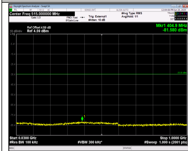
41(2555-2655)-41(2555-2655)-15MHz-10MHz-QPSK-QP SK-40315-40435-1RB#0-1RB#49-30~1000MHz-PASS
