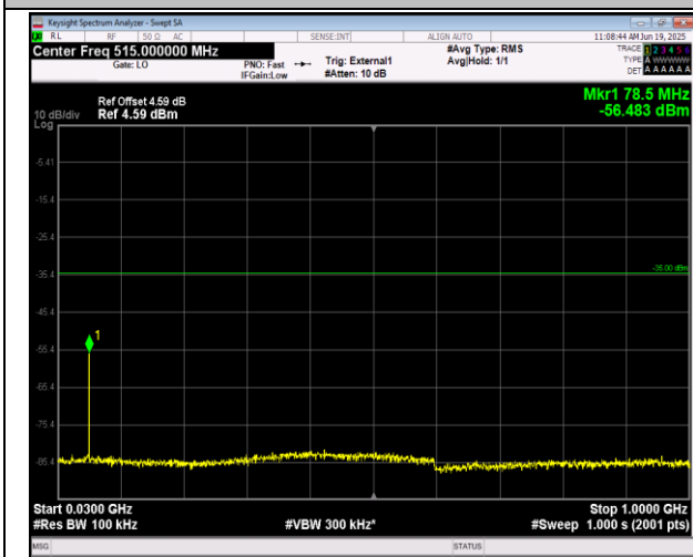
41(2555-2655)-41(2555-2655)-10MHz-15MHz-QPSK-QP SK-41045-41165-50RB#0-75RB#0-30~1000MHz-PASS
