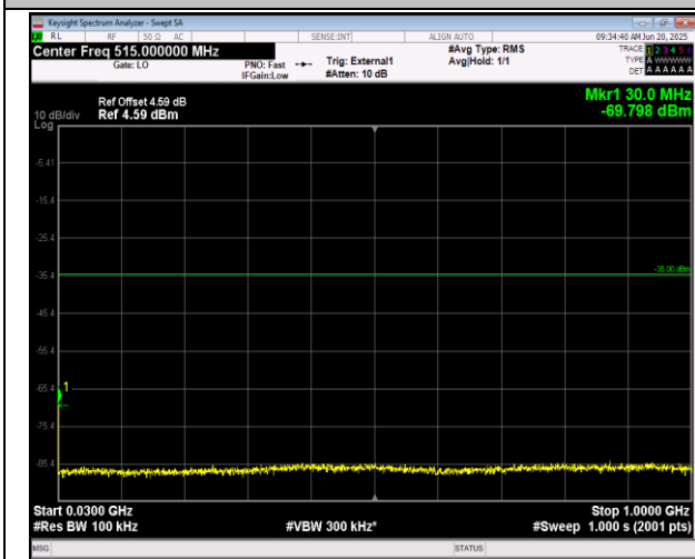
41(2555-2655)-41(2555-2655)-10MHz-20MHz-QPSK-QP SK-40646-40790-1RB#49-0RB#0-30~1000MHz-PASS
