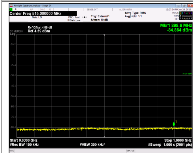
41(2555-2655)-41(2555-2655)-15MHz-10MHz-QPSK-QP SK-40315-40435-1RB#74-ORB#0-30~1000MHz-PASS
