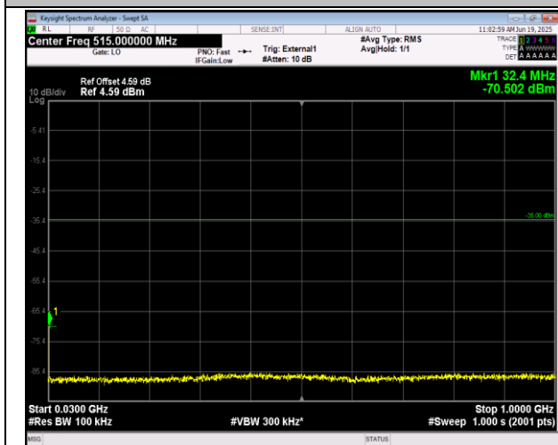
41(2555-2655)-41(2555-2655)-10MHz-15MHz-QPSK-QP SK-40669-40789-1RB#49-0RB#0-30~1000MHz-PASS
