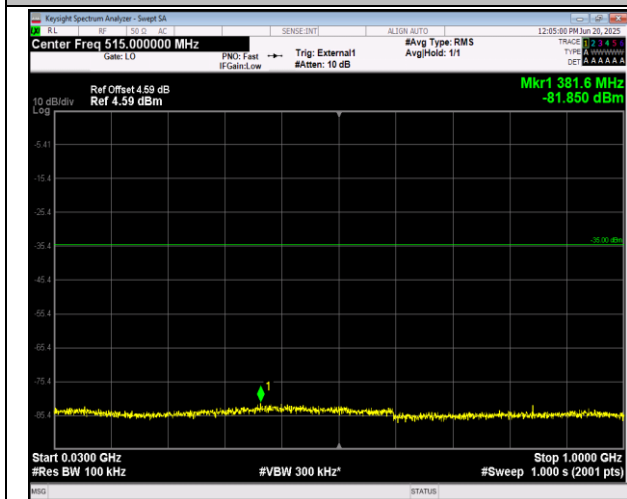
41(2555-2655)-41(2555-2655)-15MHz-10MHz-16QAM-16 QAM-40315-40435-1RB#0-1RB#49-30~1000MHz-PASS
