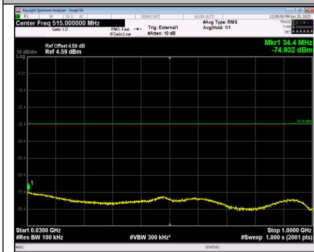
41(2555-2655)-41(2555-2655)-15MHz-10MHz-16QAM-16 QAM-40315-40435-1RB#0-0RB#0-30~1000MHz-PASS
