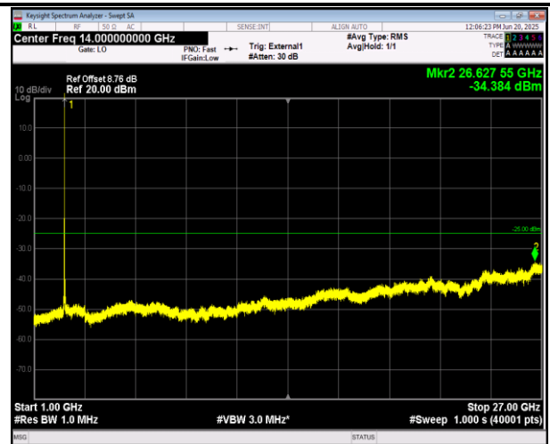
41(2555-2655)-41(2555-2655)-15MHz-10MHz-QPSK-QPS K-40315-40435-75RB#0-50RB#0-1000~27000MHz-PASS
