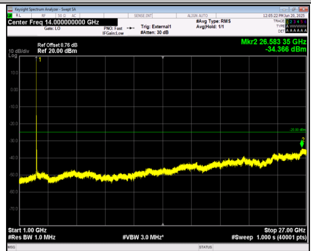
41(2555-2655)-41(2555-2655)-15MHz-10MHz-16QAM-16Q AM-40315-40435-1RB#0-1RB#49-1000~27000MHz-PASS
