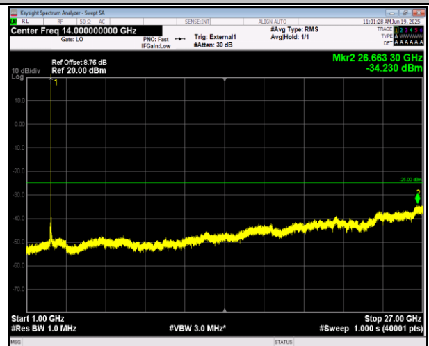
41(2555-2655)-41(2555-2655)-10MHz-15MHz-QPSK-QPS K-40669-40789-50RB#0-75RB#0-1000~27000MHz-PASS
