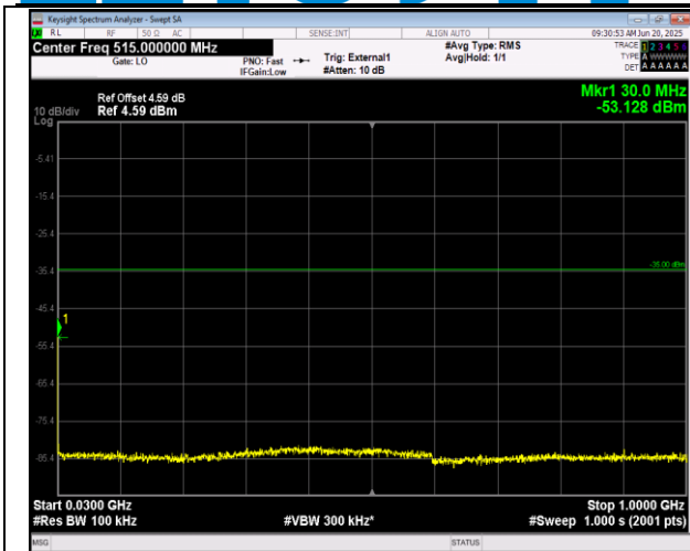
41(2555-2655)-41(2555-2655)-10MHz-20MHz-QPSK-QP SK-40646-40790-1RB#0-1RB#99-30~1000MHz-PASS
