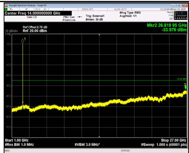
41(2555-2655)-41(2555-2655)-10MHz-20MHz-QPSK-QPS K-40295-40439-1RB#0-ORB#0-1000~27000MHz-PASS
