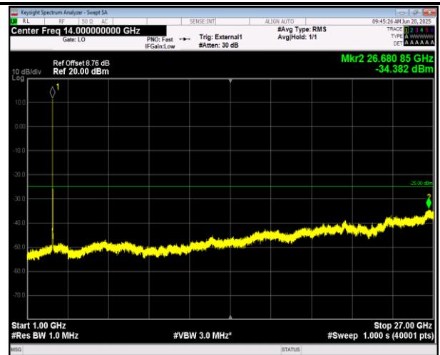
41(2555-2655)-41(2555-2655)-15MHz-10MHz-QPSK-QPS K-40315-40435-1RB#0-ORB#0-1000~27000MHz-PASS
