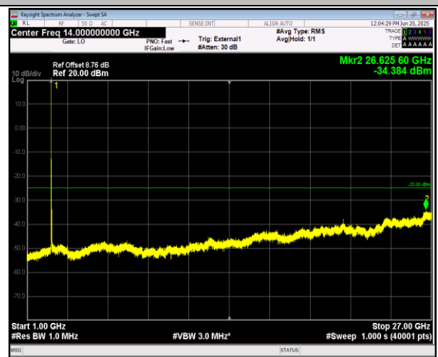
41(2555-2655)-41(2555-2655)-15MHz-10MHz-QPSK-QPS K-40315-40435-1RB#0-1RB#49-1000~27000MHz-PASS
