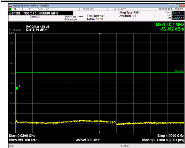
41(2555-2655)-41(2555-2655)-10MHz-20MHz-QPSK-QP SK-40646-40790-50RB#0-100RB#0-30~1000MHz-PASS
