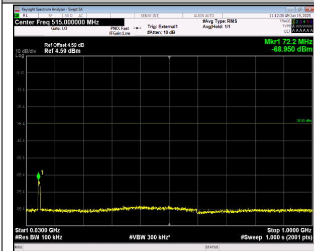
41(2555-2655)-41(2555-2655)-10MHz-15MHz-16QAM-16 QAM-41045-41165-1RB#0-ORB#0-30~1000MHz-PASS
