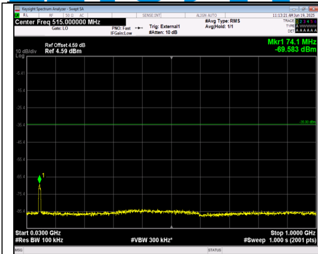
41(2555-2655)-41(2555-2655)-10MHz-20MHz-QPSK-QP SK-40295-40439-1RB#0-ORB#0-30~1000MHz-PASS
