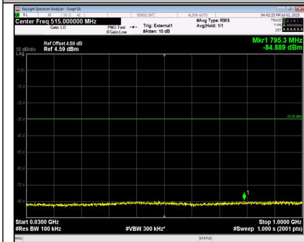
41(2555-2655)-41(2555-2655)-20MHz-5MHz-QPSK-QPS K-40340-40457-1RB#99-ORB#0-30~1000MHz-PASS
