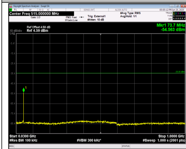
41(2555-2655)-41(2555-2655)-15MHz-20MHz-QPSK-QP SK-40969-41140-75RB#0-100RB#0-30~1000MHz-PASS
