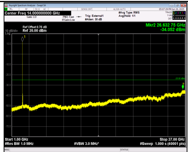
41(2555-2655)-41(2555-2655)-15MHz-20MHz-QPSK-QPS K-40969-41140-1RB#74-ORB#0-1000~27000MHz-PASS
