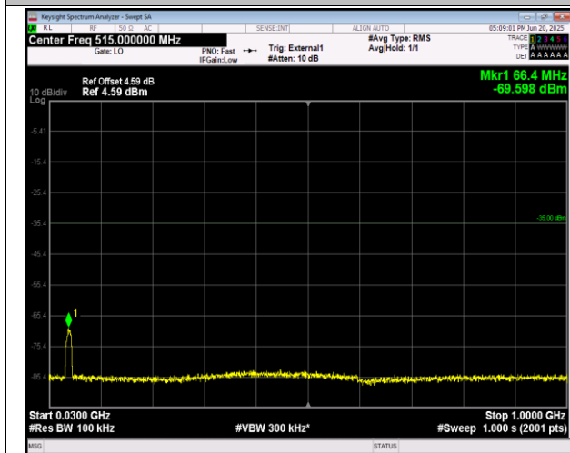
41(2555-2655)-41(2555-2655)-15MHz-20MHz-16QAM-16 QAM-40969-41140-1RB#0-ORB#0-30~1000MHz-PASS
