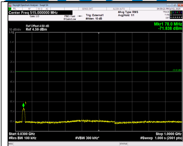
41(2555-2655)-41(2555-2655)-20MHz-20MHz-QPSK-QP SK-40340-40538-1RB#0-ORB#0-30~1000MHz-PASS
