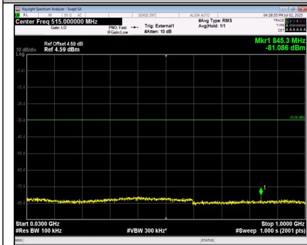
41(2555-2655)-41(2555-2655)-20MHz-5MHz-QPSK-QPS K-40340-40457-1RB#0-1RB#24-30~1000MHz-PASS
