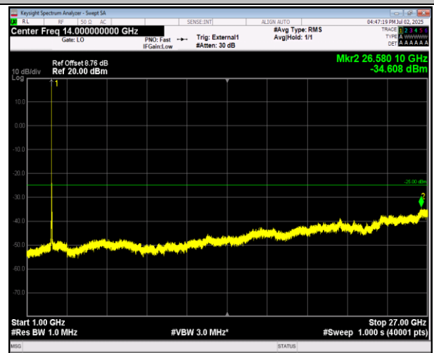
41(2555-2655)-41(2555-2655)-20MHz-5MHz-16QAM-16QA M-40715-40832-1RB#0-1RB#24-1000~27000MHz-PASS
