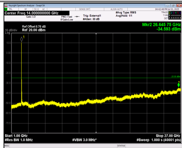
41(2555-2655)-41(2555-2655)-20MHz-5MHz-QPSK-QPSK- 40340-40457-1RB#99-ORB#0-1000~27000MHz-PASS
