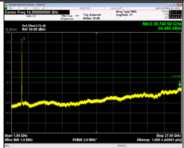
41(2555-2655)-41(2555-2655)-20MHz-5MHz-16QAM-16QA M-40715-40832-1RB#0-0RB#0-1000~27000MHz-PASS
