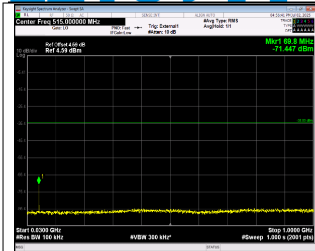
41(2555-2655)-41(2555-2655)-20MHz-5MHz-QPSK-QPS K-41090-41207-1RB#99-0RB#0-30~1000MHz-PASS
