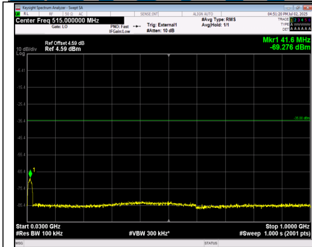
41(2555-2655)-41(2555-2655)-20MHz-5MHz-16QAM-16 QAM-40715-40832-1RB#0-0RB#0-30~1000MHz-PASS
