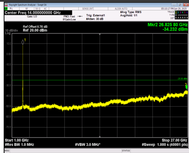
41(2555-2655)-41(2555-2655)-20MHz-5MHz-QPSK-QPSK- 40340-40457-1RB#0-ORB#0-1000~27000MHz-PASS
