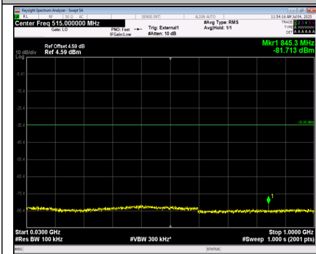
41(2555-2655)-41(2555-2655)-20MHz-20MHz-QPSK-QP SK-40340-40538-1RB#0-1RB#99-30~1000MHz-PASS
