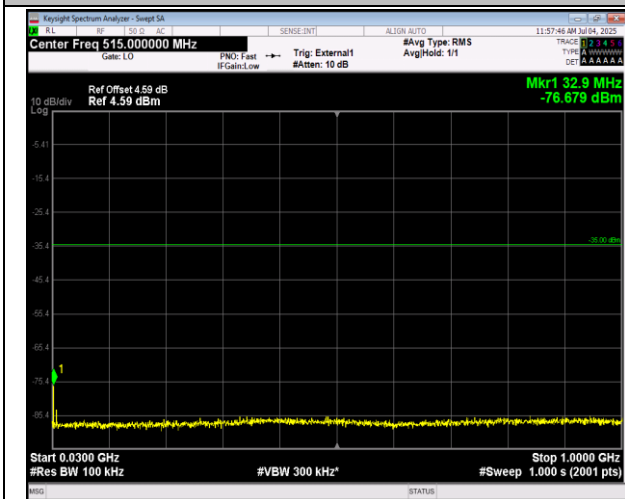
41(2555-2655)-41(2555-2655)-20MHz-20MHz-QPSK-QP SK-40340-40538-1RB#99-ORB#0-30~1000MHz-PASS
