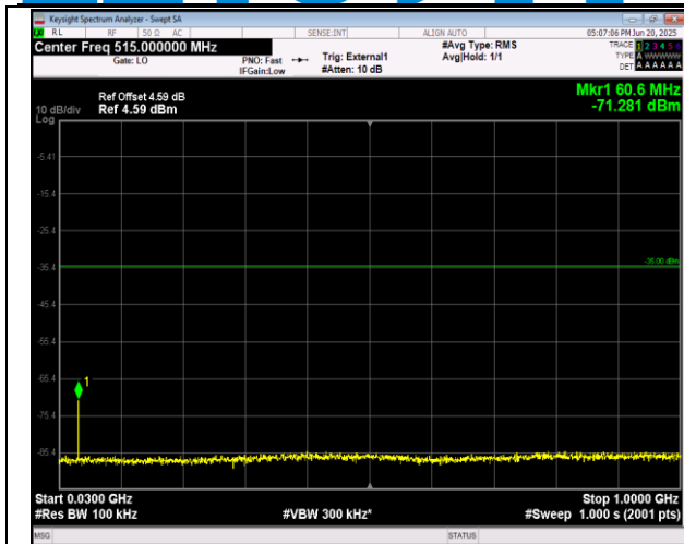
41(2555-2655)-41(2555-2655)-15MHz-20MHz-QPSK-QP SK-40969-41140-1RB#74-ORB#0-30~1000MHz-PASS
