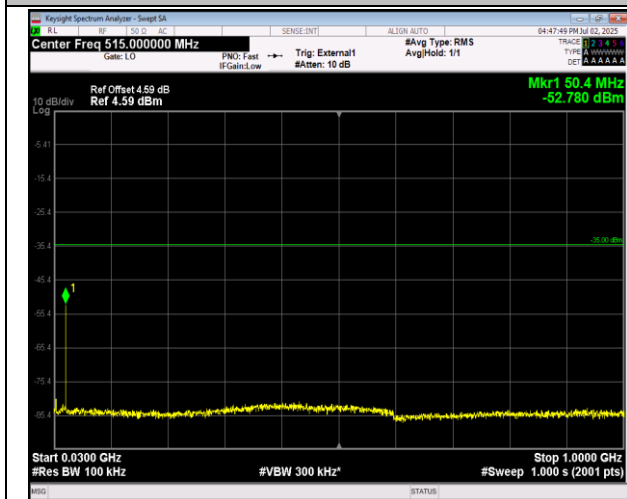
41(2555-2655)-41(2555-2655)-20MHz-5MHz-QPSK-QPS K-40715-40832-100RB#0-25RB#0-30~1000MHz-PASS
