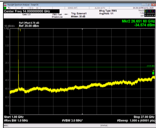
41(2555-2655)-41(2555-2655)-20MHz-5MHz-QPSK-QPSK- 40340-40457-1RB#0-1RB#24-1000~27000MHz-PASS
