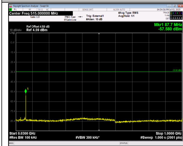
41(2555-2655)-41(2555-2655)-20MHz-5MHz-QPSK-QPS K-41090-41207-100RB#0-25RB#0-30~1000MHz-PASS
