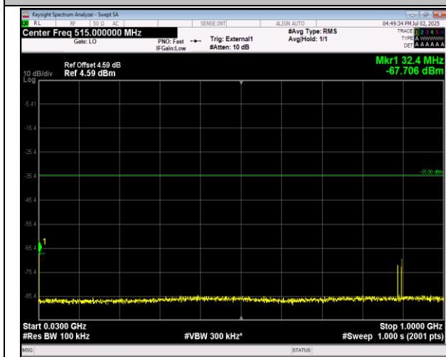
41(2555-2655)-41(2555-2655)-20MHz-5MHz-QPSK-QPS K-40715-40832-1RB#99-0RB#0-30~1000MHz-PASS
