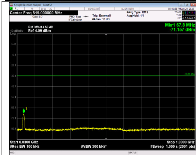
41(2555-2655)-41(2555-2655)-20MHz-5MHz-QPSK-QPS K-40340-40457-1RB#0-ORB#0-30~1000MHz-PASS
