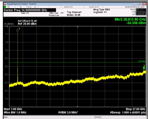
41(2555-2655)-41(2555-2655)-20MHz-5MHz-16QAM-16QA M-40715-40832-1RB#99-0RB#0-1000~27000MHz-PASS
