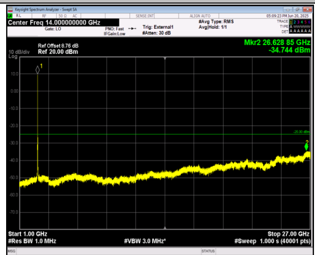
41(2555-2655)-41(2555-2655)-15MHz-20MHz-16QAM-16Q AM-40969-41140-1RB#0-ORB#0-1000~27000MHz-PASS
