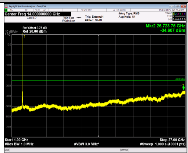
41(2555-2655)-41(2555-2655)-15MHz-20MHz-QPSK-QPS K-40969-41140-75RB#0-100RB#0-1000~27000MHz-PASS
