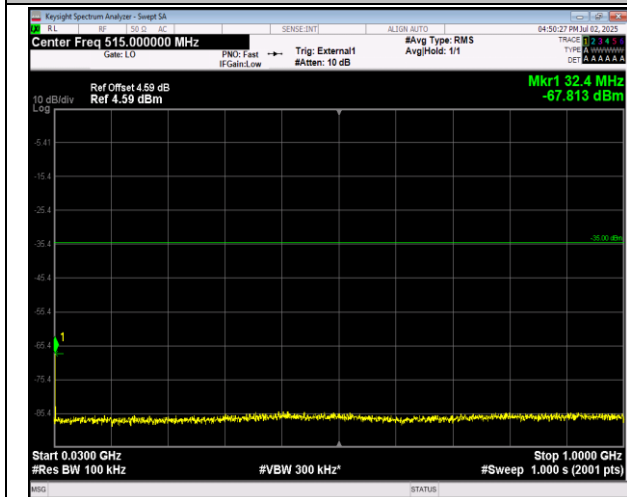
41(2555-2655)-41(2555-2655)-20MHz-5MHz-16QAM-16 QAM-40715-40832-1RB#99-0RB#0-30~1000MHz-PASS
