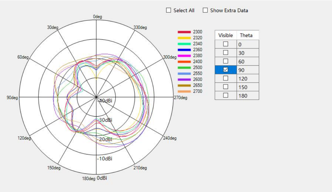
LTE B7/B38/B40/41 Theta=90deg
