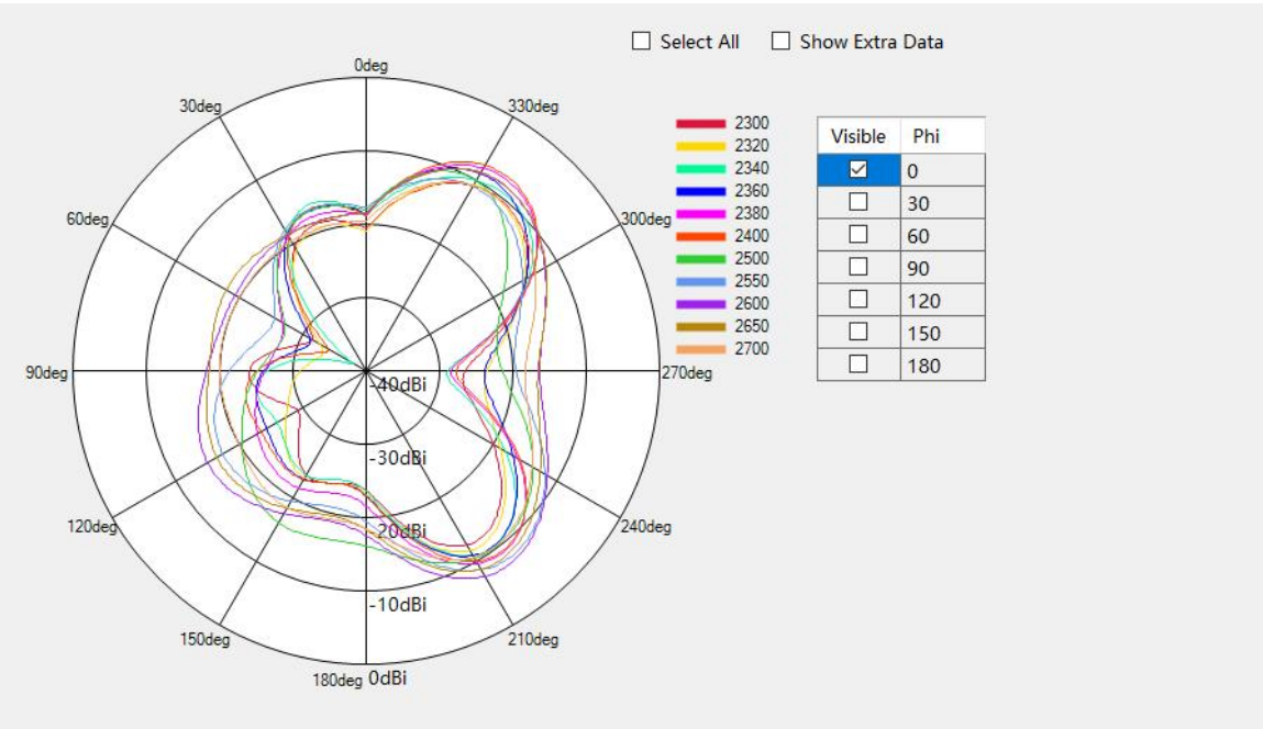
LTE B7/B38/B40/41 Phi=0deg
