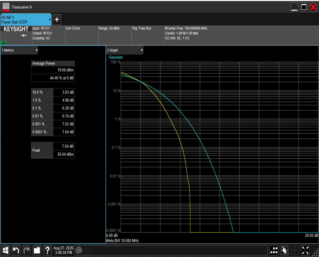
n12 SCS=15kHz DFT_QAM64 BW=10MHz Channel=140800 RB=50@0
