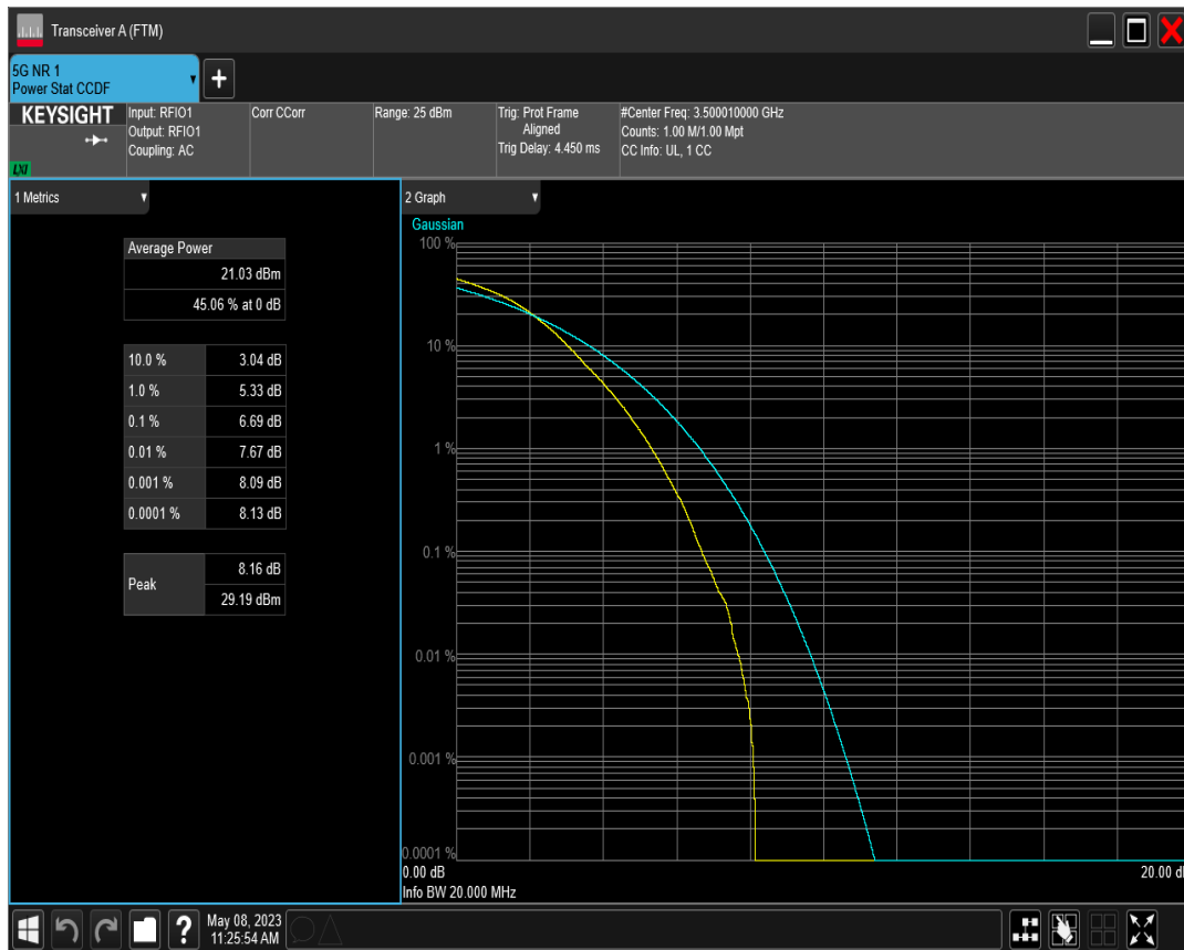
n77(3450-3550) SCS=30kHz DFT_BPSK BW=20MHz Channel=633334 RB=50@0
