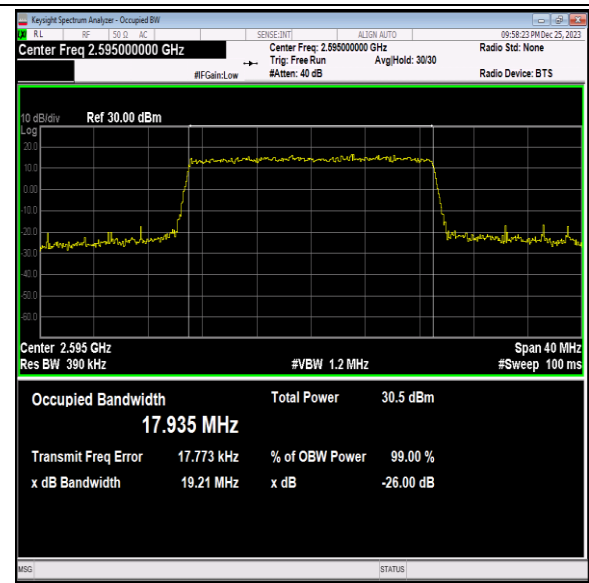
41(2535-2655)-20MHz-16QAM-40640-100RB#0-PASS
