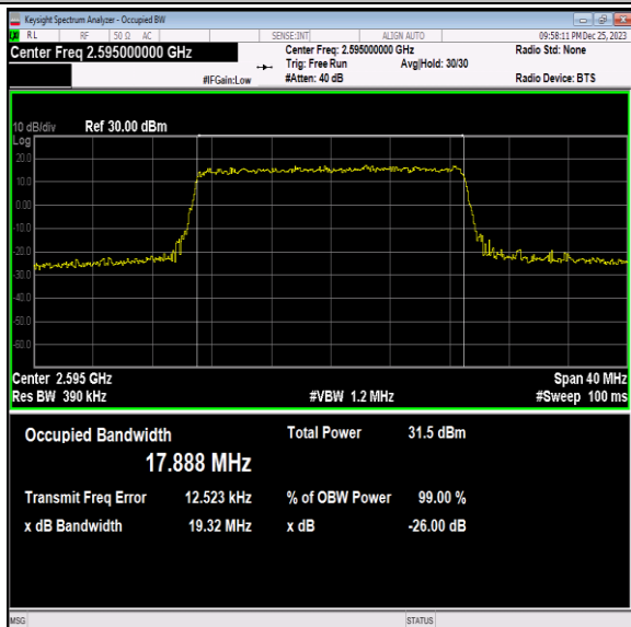
41(2535-2655)-20MHz-QPSK-40640-100RB#0-PASS
