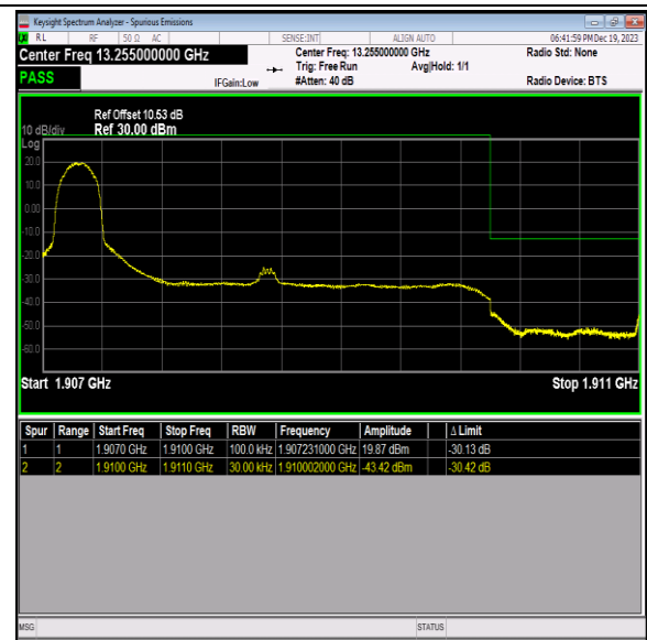
Band2_3MHz_QPSK_19185_1RB#0
