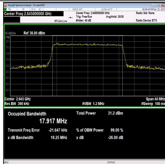
41(2535-2655)-20MHz-QPSK-41140-100RB#0-PASS
