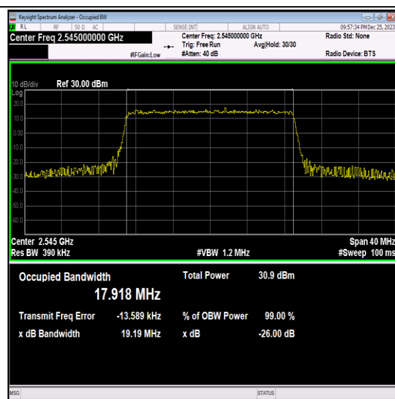
41(2535-2655)-20MHz-QPSK-40140-100RB#0-PASS
