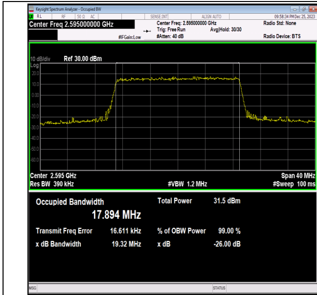
41(2535-2655)-20MHz-64QAM-40640-100RB#0-PASS
