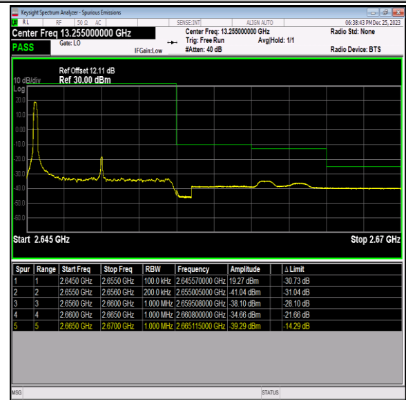
Band41_10MHz_QPSK_41190_1RB#0
