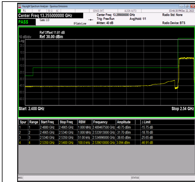
Band41_5MHz_QPSK_40065_25RB#0
