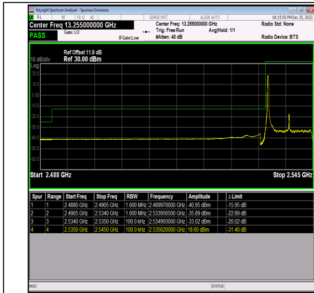
Band41_10MHz_QPSK_40090_1RB#0
