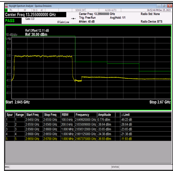
Band41_10MHz_QPSK_41190_50RB#0
