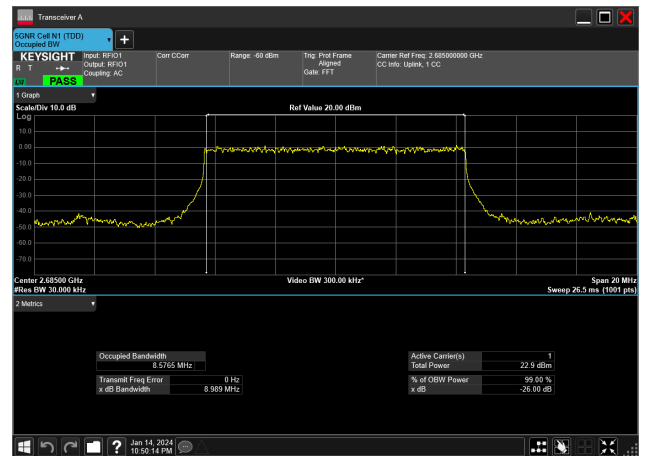
10MHz_30kHz_2685MHz_DFT-s-OFDM PI/2 BPSK_RB24@0&amp;8.576 MHz
