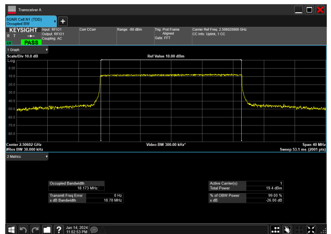
20MHz_30kHz_2506.02MHz_CP-OFDM QPSK_RB51@0&amp;18.173 MHz
