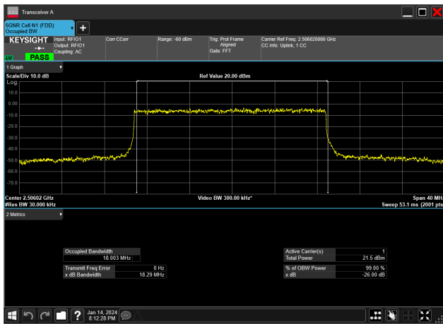
20MHz_30kHz_2506.02MHz_DFT-s-OFDM QPSK_RB50@0&18.003 MHz
