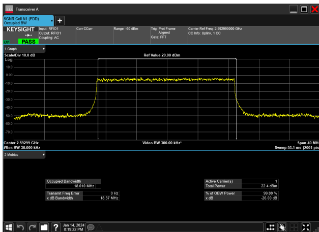
20MHz_30kHz_2592.99MHz_DFT-s-OFDM PI/2 BPSK_RB50@0&amp;18.010 MHz
