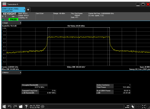
10MHz_30kHz_2685MHz_CP-OFDM 64 QAM_RB24@0&amp;8.571 MHz
