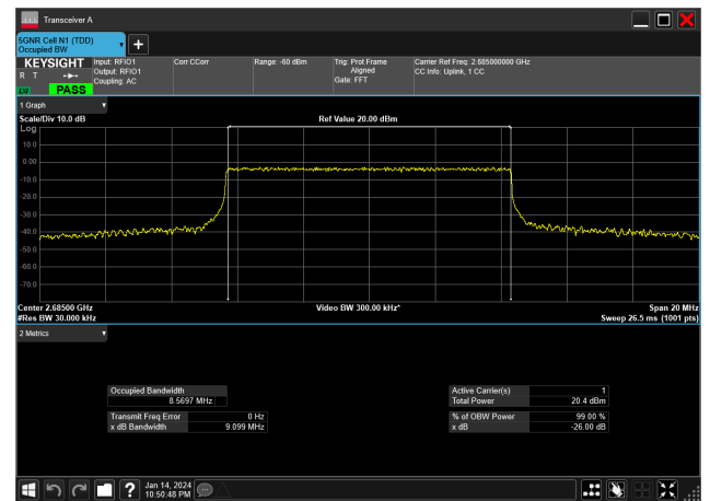
10MHz_30kHz_2685MHz_CP-OFDM QPSK_RB24@0&amp;8.570 MHz
