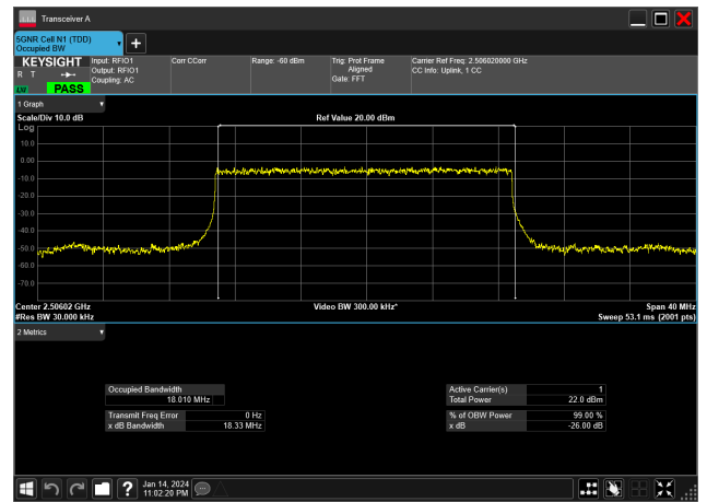
20MHz_30kHz_2506.02MHz_DFT-s-OFDM PI/2 BPSK_RB50@0&18.010 MHz
