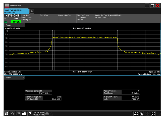
10MHz_30kHz_2685MHz_CP-OFDM 256 QAM_RB24@0&amp;8.568 MHz
