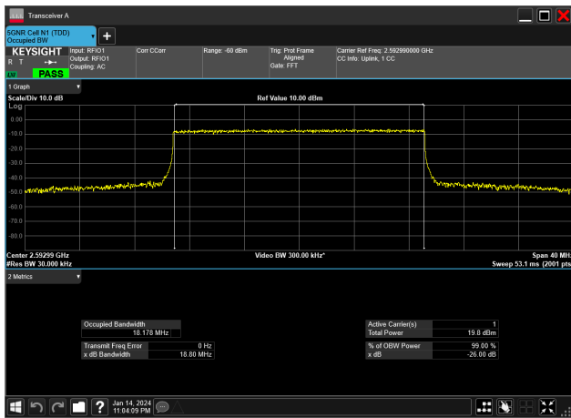
20MHz_30kHz_2592.99MHz_CP-OFDM QPSK_RB51@0&amp;18.178 MHz
