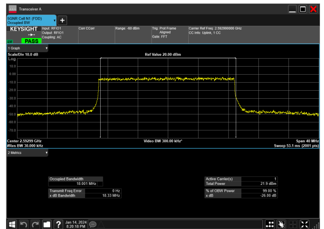
20MHz_30kHz_2592.99MHz_DFT-s-OFDM QPSK_RB50@0&amp;18.001 MHz
