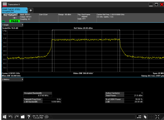
10MHz_30kHz_2501.01MHz_DFT-s-OFDM QPSK_RB24@0&8.575 MHz
