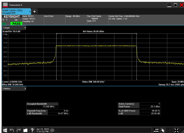
15MHz_30kHz_2682.48MHz_CP-OFDM QPSK_RB38@0&amp;13.568 MHz
