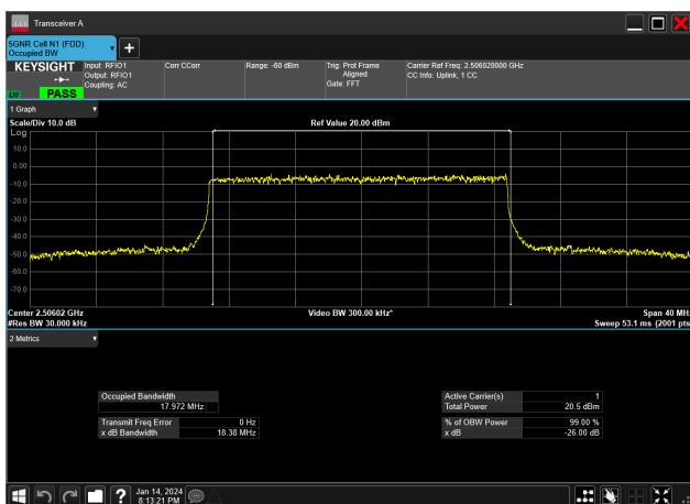
20MHz_30kHz_2506.02MHz_DFT-s-OFDM 16 QAM_RB50@0&amp;17.972 MHz
