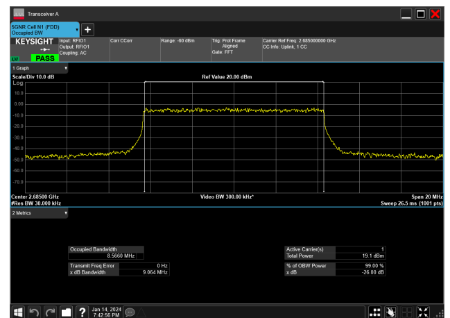
10MHz_30kHz_2685MHz_DFT-s-OFDM 256 QAM_RB24@0&amp;8.566 MHz
