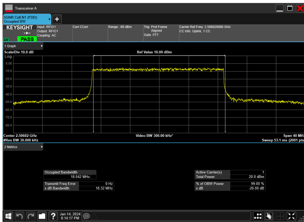
20MHz_30kHz_2506.02MHz_DFT-s-OFDM 64 QAM_RB50@0&18.042 MHz
