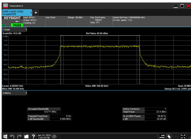
10MHz_30kHz_2685MHz_DFT-s-OFDM QPSK_RB24@0&amp;8.577 MHz
