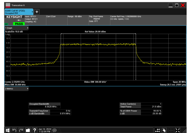
10MHz_30kHz_2592.99MHz_DFT-s-OFDM QPSK_RB24@0&amp;8.563 MHz
