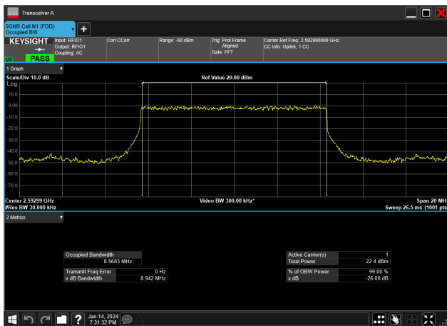
10MHz_30kHz_2592.99MHz_DFT-s-OFDM PI/2 BPSK_RB24@0&amp;8.568 MHz
