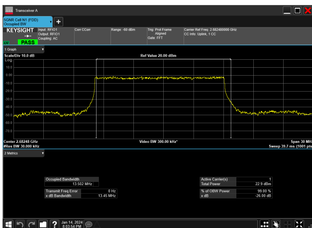
15MHz_30kHz_2682.48MHz_DFT-s-OFDM PI/2 BPSK_RB36@0&amp;13.502 MHz
