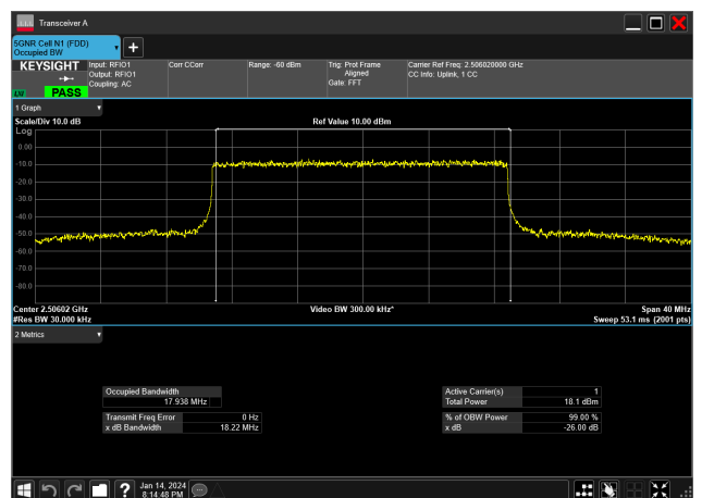
20MHz_30kHz_2506.02MHz_DFT-s-OFDM 256 QAM_RB50@0&amp;17.938 MHz
