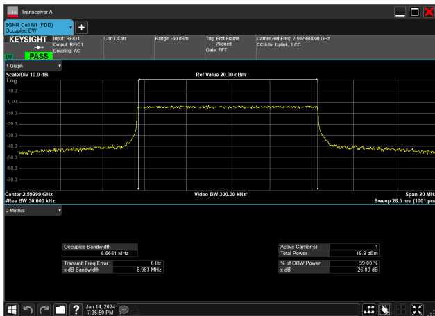
10MHz_30kHz_2592.99MHz_CP-OFDM QPSK_RB24@0&amp;8.568 MHz
