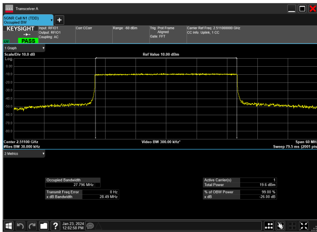
30MHz_30kHz_2511MHz_CP-OFDM QPSK_RB78@0&amp;27.796 MHz
