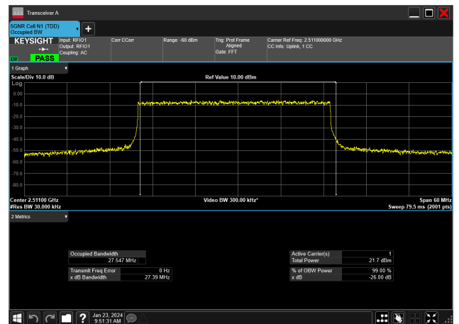
30MHz_30kHz_2511MHz_DFT-s-OFDM QPSK_RB75@0&amp;27.547 MHz
