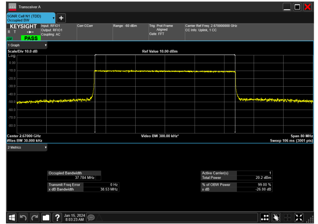
40MHz_30kHz_2670MHz_CP-OFDM QPSK_RB106@0&amp;37.784 MHz
