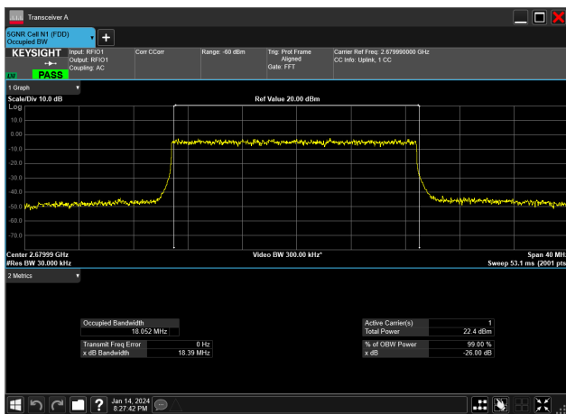
20MHz_30kHz_2679.99MHz_DFT-s-OFDM QPSK_RB50@0&18.052 MHz
