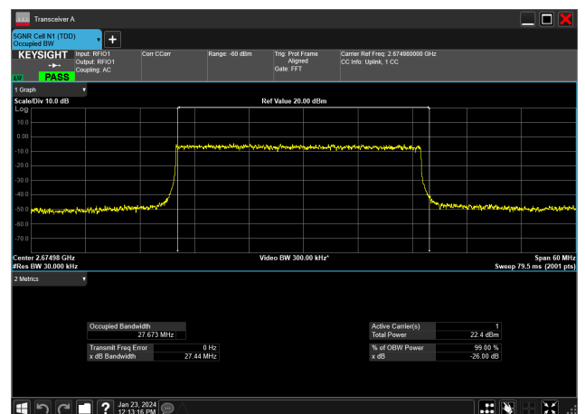
30MHz_30kHz_2674.98MHz_DFT-s-OFDM QPSK_RB75@0&amp;27.673 MHz
