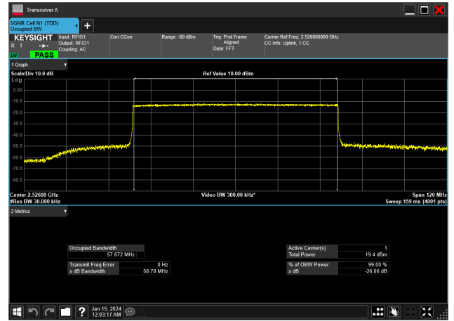
60MHz_30kHz_2526MHz_CP-OFDM QPSK_RB162@0&amp;57.672 MHz
