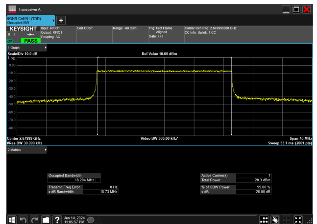
20MHz_30kHz_2679.99MHz_CP-OFDM QPSK_RB51@0&amp;18.204 MHz
