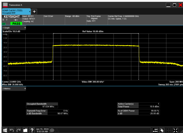
100MHz_30kHz_2640MHz_CP-OFDM QPSK_RB273@0&amp;97.034 MHz
