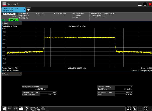
80MHz_30kHz_2649.99MHz_CP-OFDM QPSK_RB217@0&amp;77.299 MHz
