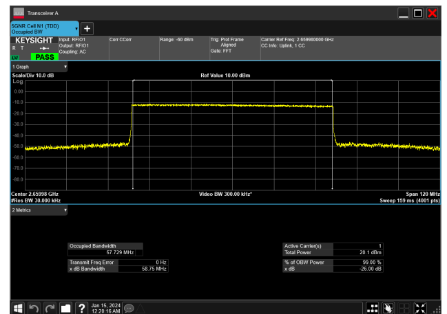
60MHz_30kHz_2659.98MHz_CP-OFDM QPSK_RB162@0&amp;57.729 MHz
