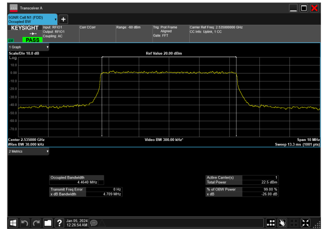
5MHz_15kHz_2535MHz_DFT-s-OFDM QPSK_RB25@0&amp;4.464 MHz
