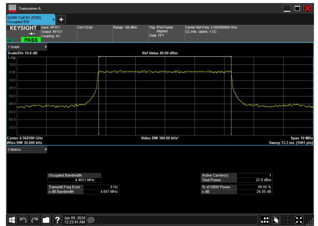
5MHz_15kHz_2502.5MHz_DFT-s-OFDM PI/2 BPSK_RB25@0&amp;4.465 MHz
