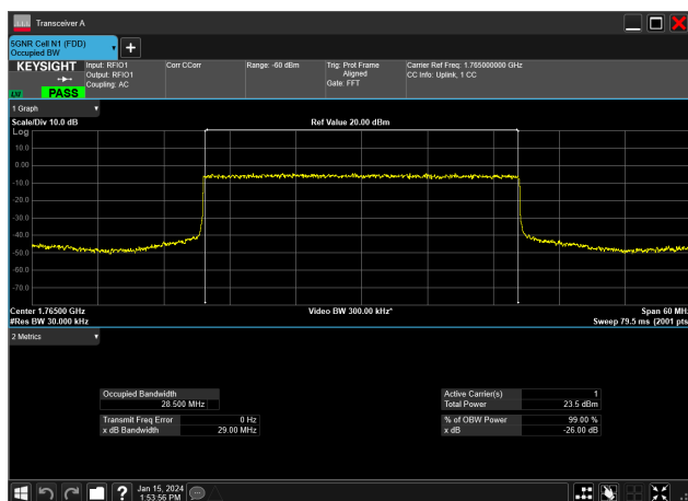
30MHz_15kHz_1765MHz_DFT-s-OFDM PI/2 BPSK_RB160@0&amp;28.500 MHz
