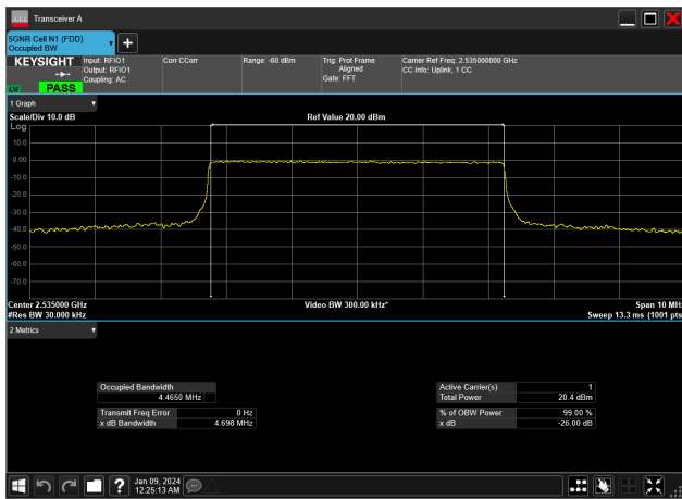
5MHz_15kHz_2535MHz_CP-OFDM QPSK_RB25@0&amp;4.465 MHz
