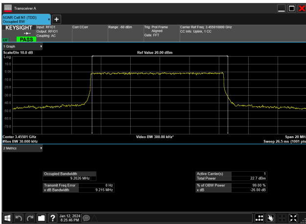
10MHz_15kHz_3455MHz_DFT-s-OFDM QPSK_RB50@0&amp;9.203 MHz
