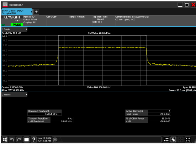
10MHz_15kHz_2565MHz_CP-OFDM QPSK_RB52@0&amp;9.285 MHz
