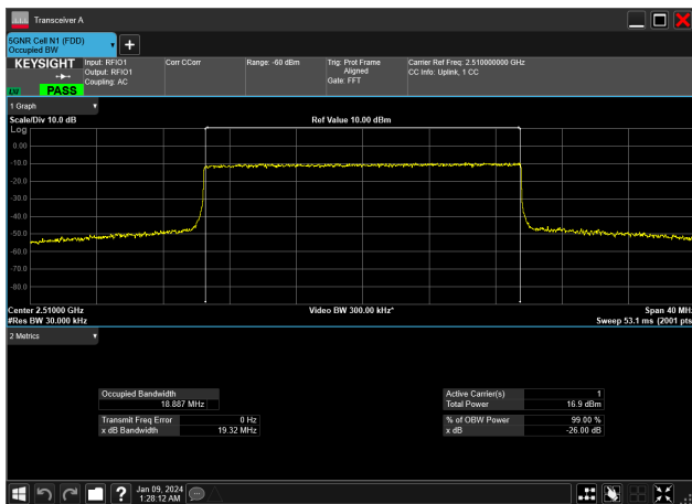
20MHz_15kHz_2510MHz_CP-OFDM 256 QAM_RB106@0&18.887 MHz
