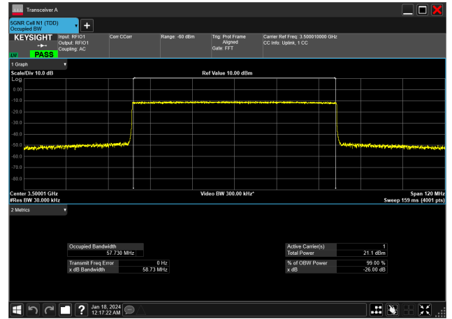
60MHz_30kHz_3500MHz_CP-OFDM QPSK_RB162@0&amp;57.730 MHz
