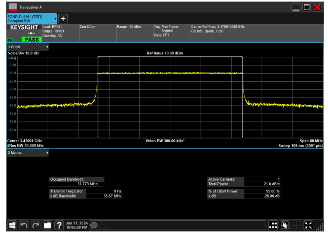
40MHz_30kHz_3470MHz_CP-OFDM QPSK_RB106@0&amp;37.779 MHz
