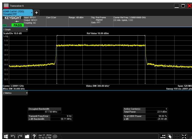
60MHz_30kHz_3500MHz_DFT-s-OFDM QPSK_RB162@0&amp;57.738 MHz
