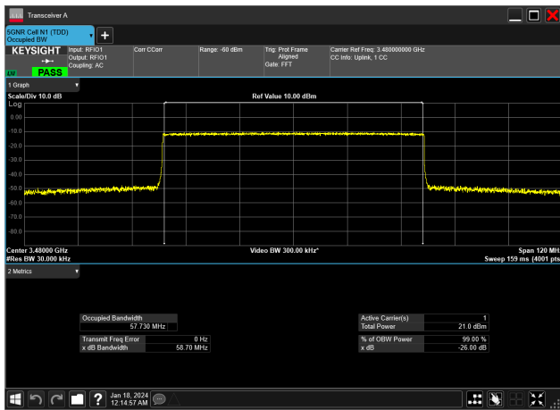
60MHz_30kHz_3480MHz_CP-OFDM QPSK_RB162@0&amp;57.730 MHz
