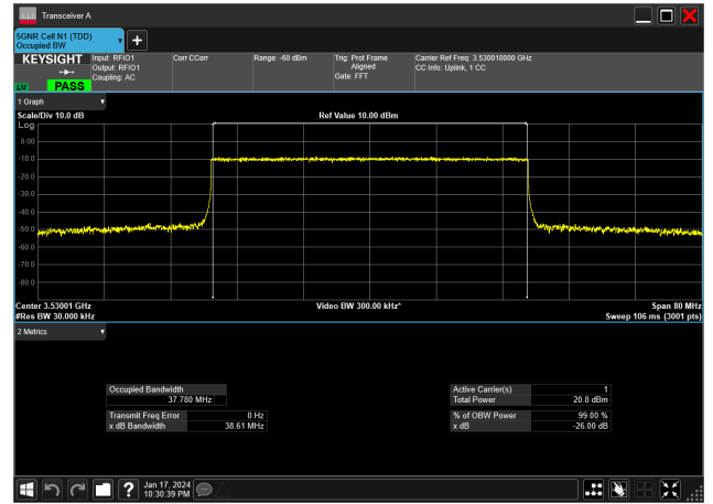
40MHz_30kHz_3530MHz_CP-OFDM QPSK_RB106@0&amp;37.780 MHz
