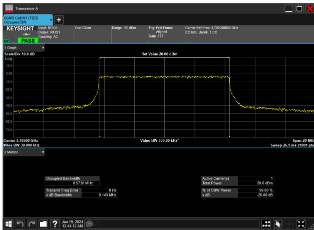
10MHz_30kHz_3705MHz_CP-OFDM QPSK_RB24@0&amp;8.573 MHz
