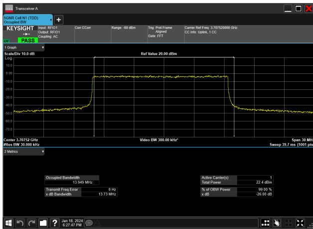
15MHz_15kHz_3707.5MHz_DFT-s-OFDM QPSK_RB75@0&13.949 MHz
