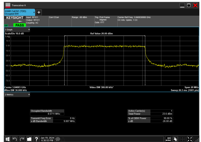
10MHz_30kHz_3840MHz_DFT-s-OFDM PI/2 BPSK_RB24@0&amp;8.571 MHz
