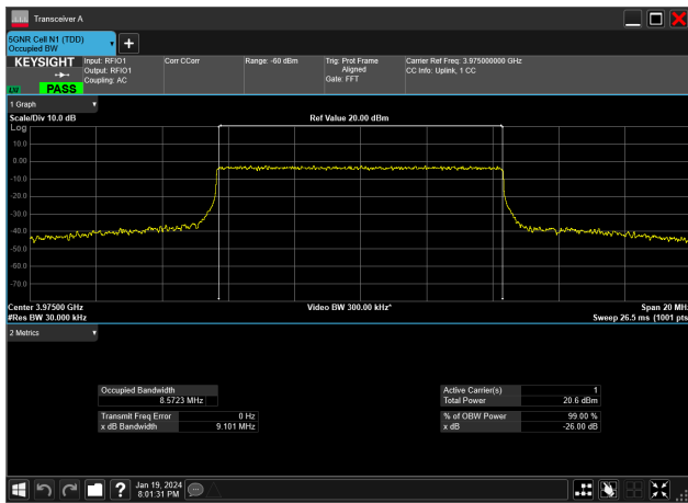
10MHz_30kHz_3975MHz_CP-OFDM QPSK_RB24@0&amp;8.572 MHz
