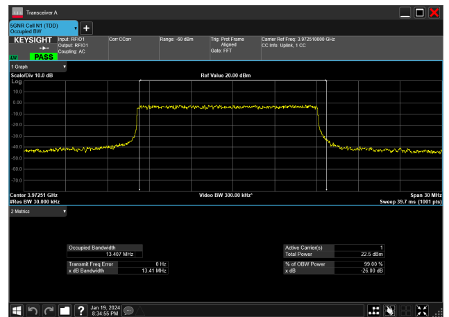
15MHz_30kHz_3972.5MHz_DFT-s-OFDM QPSK_RB36@0&amp;13.407 MHz
