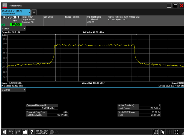
10MHz_15kHz_3705MHz_DFT-s-OFDM QPSK_RB50@0&amp;9.209 MHz
