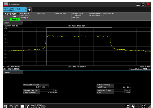
10MHz_15kHz_3840MHz_DFT-s-OFDM QPSK_RB50@0&amp;9.211 MHz
