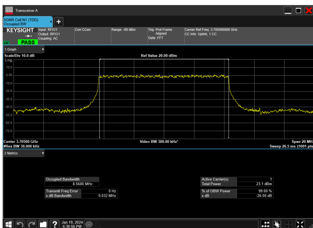
10MHz_30kHz_3705MHz_DFT-s-OFDM PI/2 BPSK_RB24@0&amp;8.568 MHz
