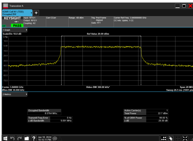
10MHz_30kHz_3840MHz_DFT-s-OFDM QPSK_RB24@0&amp;8.576 MHz
