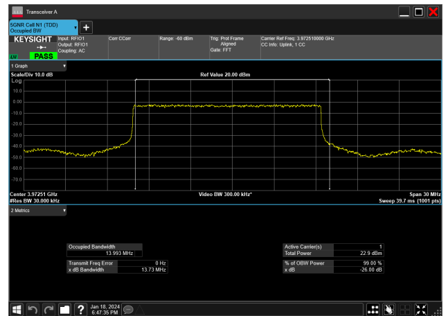
15MHz_15kHz_3972.5MHz_DFT-s-OFDM PI/2 BPSK_RB75@0&13.993 MHz
