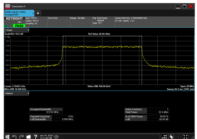
10MHz_30kHz_3705MHz_DFT-s-OFDM QPSK_RB24@0&amp;8.575 MHz
