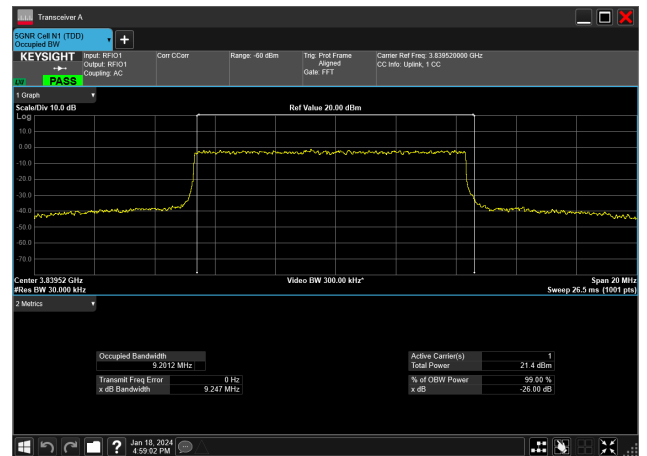
10MHz_15kHz_3840MHz_DFT-s-OFDM 16 QAM_RB50@0&amp;9.201 MHz
