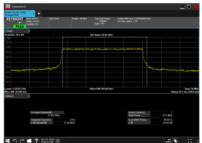
15MHz_30kHz_3707.5MHz_DFT-s-OFDM QPSK_RB36@0&amp;13.402 MHz
