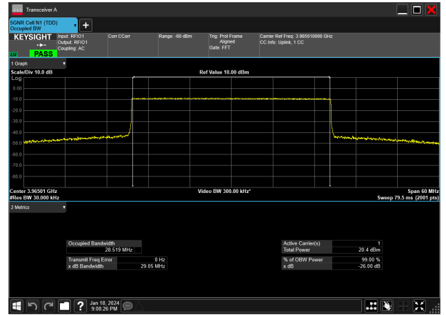
30MHz_15kHz_3965MHz_CP-OFDM QPSK_RB160@0&amp;28.519 MHz
