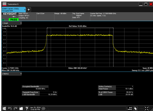
20MHz_30kHz_3710MHz_DFT-s-OFDM 256 QAM_RB50@0&amp;18.009 MHz
