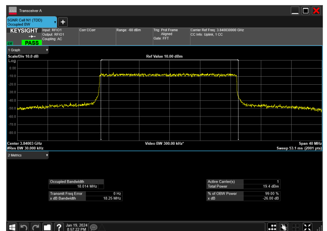
20MHz_30kHz_3840MHz_DFT-s-OFDM 256 QAM_RB50@0&amp;18.014 MHz
