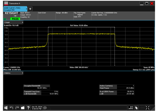
20MHz_30kHz_3840MHz_CP-OFDM QPSK_RB51@0&amp;18.201 MHz
