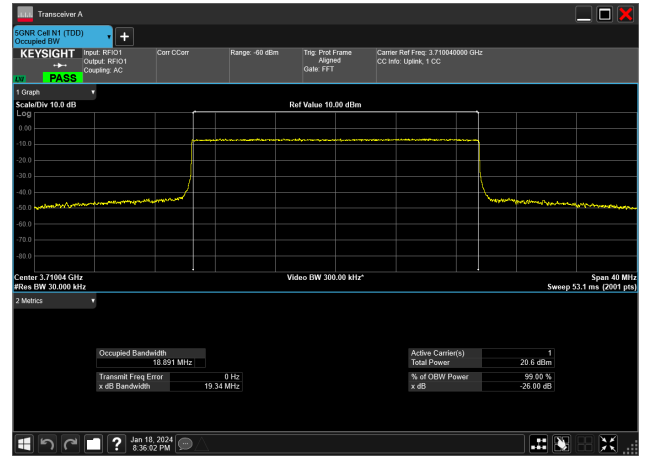
20MHz_15kHz_3710MHz_CP-OFDM QPSK_RB106@0&amp;18.891 MHz
