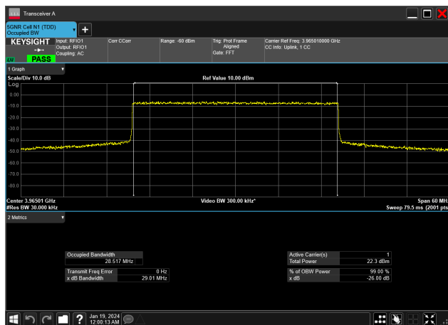
30MHz_15kHz_3965MHz_DFT-s-OFDM QPSK_RB160@0&amp;28.517 MHz
