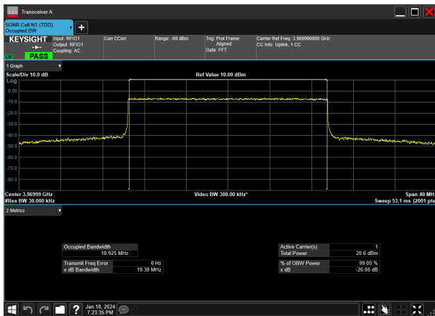
20MHz_15kHz_3970MHz_CP-OFDM 16 QAM_RB106@0&amp;18.925 MHz
