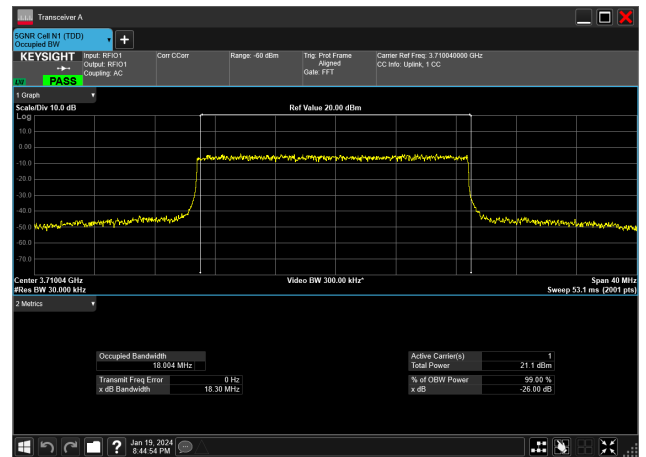
20MHz_30kHz_3710MHz_DFT-s-OFDM 64 QAM_RB50@0&amp;18.004 MHz
