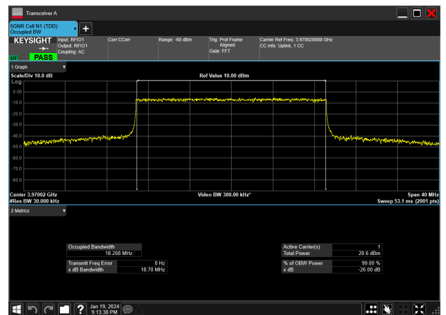
20MHz_30kHz_3970MHz_CP-OFDM 16 QAM_RB51@0&amp;18.208 MHz
