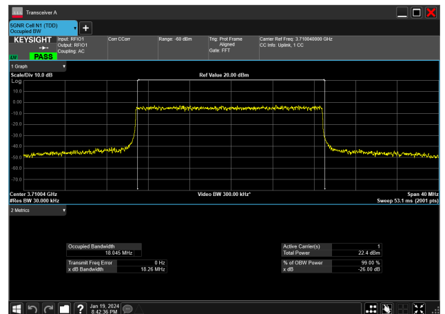
20MHz_30kHz_3710MHz_DFT-s-OFDM QPSK_RB50@0&amp;18.045 MHz
