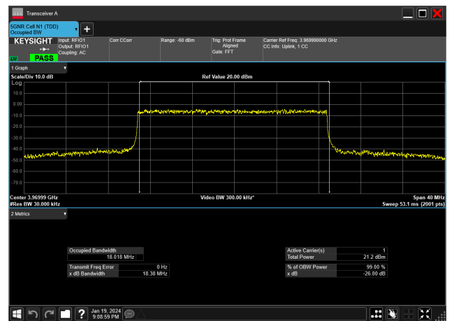
20MHz_30kHz_3970MHz_DFT-s-OFDM 64 QAM_RB50@0&amp;18.018 MHz
