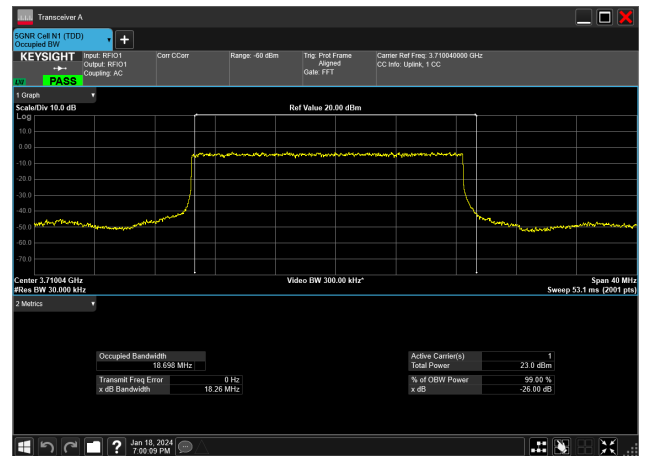
20MHz_15kHz_3710MHz_DFT-s-OFDM PI/2 BPSK_RB100@0&amp;18.698 MHz
