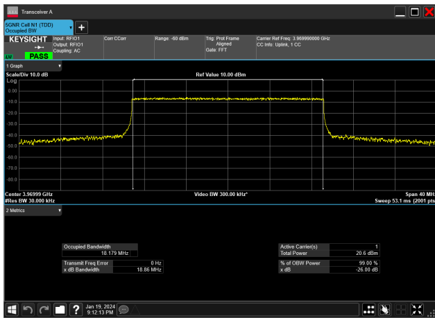
20MHz_30kHz_3970MHz_CP-OFDM QPSK_RB51@0&amp;18.179 MHz
