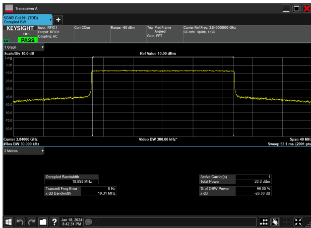
20MHz_15kHz_3840MHz_CP-OFDM QPSK_RB106@0&amp;18.893 MHz
