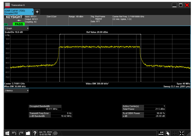
20MHz_30kHz_3710MHz_DFT-s-OFDM 16 QAM_RB50@0&amp;18.011 MHz
