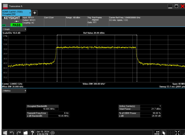
20MHz_30kHz_3840MHz_DFT-s-OFDM 16 QAM_RB50@0&amp;18.005 MHz
