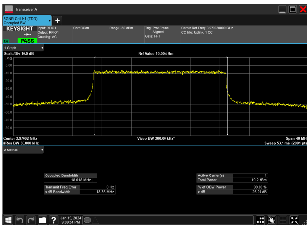
20MHz_30kHz_3970MHz_DFT-s-OFDM 256 QAM_RB50@0&amp;18.018 MHz
