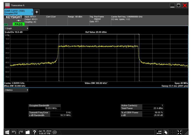
20MHz_30kHz_3970MHz_DFT-s-OFDM QPSK_RB50@0&amp;18.053 MHz
