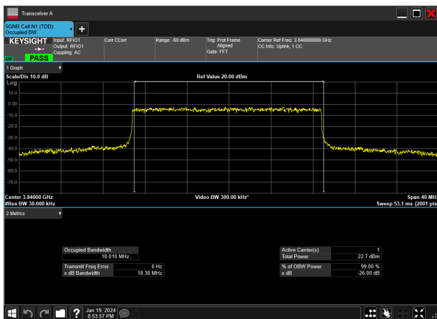
20MHz_30kHz_3840MHz_DFT-s-OFDM QPSK_RB50@0&amp;18.010 MHz
