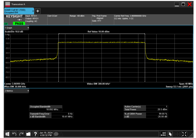
20MHz_15kHz_3970MHz_CP-OFDM QPSK_RB106@0&amp;18.892 MHz
