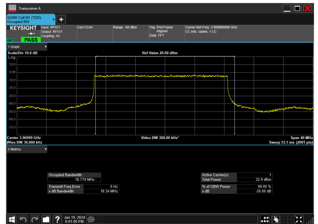
20MHz_15kHz_3970MHz_DFT-s-OFDM PI/2 BPSK_RB100@0&amp;18.779 MHz
