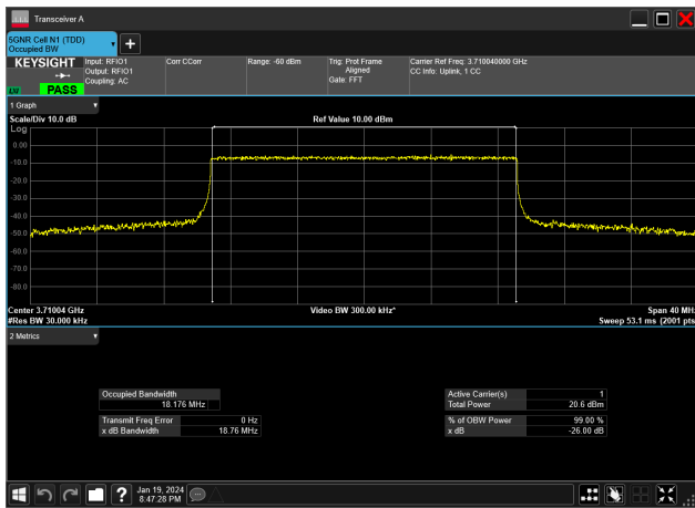
20MHz_30kHz_3710MHz_CP-OFDM QPSK_RB51@0&amp;18.176 MHz
