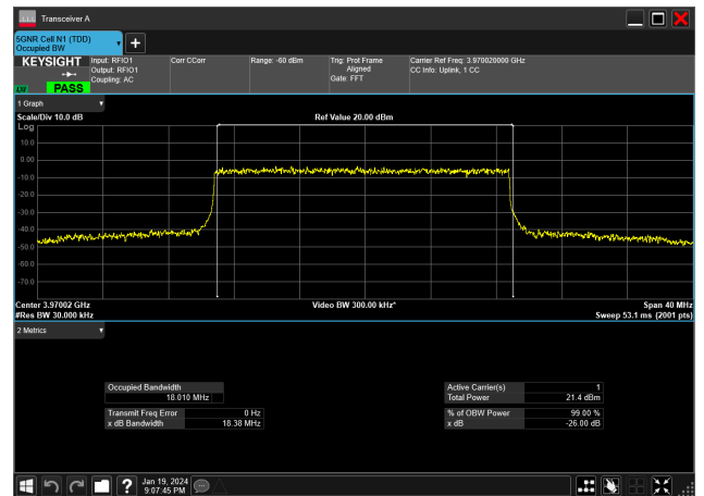
20MHz_30kHz_3970MHz_DFT-s-OFDM 16 QAM_RB50@0&amp;18.010 MHz
