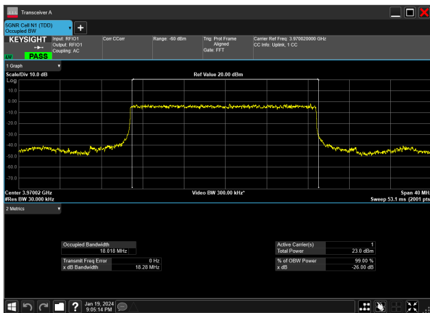
20MHz_30kHz_3970MHz_DFT-s-OFDM PI/2 BPSK_RB50@0&amp;18.018 MHz
