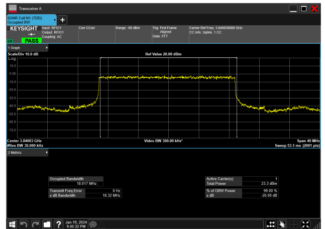
20MHz_30kHz_3840MHz_DFT-s-OFDM PI/2 BPSK_RB50@0&amp;18.017 MHz
