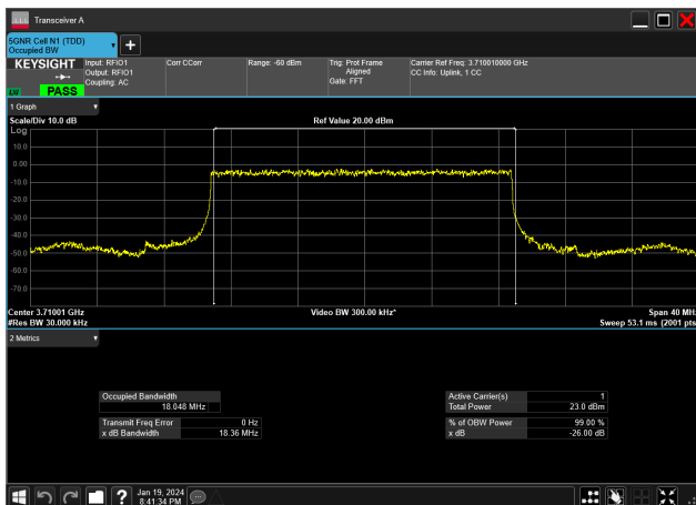
20MHz_30kHz_3710MHz_DFT-s-OFDM PI/2 BPSK_RB50@0&amp;18.048 MHz
