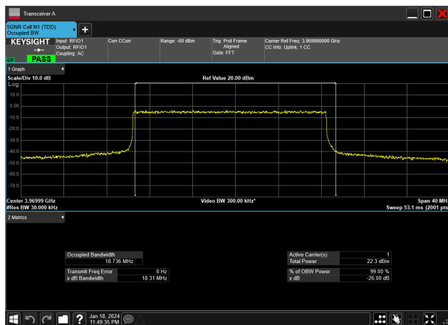
20MHz_15kHz_3970MHz_DFT-s-OFDM QPSK_RB100@0&amp;18.736 MHz
