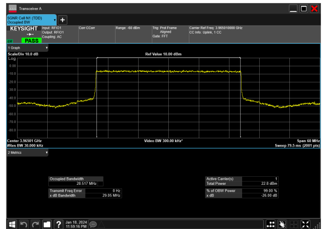
30MHz_15kHz_3965MHz_DFT-s-OFDM PI/2 BPSK_RB160@0&amp;28.517 MHz
