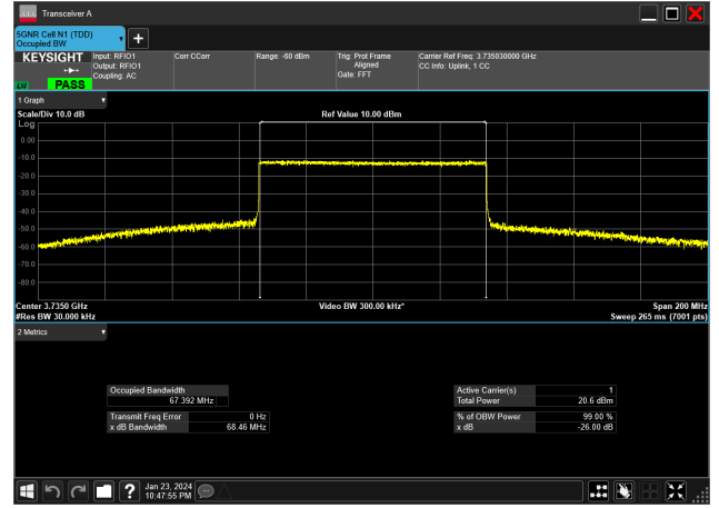
70MHz_30kHz_3735MHz_CP-OFDM QPSK_RB189@0&amp;67.392 MHz
