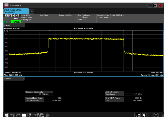
60MHz_30kHz_3950MHz_DFT-s-OFDM QPSK_RB162@0&amp;57.731 MHz
