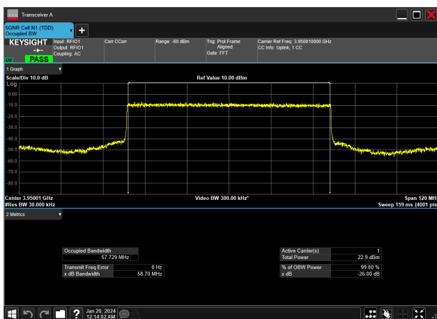
60MHz_30kHz_3950MHz_DFT-s-OFDM PI/2 BPSK_RB162@0&amp;57.729 MHz
