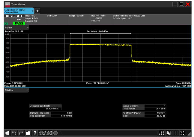
70MHz_30kHz_3945MHz_CP-OFDM QPSK_RB189@0&amp;67.429 MHz
