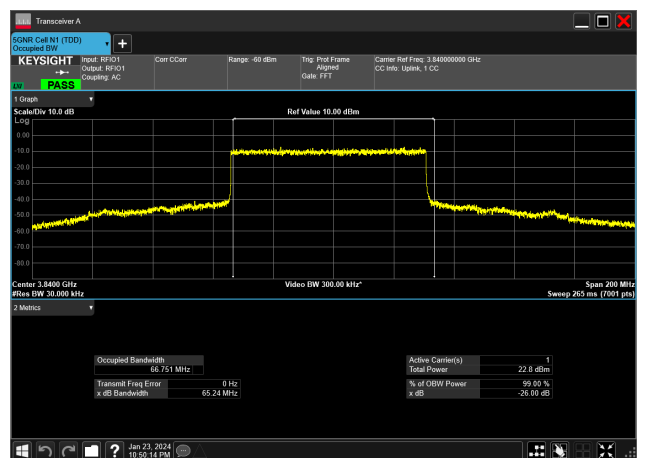
70MHz_30kHz_3840MHz_DFT-s-OFDM QPSK_RB180@0&amp;66.751 MHz
