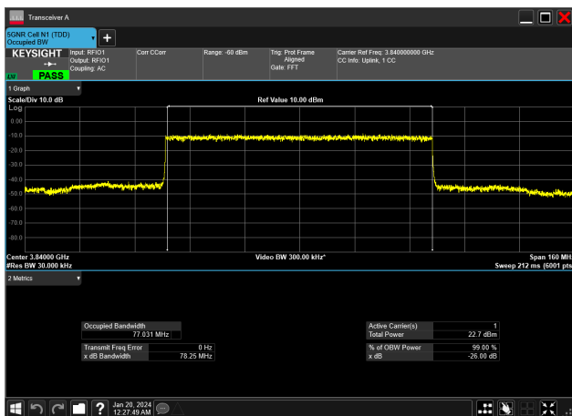
80MHz_30kHz_3840MHz_DFT-s-OFDM QPSK_RB216@0&amp;77.031 MHz
