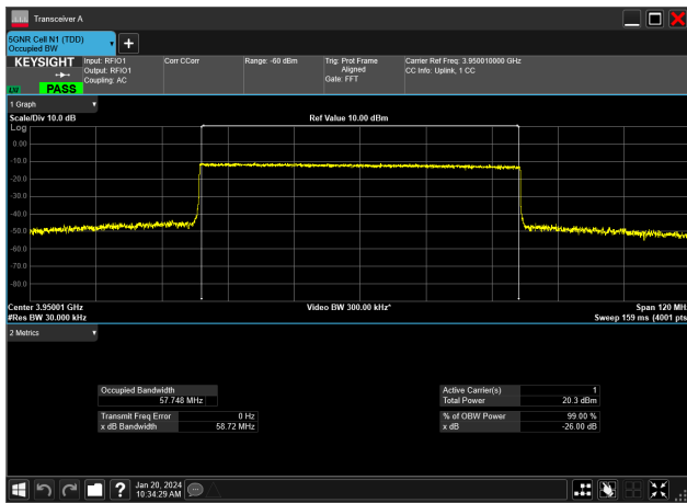
60MHz_30kHz_3950MHz_CP-OFDM QPSK_RB162@0&amp;57.748 MHz
