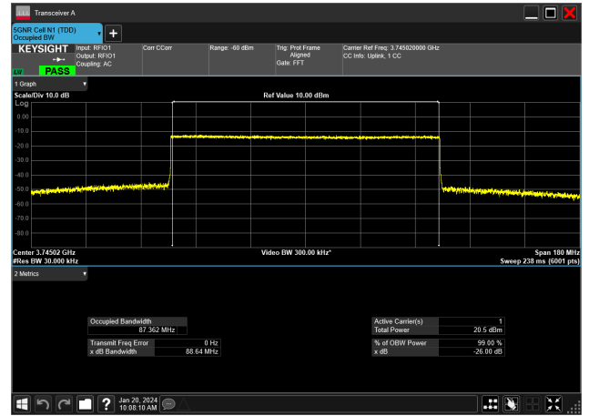
90MHz_30kHz_3745MHz_CP-OFDM QPSK_RB245@0&amp;87.362 MHz
