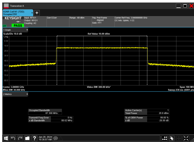
90MHz_30kHz_3840MHz_CP-OFDM QPSK_RB245@0&amp;87.308 MHz
