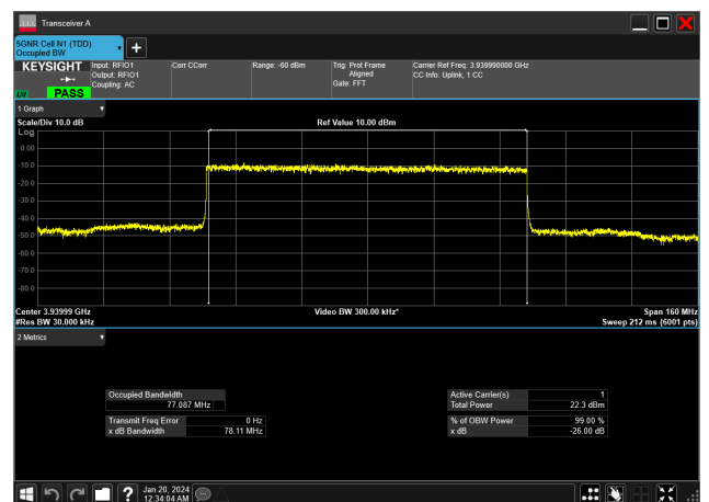
80MHz_30kHz_3940MHz_DFT-s-OFDM QPSK_RB216@0&amp;77.087 MHz
