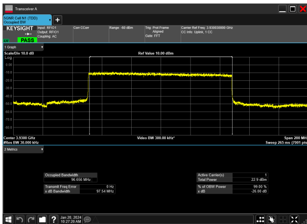
100MHz_30kHz_3930MHz_DFT-s-OFDM PI/2 BPSK_RB270@0&96.656 MHz
