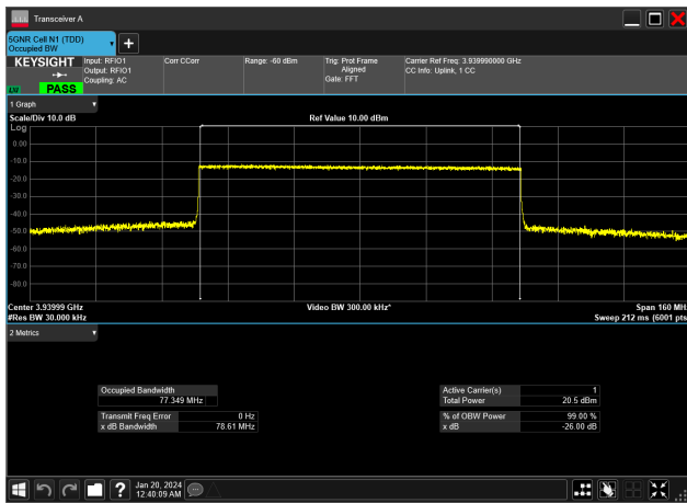
80MHz_30kHz_3940MHz_CP-OFDM QPSK_RB217@0&amp;77.349 MHz
