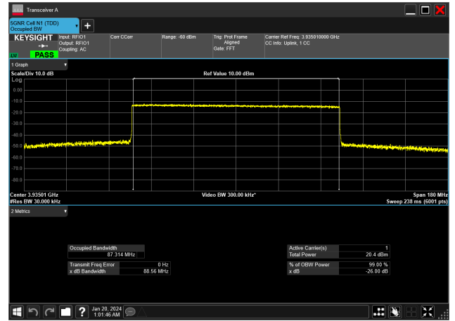
90MHz_30kHz_3935MHz_CP-OFDM QPSK_RB245@0&amp;87.314 MHz
