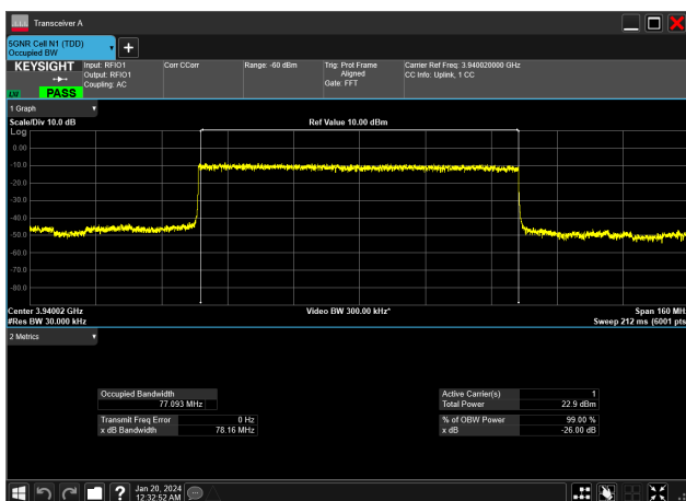
80MHz_30kHz_3940MHz_DFT-s-OFDM PI/2 BPSK_RB216@0&amp;77.093 MHz
