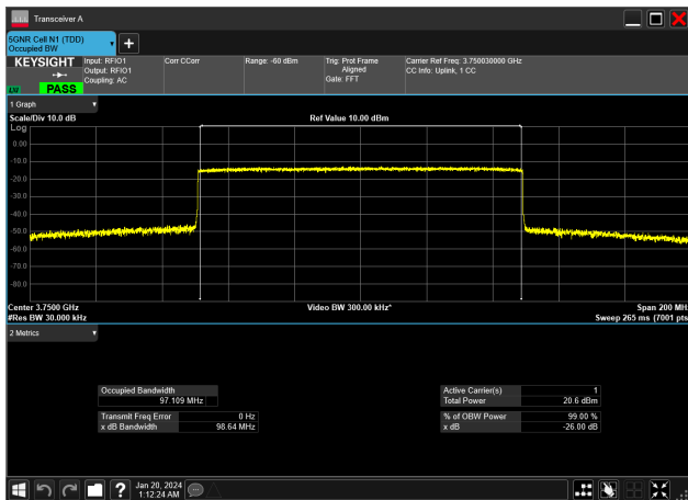
100MHz_30kHz_3750MHz_CP-OFDM QPSK_RB273@0&97.109 MHz
