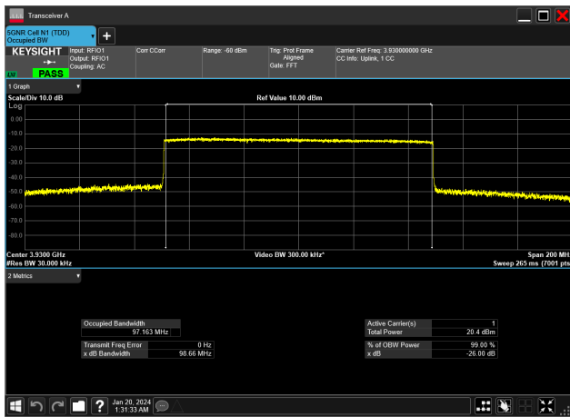
100MHz_30kHz_3930MHz_CP-OFDM QPSK_RB273@0&97.163 MHz
