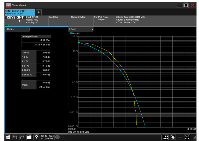
10MHz_15kHz_836.5MHz_DFT-s-OFDM 16 QAM_RB50@0&amp;8.70 dB
