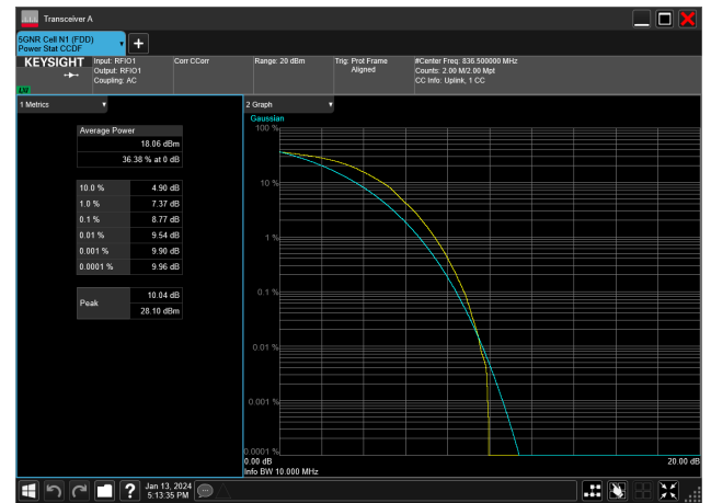
10MHz_15kHz_836.5MHz_DFT-s-OFDM 64 QAM_RB50@0&amp;8.77 dB
