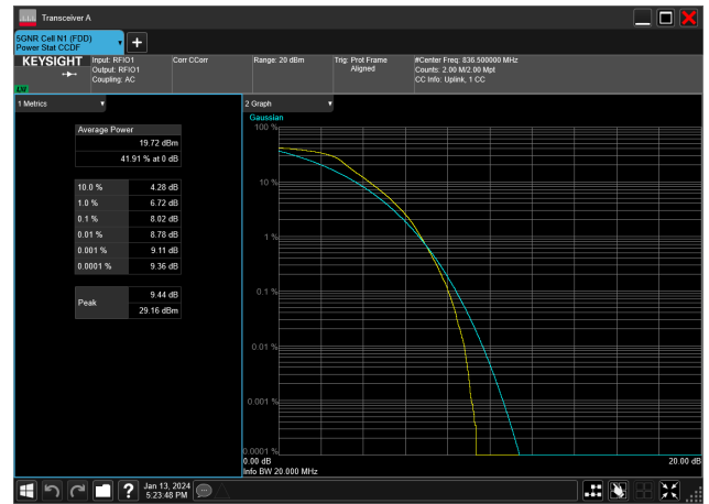
20MHz_15kHz_836.5MHz_DFT-s-OFDM QPSK_RB100@0&amp;8.02 dB
