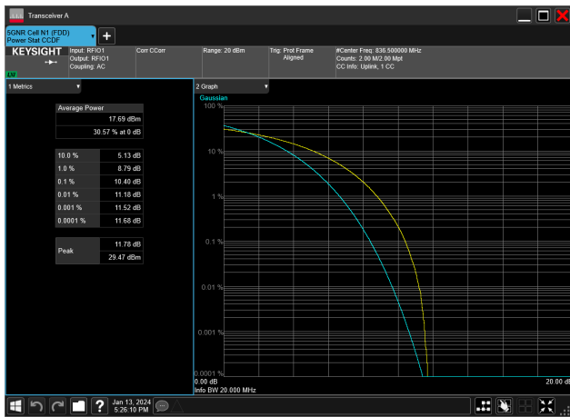
20MHz_15kHz_836.5MHz_CP-OFDM QPSK_RB106@0&amp;10.40 dB
