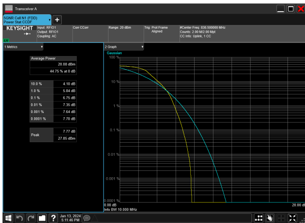
10MHz_15kHz_836.5MHz_DFT-s-OFDM PI/2 BPSK_RB50@0&amp;6.75 dB
