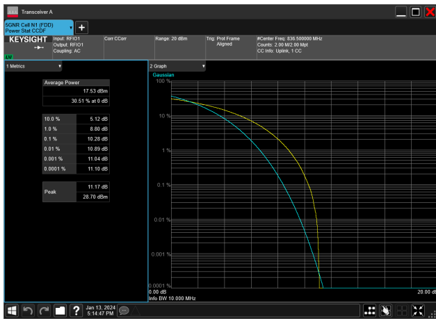
10MHz_15kHz_836.5MHz_CP-OFDM QPSK_RB52@0&amp;10.28 dB
