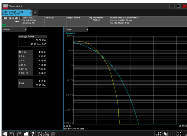
20MHz_15kHz_836.5MHz_DFT-s-OFDM PI/2 BPSK_RB100@0&amp;6.82 dB
