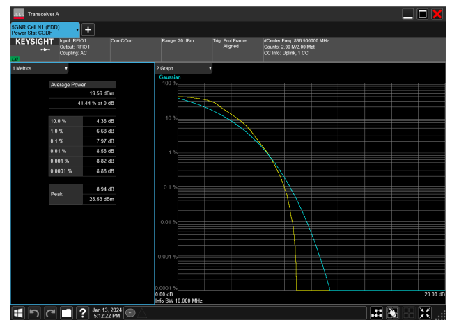
10MHz_15kHz_836.5MHz_DFT-s-OFDM QPSK_RB50@0&amp;7.97 dB
