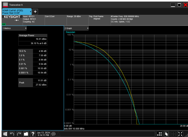
10MHz_15kHz_836.5MHz_DFT-s-OFDM 256 QAM_RB50@0&amp;8.99 dB
