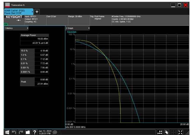
5MHz_15kHz_2535MHz_DFT-s-OFDM PI/2 BPSK_RB25@0&amp;7.12 dB
