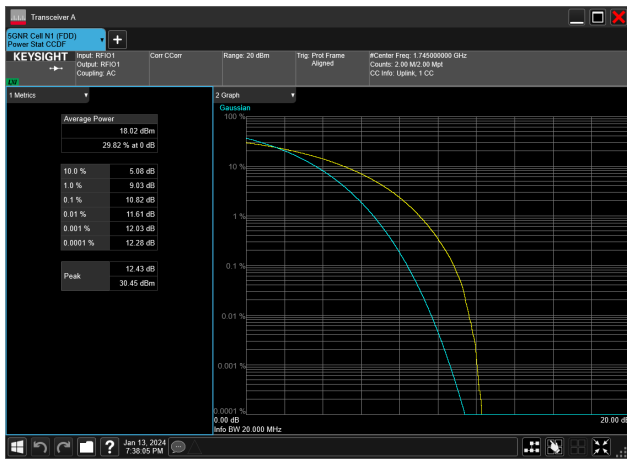
20MHz_15kHz_1745MHz_CP-OFDM QPSK_RB106@0&amp;10.82 dB
