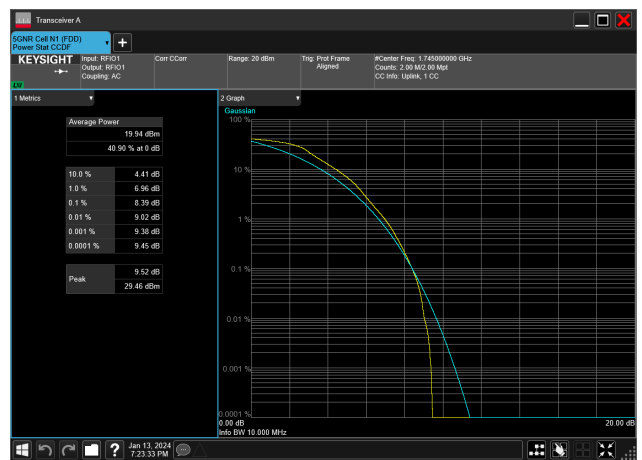
10MHz_15kHz_1745MHz_DFT-s-OFDM QPSK_RB50@0&amp;8.39 dB
