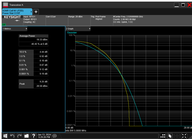
5MHz_15kHz_2535MHz_DFT-s-OFDM QPSK_RB25@0&amp;8.18 dB
