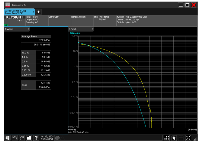
20MHz_15kHz_2535MHz_CP-OFDM 16 QAM_RB106@0&amp;10.68 dB
