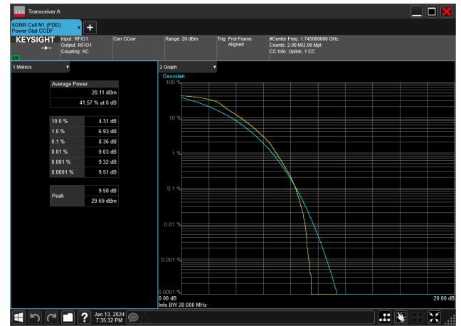
20MHz_15kHz_1745MHz_DFT-s-OFDM QPSK_RB100@0&amp;8.36 dB
