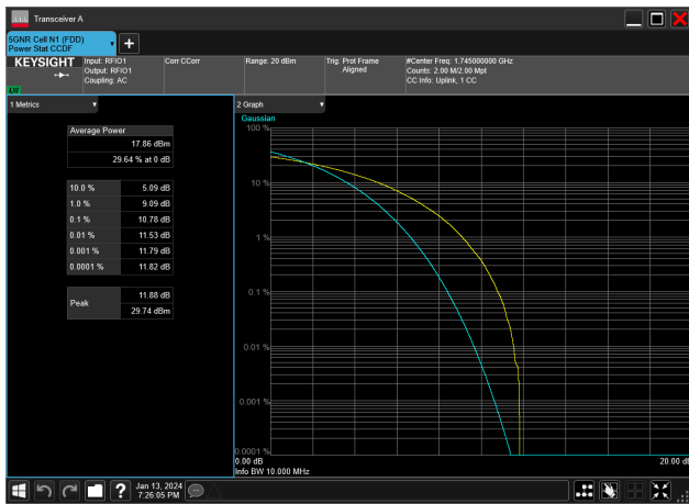
10MHz_15kHz_1745MHz_CP-OFDM QPSK_RB50@0&amp;10.78 dB
