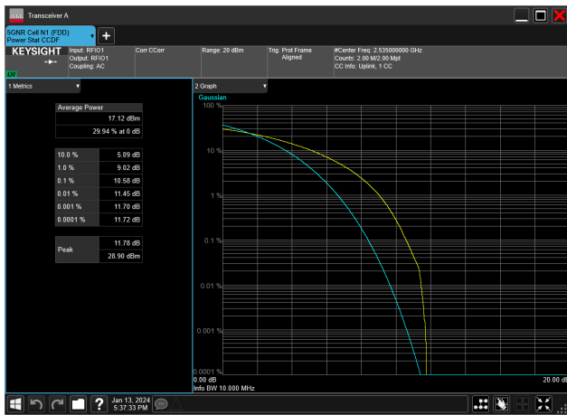
10MHz_15kHz_2535MHz_CP-OFDM QPSK_RB50@0&amp;10.58 dB
