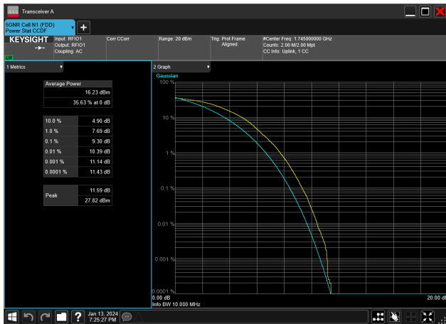
10MHz_15kHz_1745MHz_DFT-s-OFDM 256 QAM_RB50@0&amp;9.30 dB
