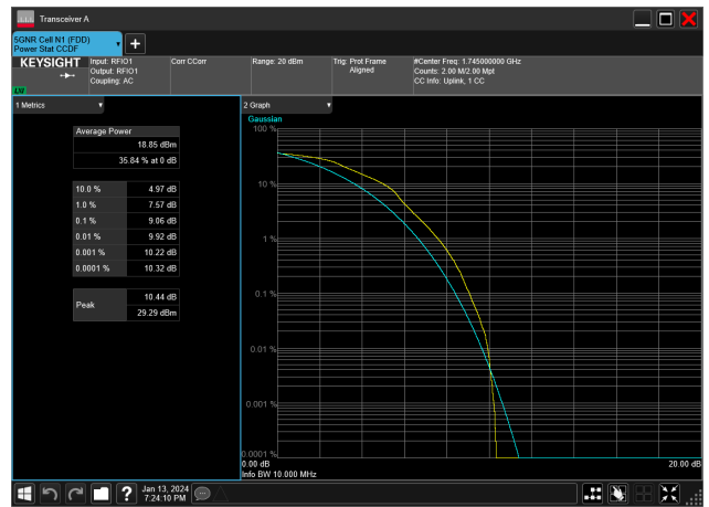
10MHz_15kHz_1745MHz_DFT-s-OFDM 16 QAM_RB50@0&amp;9.06 dB
