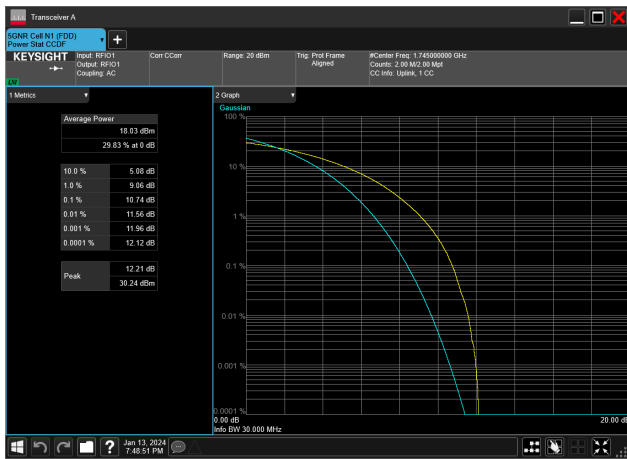
30MHz_15kHz_1745MHz_CP-OFDM QPSK_RB160@0&amp;10.74 dB
