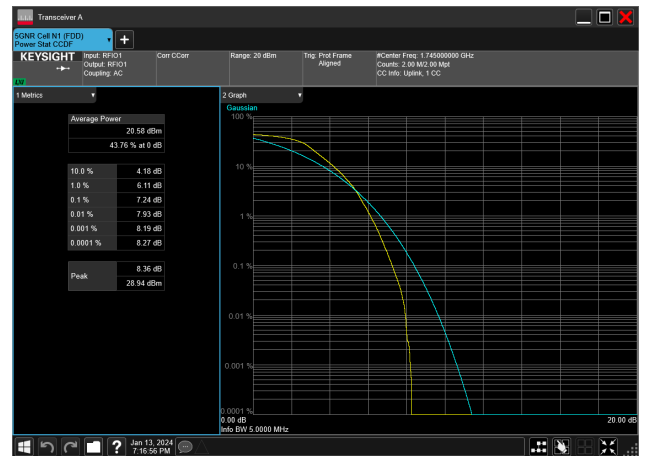
5MHz_15kHz_1745MHz_DFT-s-OFDM PI/2 BPSK_RB25@0&amp;7.24 dB
