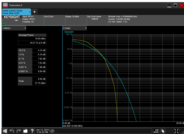
10MHz_15kHz_2535MHz_DFT-s-OFDM PI/2 BPSK_RB50@0&amp;7.05 dB
