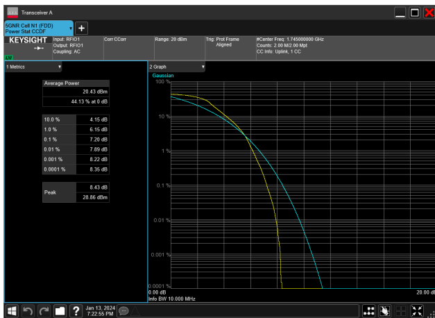
10MHz_15kHz_1745MHz_DFT-s-OFDM PI/2 BPSK_RB50@0&amp;7.20 dB
