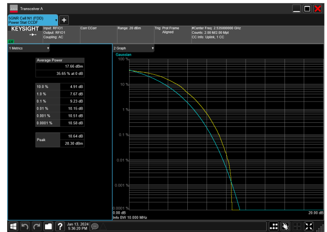
10MHz_15kHz_2535MHz_DFT-s-OFDM 64 QAM_RB50@0&amp;9.23 dB
