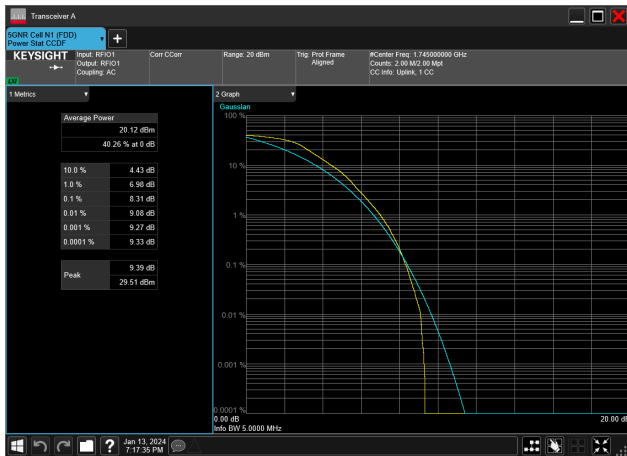
5MHz_15kHz_1745MHz_DFT-s-OFDM QPSK_RB25@0&amp;8.31 dB
