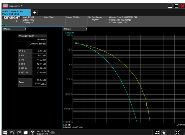
20MHz_15kHz_2535MHz_CP-OFDM 256 QAM_RB106@0&amp;11.32 dB
