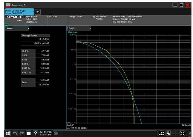
10MHz_15kHz_2535MHz_DFT-s-OFDM 16 QAM_RB50@0&amp;8.92 dB
