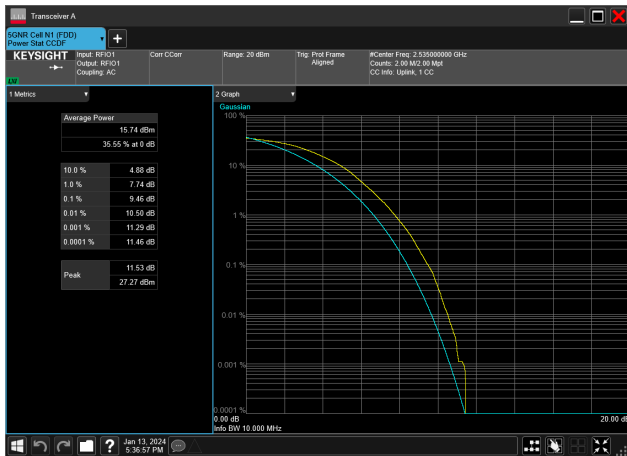
10MHz_15kHz_2535MHz_DFT-s-OFDM 256 QAM_RB50@0&amp;9.46 dB
