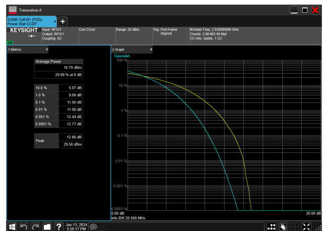
20MHz_15kHz_2535MHz_CP-OFDM 64 QAM_RB106@0&amp;11.00 dB
