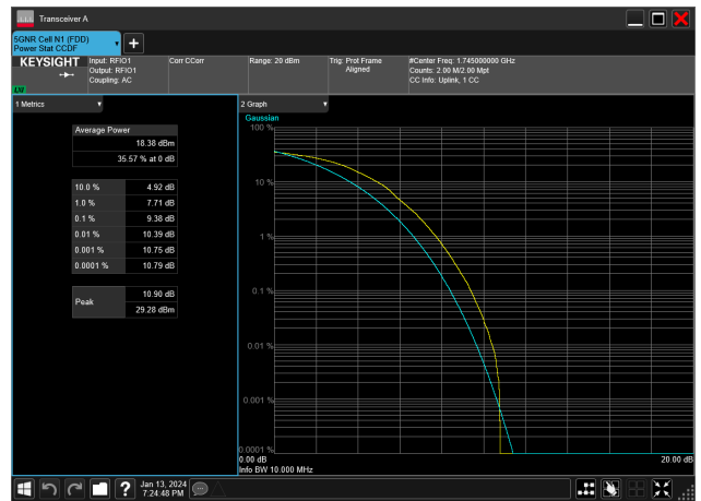
10MHz_15kHz_1745MHz_DFT-s-OFDM 64 QAM_RB50@0&amp;9.38 dB
