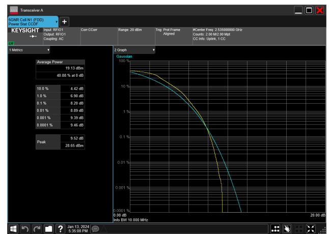
10MHz_15kHz_2535MHz_DFT-s-OFDM QPSK_RB50@0&amp;8.20 dB
