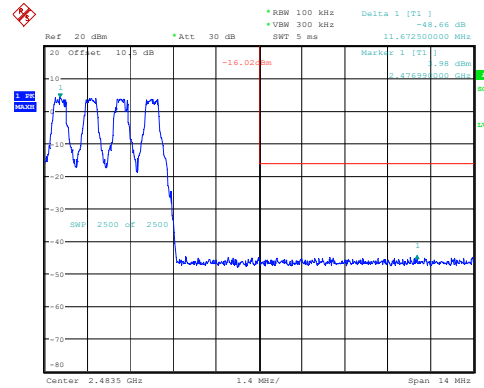
DH1_Hopping_Upper
