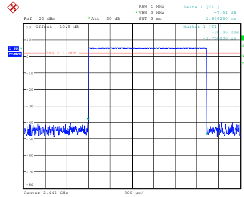
DH3_Hopping 1.646ms
