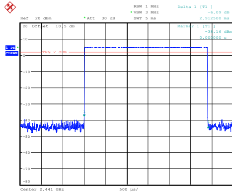
DH5_Hopping 2.913ms
