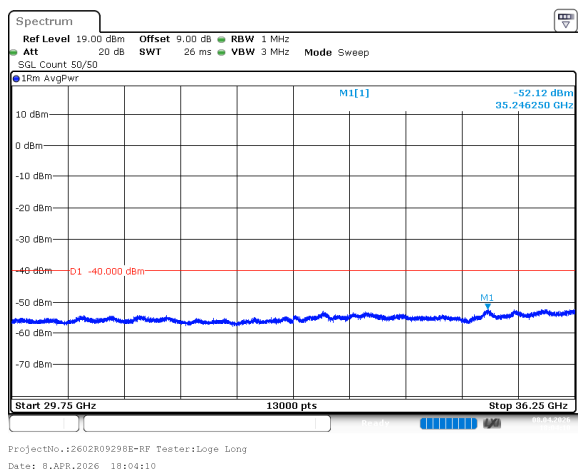
n77_2_25MHz_30kHz_3625MHz_DFT-s-OFDM QPSK_RB1@64 -52.12dBm
