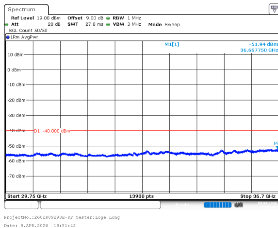
n77_2_60MHz_30kHz_3670MHz_DFT-s-OFDM QPSK_RB162@0 -51.94dBm
