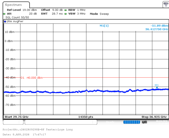
n77_2_15MHz_30kHz_3692.5MHz_DFT-s-OFDM QPSK_RB36@0 -51.89dBm
