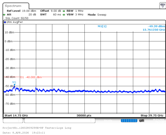
n77_2_90MHz_30kHz_3625MHz_DFT-s-OFDM QPSK_RB243@0 -49.39dBm
