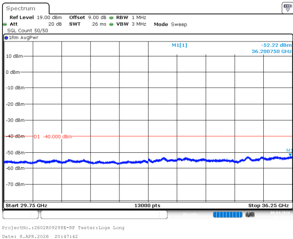
n78_2_50MHz_30kHz_3625MHz_DFT-s-OFDM QPSK_RB1@0 -52.22dBm
