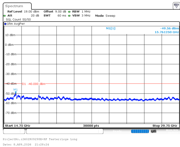
n78_2_90MHz_30kHz_3595MHz_DFT-s-OFDM QPSK_RB1@244 -49.56dBm
