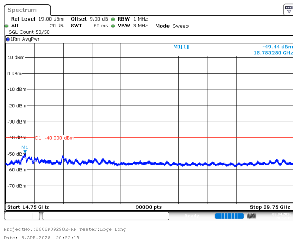
n78_2_50MHz_30kHz_3675MHz_DFT-s-OFDM QPSK_RB1@132 -49.44dBm
