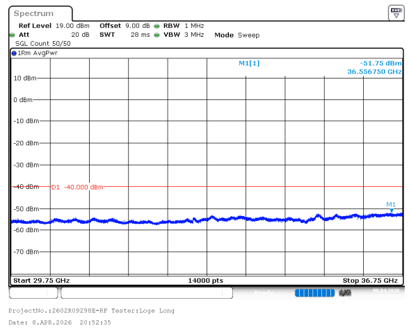
n78_2_50MHz_30kHz_3675MHz_DFT-s-OFDM QPSK_RB1@132 -51.75dBm
