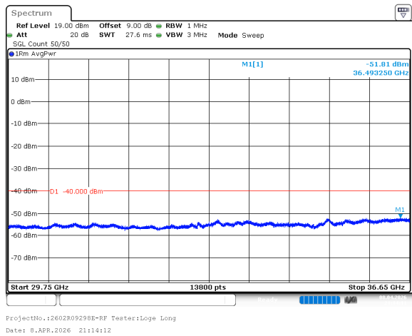
n78_2_70MHz_30kHz_3665MHz_DFT-s-OFDM QPSK_RB1@188 -51.81dBm
