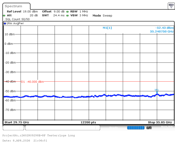
n78_2_70MHz_30kHz_3585MHz_DFT-s-OFDM QPSK_RB1@188 -52.43dBm
