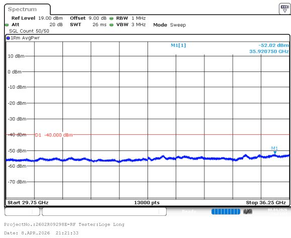
n78_2_80MHz_30kHz_3625MHz_DFT-s-OFDM QPSK_RB1@216 -52.02dBm
