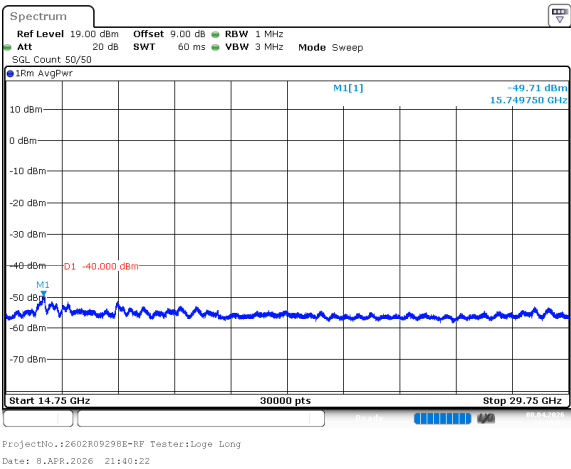
n78_2_100MHz_30kHz_3600MHz_DFT-s-OFDM QPSK_RB270@0 -49.71dBm
