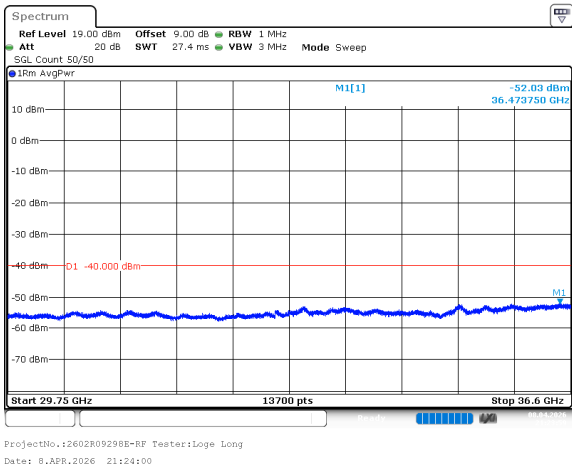
n78_2_80MHz_30kHz_3660MHz_DFT-s-OFDM QPSK_RB1@0 -52.03dBm
