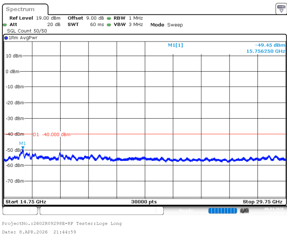
n78_2_100MHz_30kHz_3650MHz_DFT-s-OFDM QPSK_RB1@0 -49.45dBm
