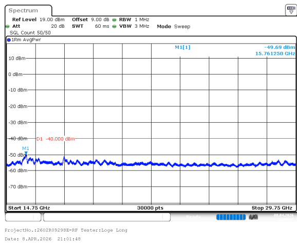
n78_2_60MHz_30kHz_3670MHz_DFT-s-OFDM QPSK_RB1@0 -49.69dBm
