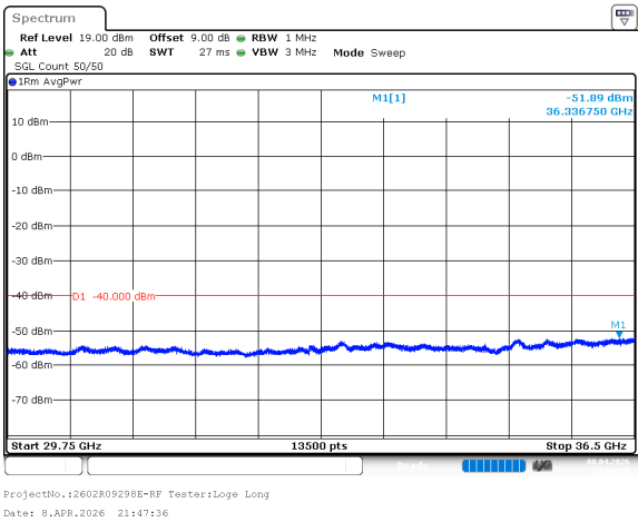
n78_2_100MHz_30kHz_3650MHz_DFT-s-OFDM QPSK_RB270@0 -51.89dBm
