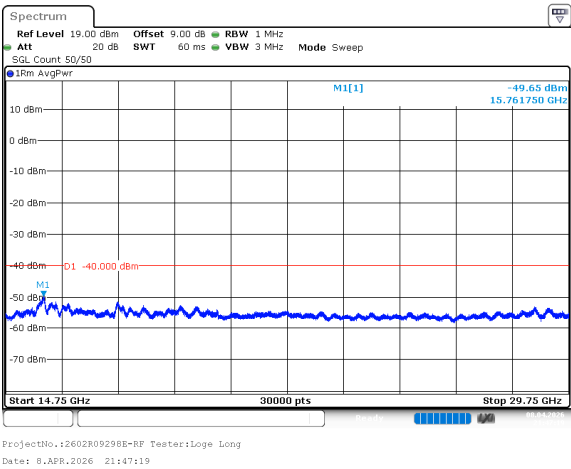
n78_2_100MHz_30kHz_3650MHz_DFT-s-OFDM QPSK_RB270@0 -49.65dBm
