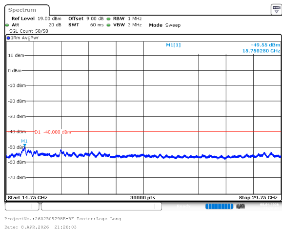
n78_2_80MHz_30kHz_3660MHz_DFT-s-OFDM QPSK_RB216@0 -49.55dBm
