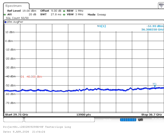
n78_2_60MHz_30kHz_3670MHz_DFT-s-OFDM QPSK_RB162@0 -51.93dBm
