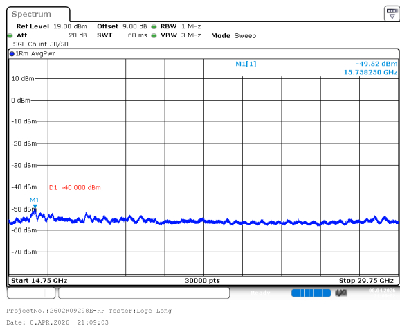
n78_2_70MHz_30kHz_3625MHz_DFT-s-OFDM QPSK_RB1@0 -49.52dBm
