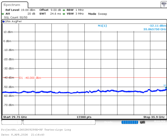
n78_2_80MHz_30kHz_3590MHz_DFT-s-OFDM QPSK_RB1@0 -52.11dBm
