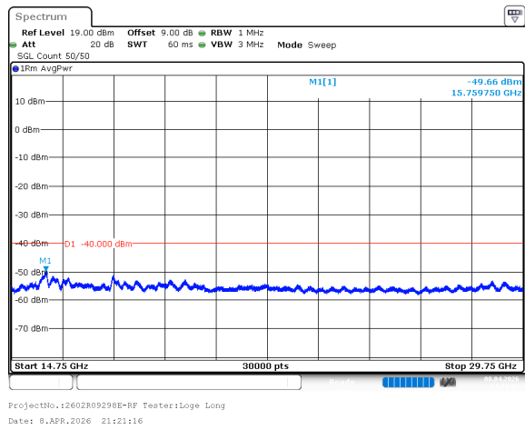
n78_2_80MHz_30kHz_3625MHz_DFT-s-OFDM QPSK_RB1@216 -49.66dBm
