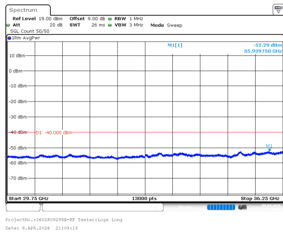
n78_2_70MHz_30kHz_3625MHz_DFT-s-OFDM QPSK_RB1@0 -52.29dBm
