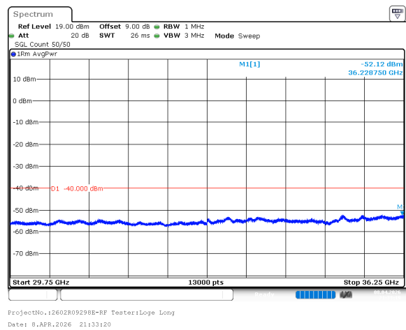
n78_2_90MHz_30kHz_3625MHz_DFT-s-OFDM QPSK_RB243@0 -52.12dBm
