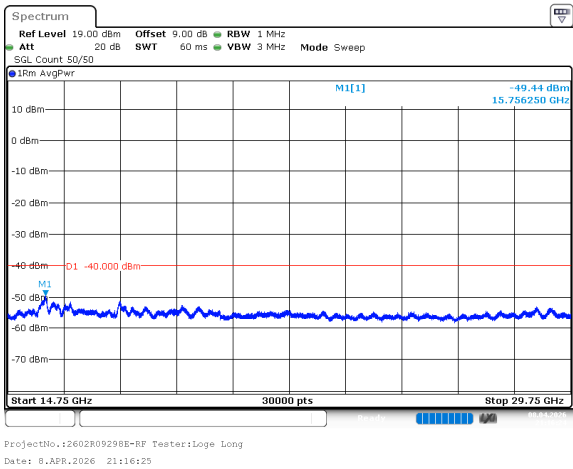
n78_2_80MHz_30kHz_3590MHz_DFT-s-OFDM QPSK_RB1@0 -49.44dBm
