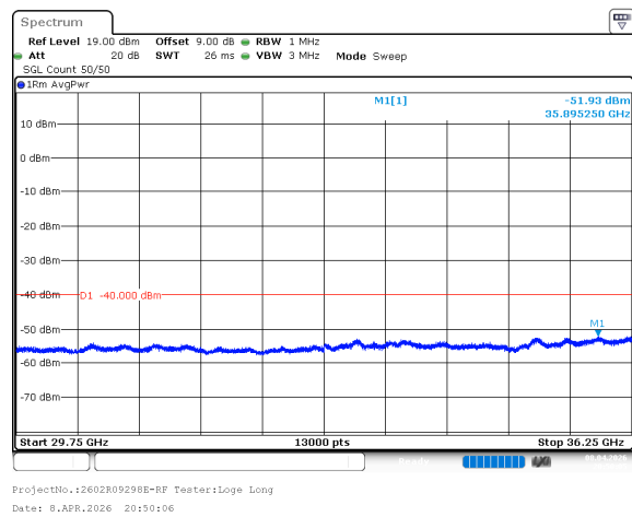
n78_2_50MHz_30kHz_3625MHz_DFT-s-OFDM QPSK_RB128@0 -51.93dBm
