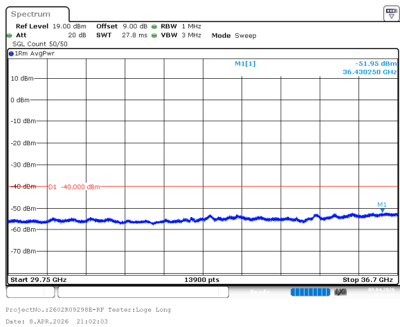
n78_2_60MHz_30kHz_3670MHz_DFT-s-OFDM QPSK_RB1@0 -51.95dBm
