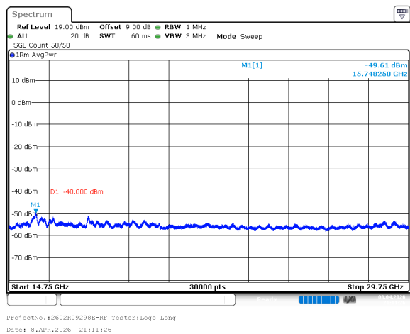
n78_2_70MHz_30kHz_3625MHz_DFT-s-OFDM QPSK_RB180@0 -49.61dBm
