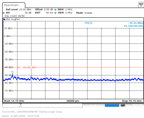
n78_2_60MHz_30kHz_3580MHz_DFT-s-OFDM QPSK_RB162@0 -49.45dBm
