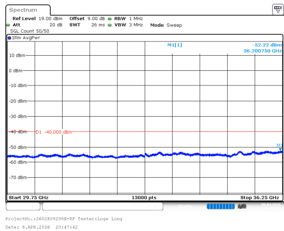
n78_2_50MHz_30kHz_3625MHz_DFT-s-OFDM QPSK_RB1@0 -52.22dBm
