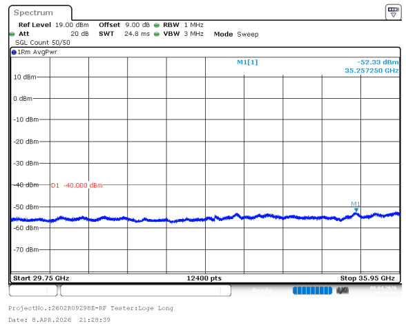
n78_2_90MHz_30kHz_3595MHz_DFT-s-OFDM QPSK_RB1@244 -52.33dBm
