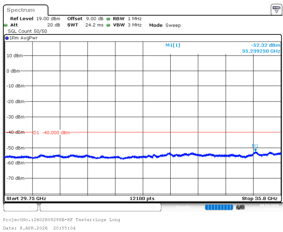
n78_2_60MHz_30kHz_3580MHz_DFT-s-OFDM QPSK_RB1@0 -52.32dBm
