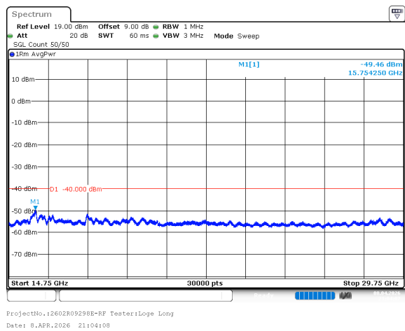
n78_2_60MHz_30kHz_3670MHz_DFT-s-OFDM QPSK_RB162@0 -49.46dBm
