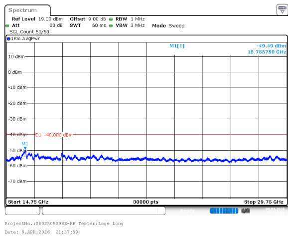
n78_2_100MHz_30kHz_3600MHz_DFT-s-OFDM QPSK_RB1@0 -49.49dBm
