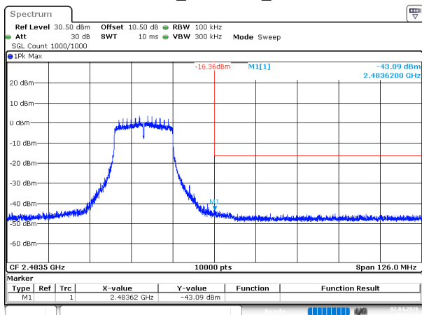
802.11n20_2462MHz_Chain 0
