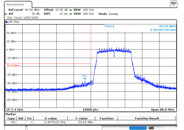
802.11n20_2412MHz_Chain 0
