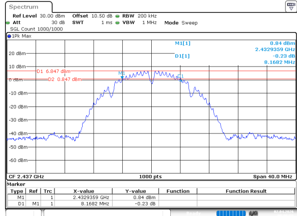
802.11b_2437MHz_Chain 0
