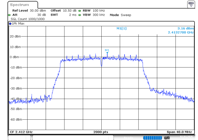
802.11n20_2412MHz_Chain 0
