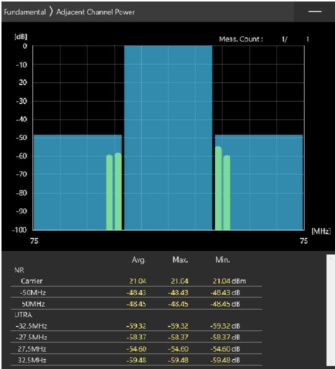
50MHz_30kHz_3575MHz-OFDM QPSK_RB1@132 -48.43,-48.45dB
