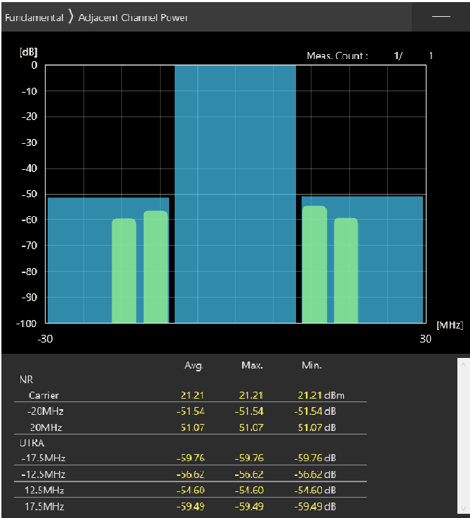
20MHz_30kHz_3690MHz-OFDM QPSK_RB1@50 -51.54,-51.07dB
