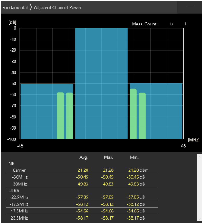
30MHz_30kHz_3685MHz-OFDM QPSK_RB1@77 -50.45,-49.83dB
