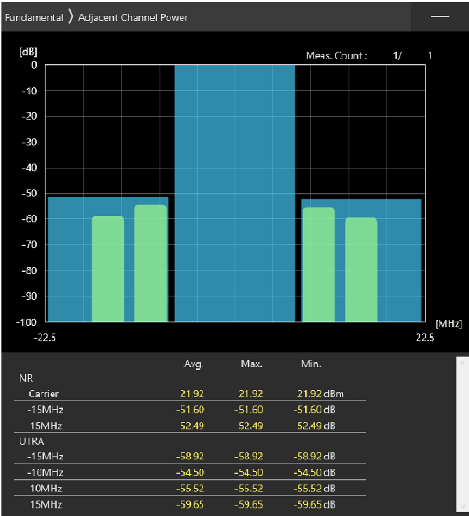
15MHz_30kHz_3557.5MHz-OFDM QPSK_RB18@9 -51.6,-52.49dB
