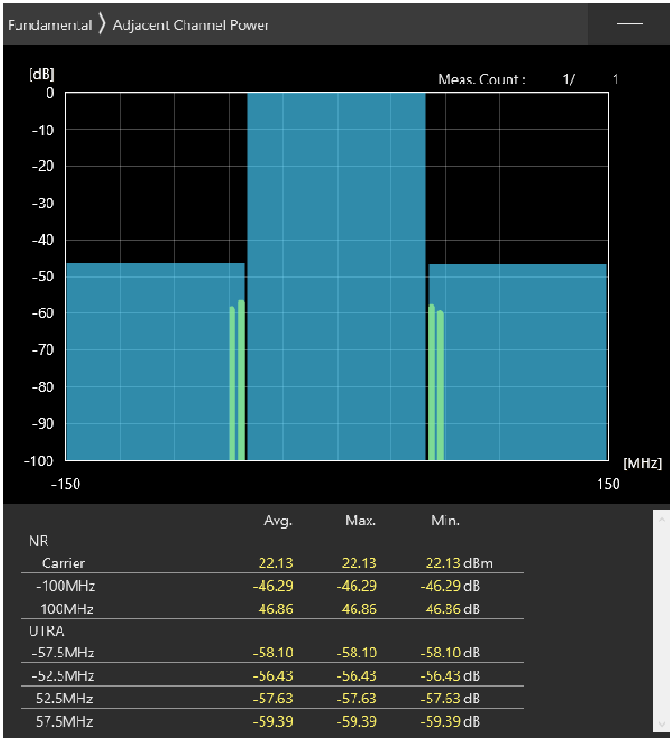
100MHz_30kHz_3650MHz-OFDM QPSK_RB135@67 -46.29,-46.86dB
