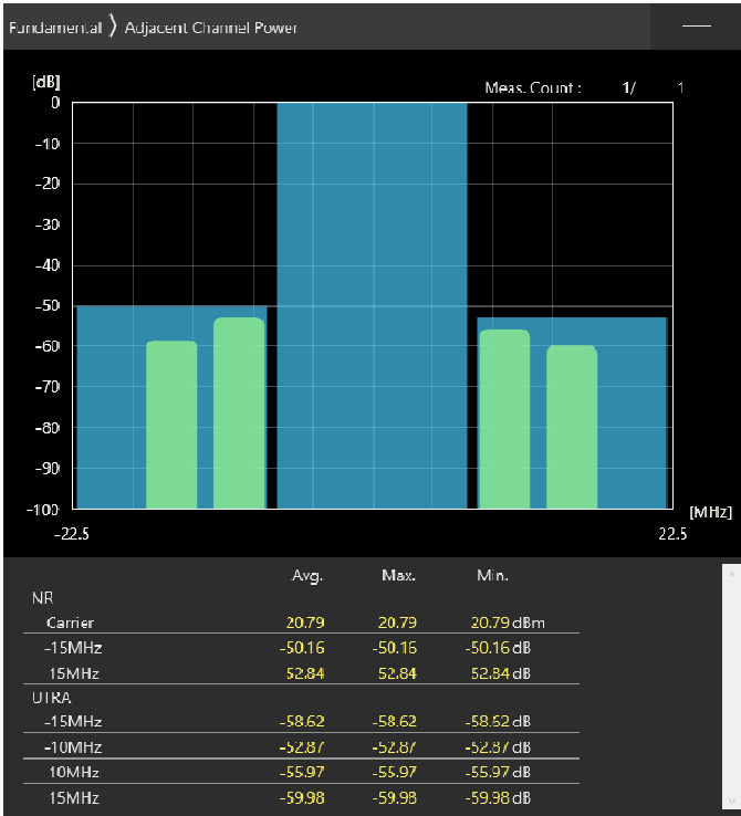
15MHz_30kHz_3557.5MHz-OFDM QPSK_RB1@0 -50.16,-52.84dB
