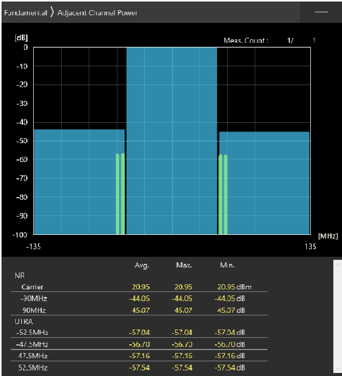
90MHz_30kHz_3595MHz-OFDM QPSK_RB243@0 -44.05,-45.07dB
