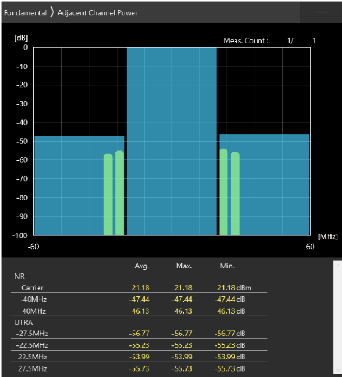
40MHz_30kHz_3680MHz-OFDM QPSK_RB100@0 -47.44,-46.13dB
