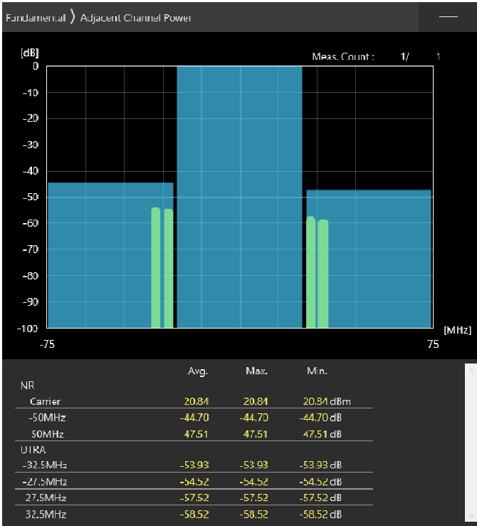
50MHz_30kHz_3575MHz-OFDM QPSK_RB128@0 -44.7,-47.51dB
