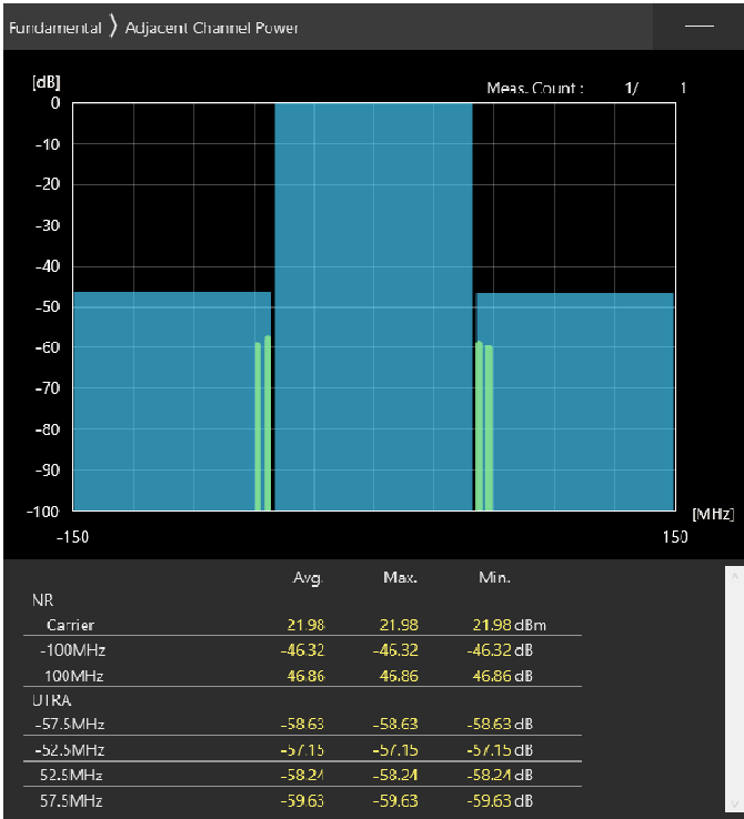
100MHz_30kHz_3600MHz-OFDM QPSK_RB135@67 -46.32,-46.86dB
