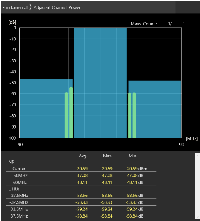
60MHz_30kHz_3580MHz-OFDM QPSK_RB1@0 -47.08,-48.11dB
