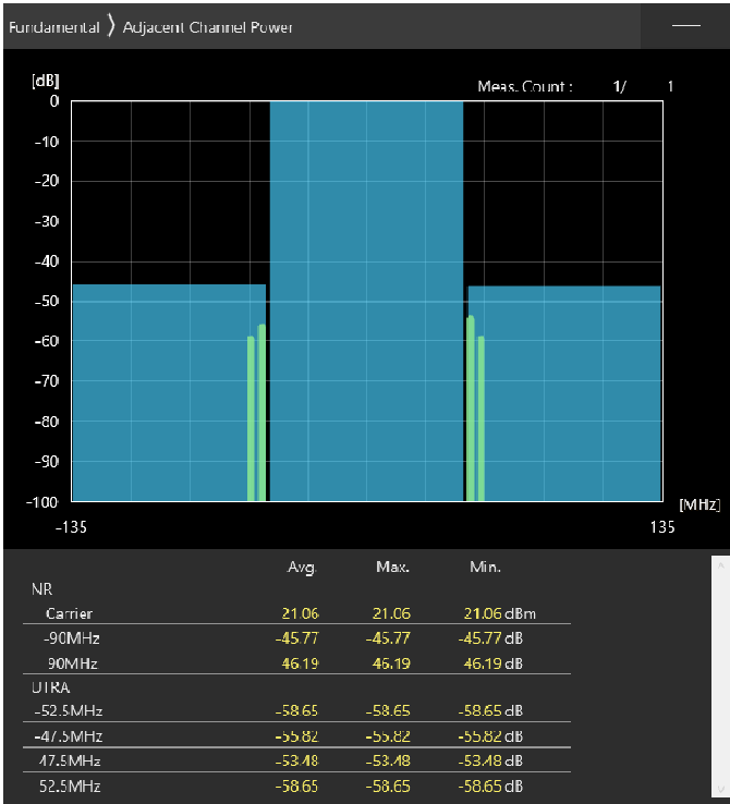
90MHz_30kHz_3655MHz-OFDM QPSK_RB1@244 -45.77,-46.19dB
