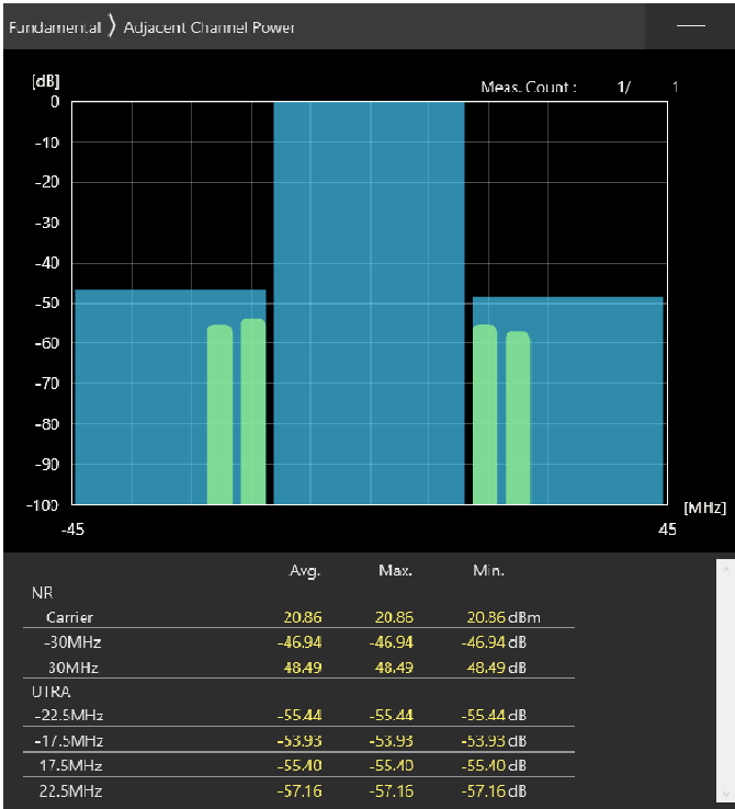
30MHz_30kHz_3565MHz-OFDM QPSK_RB75@0 -46.94,-48.49dB
