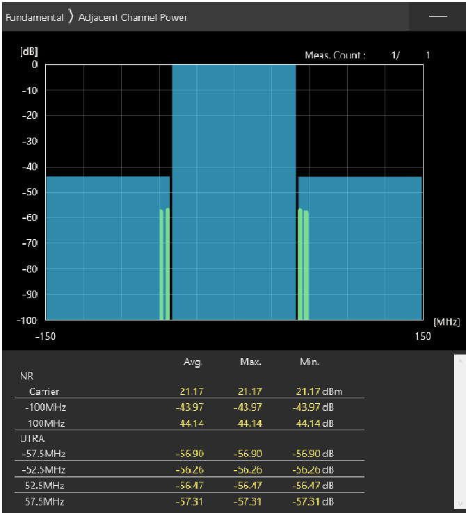
100MHz_30kHz_3650MHz-OFDM QPSK_RB270@0 -43.97,-44.14dB
