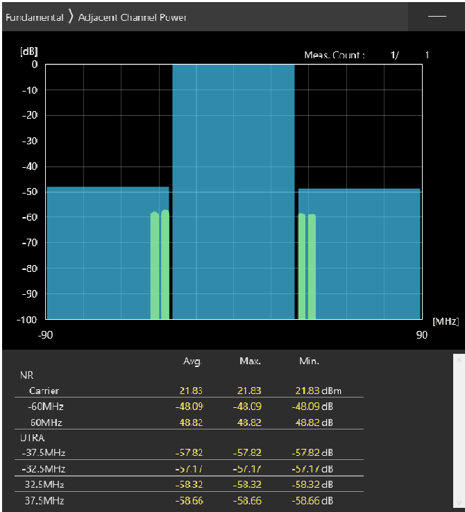
60MHz_30kHz_3580MHz-OFDM QPSK_RB81@40 -48.09,-48.82dB
