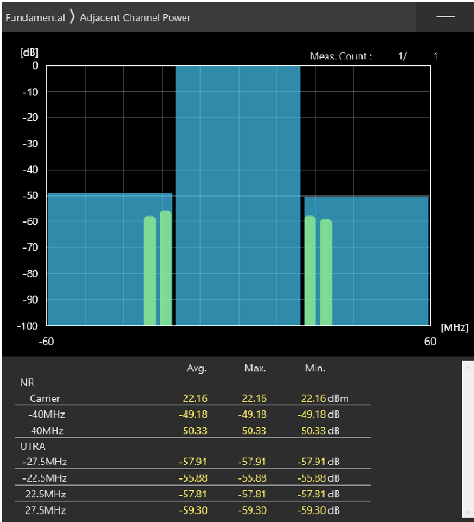
40MHz_30kHz_3680MHz-OFDM QPSK_RB50@25 -49.18,-50.33dB
