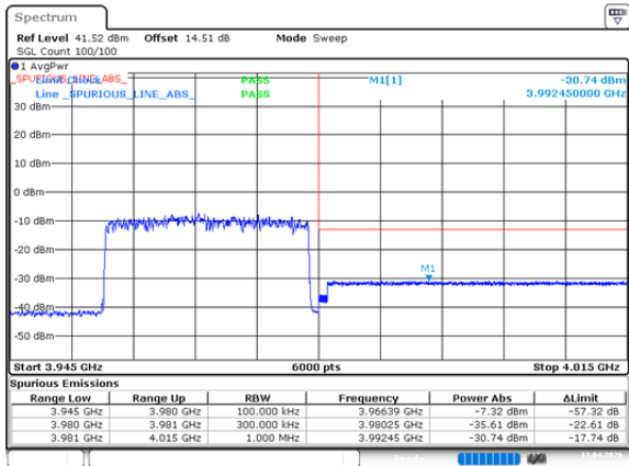
n77_3_25MHz_30kHz_3967.5MHz_DFT-s-OFDM QPSK_RB64@0
