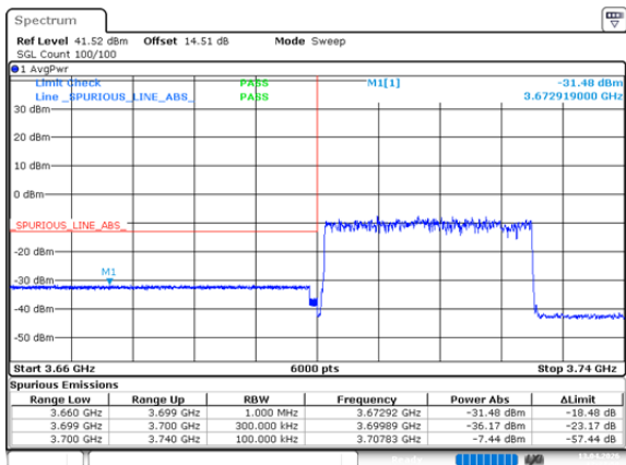
n77_3_30MHz_30kHz_3715MHz_DFT-s-OFDM QPSK_RB75@0
