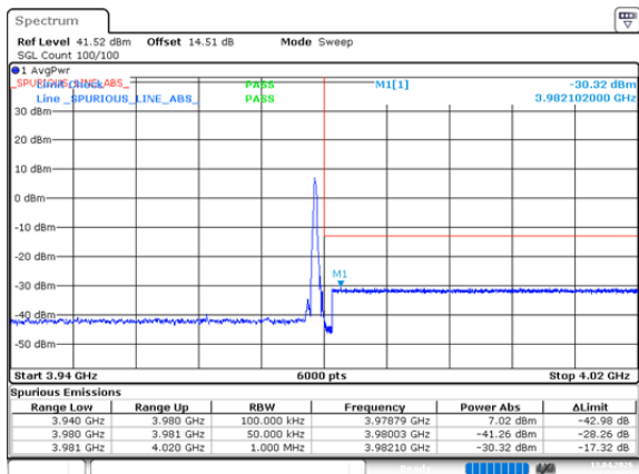
n77_3_30MHz_30kHz_3965MHz_DFT-s-OFDM QPSK_RB1@77
