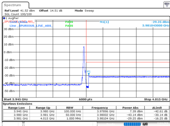
n77_3_25MHz_30kHz_3967.5MHz_DFT-s-OFDM QPSK_RB1@64
