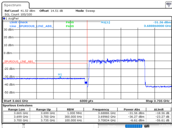
n77_3_25MHz_30kHz_3712.5MHz_DFT-s-OFDM QPSK_RB64@0
