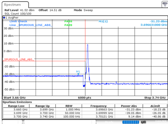
n77_3_30MHz_30kHz_3715MHz_DFT-s-OFDM QPSK_RB1@0
