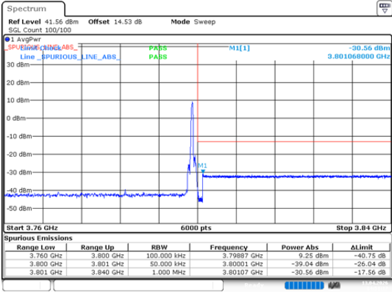
n78_3_30MHz_30kHz_3785MHz_DFT-s-OFDM QPSK_RB1@77
