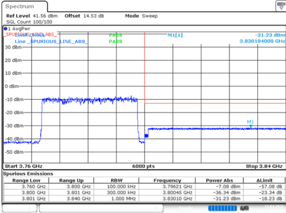
n78_3_30MHz_30kHz_3785MHz_DFT-s-OFDM QPSK_RB75@0
