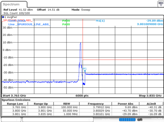
n78_3_25MHz_30kHz_3787.5MHz_DFT-s-OFDM QPSK_RB1@64
