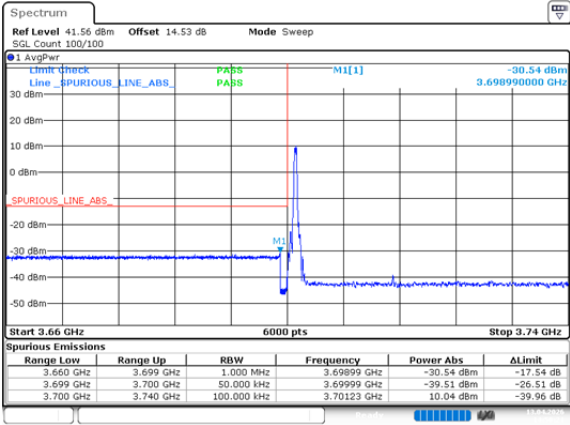
n78_3_30MHz_30kHz_3715MHz_DFT-s-OFDM QPSK_RB1@0
