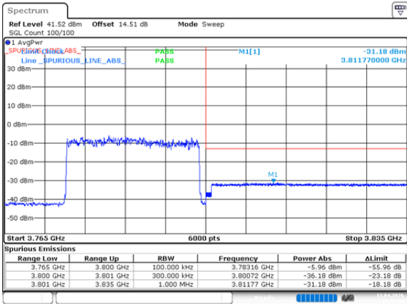
n78_3_25MHz_30kHz_3787.5MHz_DFT-s-OFDM QPSK_RB64@0
