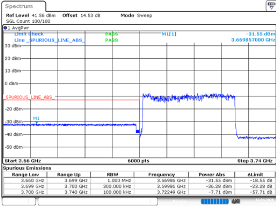
n78_3_30MHz_30kHz_3715MHz_DFT-s-OFDM QPSK_RB75@0
