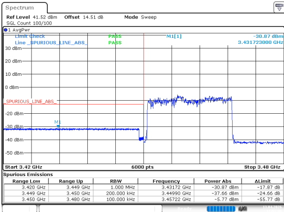
n77_1_20MHz_30kHz_3460MHz_DFT-s-OFDM QPSK_RB50@0
