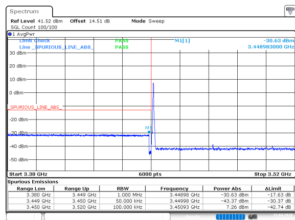
n77_1_60MHz_30kHz_3480MHz_DFT-s-OFDM QPSK_RB1@0
