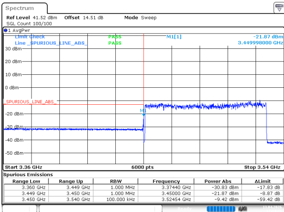
n77_1_80MHz_30kHz_3490MHz_DFT-s-OFDM QPSK_RB216@0
