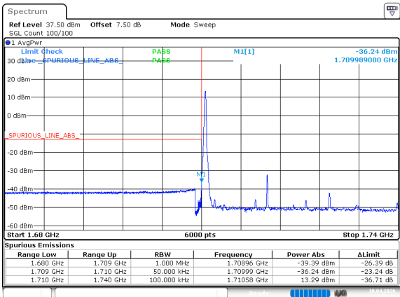
n66_20MHz_15kHz_1720MHz_DFT-s-OFDM QPSK_RB1@0
