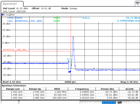
n77_1_20MHz_30kHz_3460MHz_DFT-s-OFDM QPSK_RB1@0
