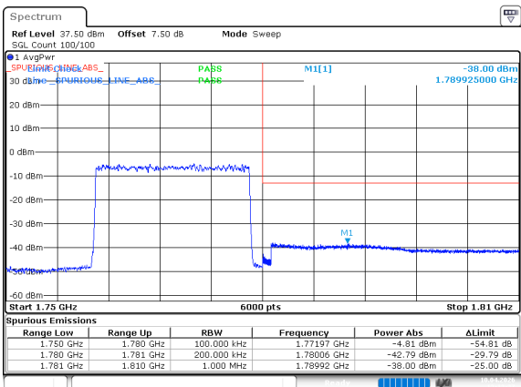
n66_20MHz_15kHz_1770MHz_DFT-s-OFDM QPSK_RB100@0
