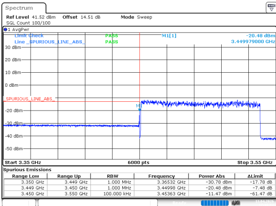
n77_1_90MHz_30kHz_3495MHz_DFT-s-OFDM QPSK_RB243@0
