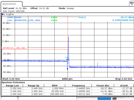
n77_1_90MHz_30kHz_3495MHz_DFT-s-OFDM QPSK_RB1@0
