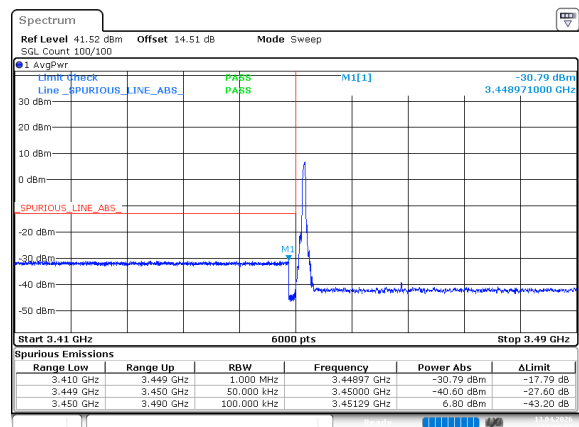
n77_1_30MHz_30kHz_3465MHz_DFT-s-OFDM QPSK_RB1@0
