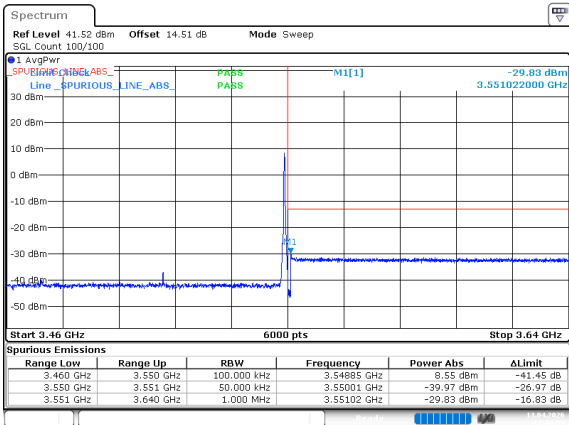
n77_1_80MHz_30kHz_3510MHz_DFT-s-OFDM QPSK_RB1@216
