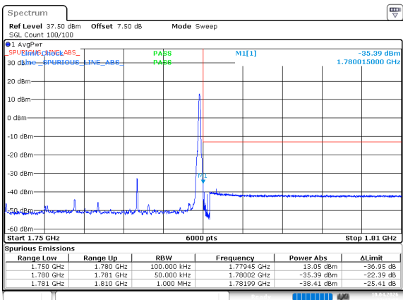
n66_20MHz_15kHz_1770MHz_DFT-s-OFDM QPSK_RB1@105
