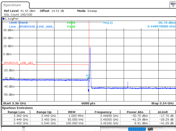
n77_1_80MHz_30kHz_3490MHz_DFT-s-OFDM QPSK_RB1@0
