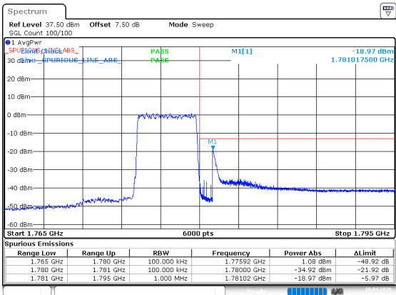
n66_5MHz_15kHz_1777.5MHz_DFT-s-OFDM QPSK_RB1@24 n66_5MHz_15kHz_1777.5MHz_DFT-s-OFDM QPSK_RB25@0
