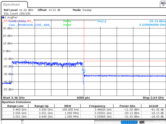
n77_1_80MHz_30kHz_3510MHz_DFT-s-OFDM QPSK_RB216@0
