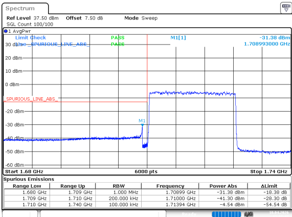
n66_20MHz_15kHz_1720MHz_DFT-s-OFDM QPSK_RB100@0
