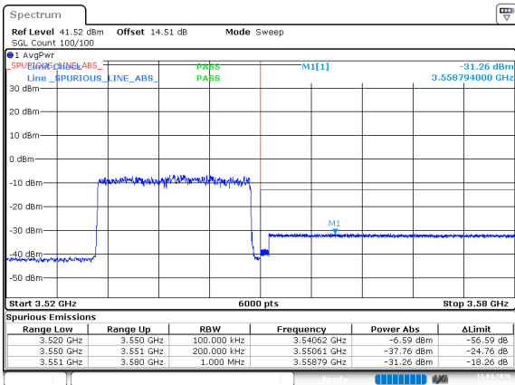
n77_1_20MHz_30kHz_3540MHz_DFT-s-OFDM QPSK_RB50@0
