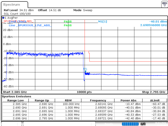
n41_100MHz_30kHz_2640MHz_DFT-s-OFDM QPSK_RB270@0
