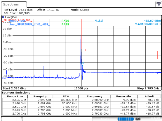
n41_100MHz_30kHz_2640MHz_DFT-s-OFDM QPSK_RB1@272
