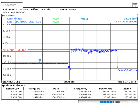
n77_1_30MHz_30kHz_3465MHz_DFT-s-OFDM QPSK_RB75@0
