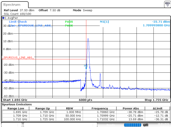
n66 n66_5MHz_15kHz_1712.5MHz_DFT-s-OFDM QPSK_RB1@0 n66_5MHz_15kHz_1712.5MHz_DFT-s-OFDM QPSK_RB25@0
