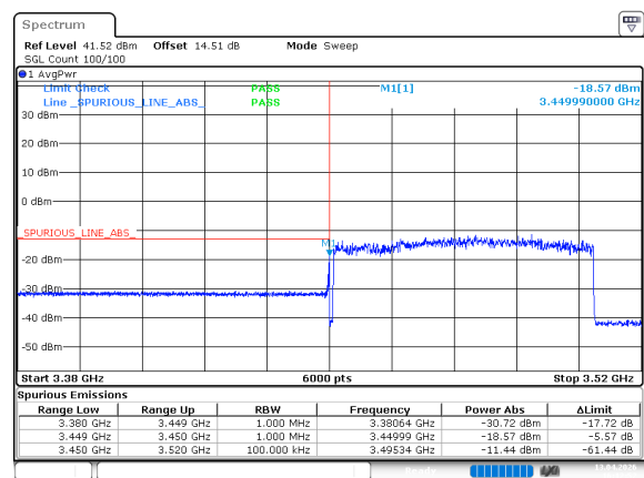
n77_1_60MHz_30kHz_3480MHz_DFT-s-OFDM QPSK_RB162@0
