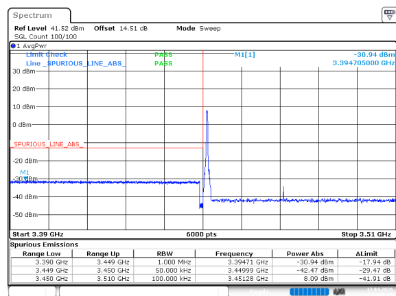
n77_1_50MHz_30kHz_3475MHz_DFT-s-OFDM QPSK_RB1@0
