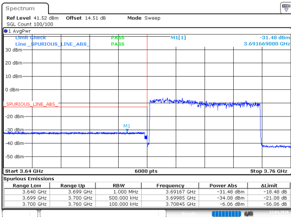
n78_3_50MHz_30kHz_3725MHz_DFT-s-OFDM QPSK_RB128@0
