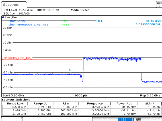
n78_3_40MHz_30kHz_3720MHz_DFT-s-OFDM QPSK_RB100@0
