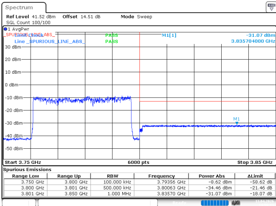
n78_3_40MHz_30kHz_3780MHz_DFT-s-OFDM QPSK_RB100@0
