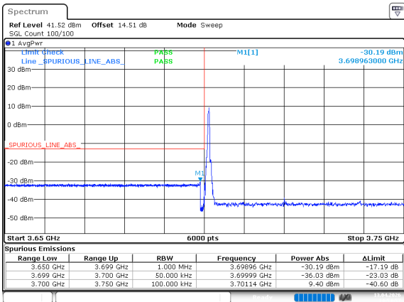
n78_3_40MHz_30kHz_3720MHz_DFT-s-OFDM QPSK_RB1@0
