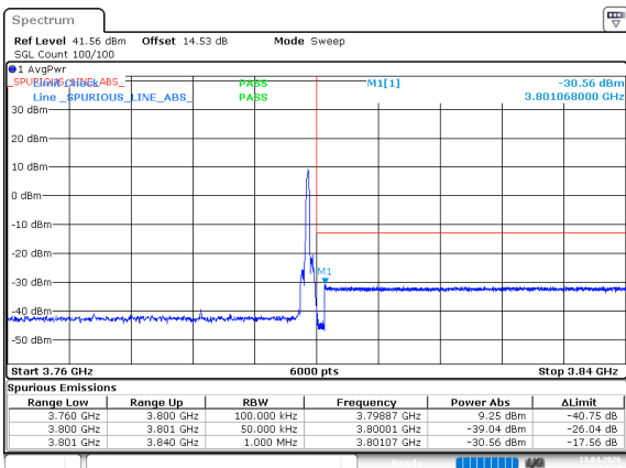
n78_3_30MHz_30kHz_3785MHz_DFT-s-OFDM QPSK_RB1@77
