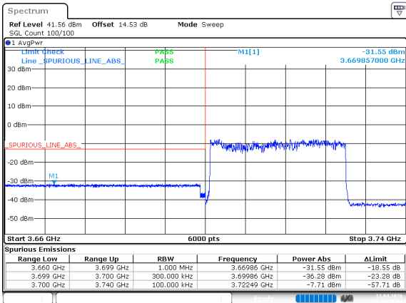
n78_3_30MHz_30kHz_3715MHz_DFT-s-OFDM QPSK_RB75@0
