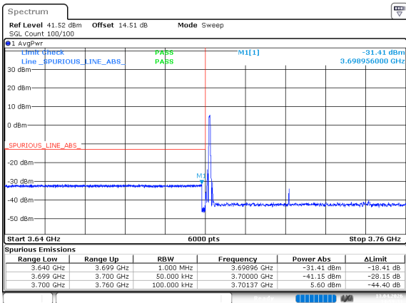
n78_3_50MHz_30kHz_3725MHz_DFT-s-OFDM QPSK_RB1@0
