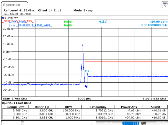
n78_3_25MHz_30kHz_3787.5MHz_DFT-s-OFDM QPSK_RB1@64
