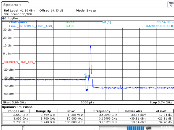
n78_3_30MHz_30kHz_3715MHz_DFT-s-OFDM QPSK_RB1@0
