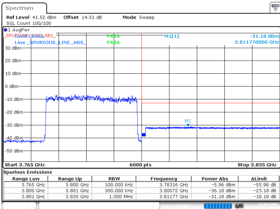
n78_3_25MHz_30kHz_3787.5MHz_DFT-s-OFDM QPSK_RB64@0
