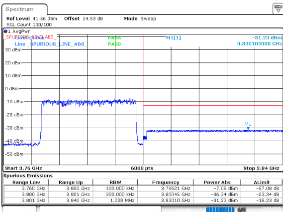
n78_3_30MHz_30kHz_3785MHz_DFT-s-OFDM QPSK_RB75@0
