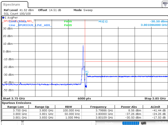
n78_3_40MHz_30kHz_3780MHz_DFT-s-OFDM QPSK_RB1@105
