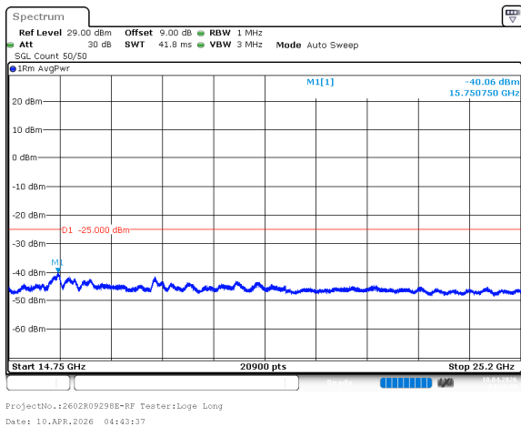
n7_40MHz_15kHz_2520MHz_DFT-s-OFDM QPSK_RB216@0 -40.06dBm
