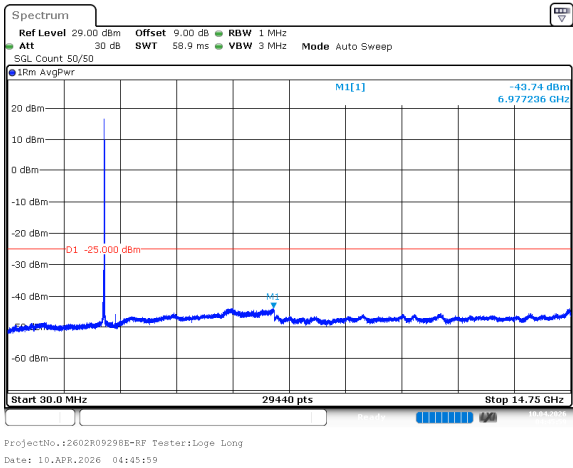
n7_40MHz_15kHz_2535MHz_DFT-s-OFDM QPSK_RB216@0 -43.74dBm
