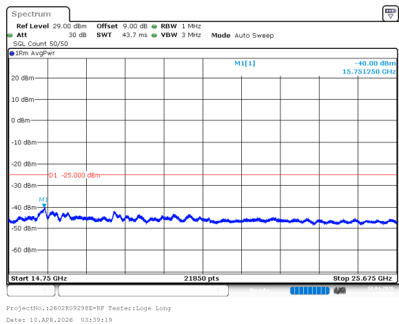
n7_5MHz_15kHz_2567.5MHz_DFT-s-OFDM QPSK_RB25@0 -40dBm
