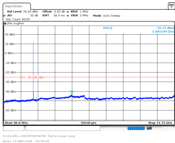
n7_5MHz_15kHz_2567.5MHz_DFT-s-OFDM QPSK_RB25@0 -43.72dBm
