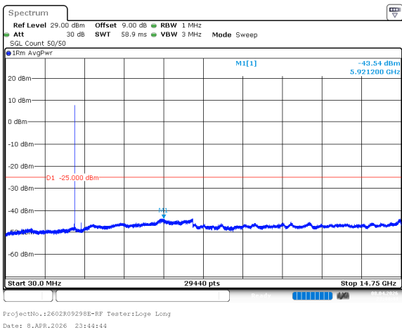
n38_10MHz_30kHz_2595MHz_DFT-s-OFDM QPSK_RB1@23 -43.54dBm
