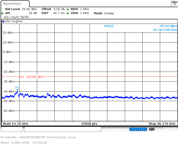
n38_5MHz_15kHz_2617.5MHz_DFT-s-OFDM QPSK_RB1@0 -39.55dBm
