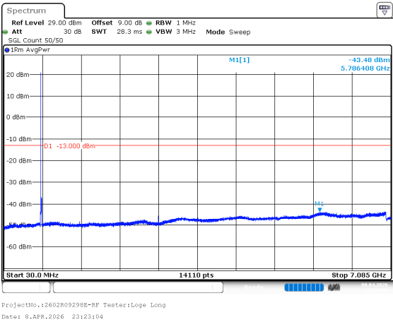
n12_15MHz_15kHz_708.5MHz_DFT-s-OFDM QPSK_RB1@0 -43.48dBm
