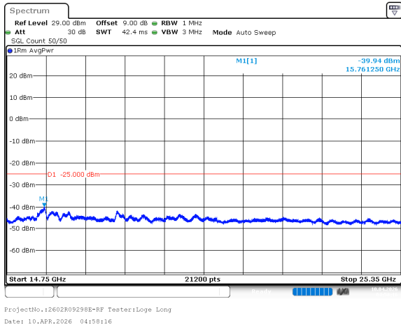
n7_50MHz_15kHz_2535MHz_DFT-s-OFDM QPSK_RB270@0 -39.94dBm
