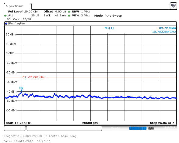
n7_10MHz_15kHz_2505MHz_DFT-s-OFDM QPSK_RB50@0 -39.72dBm
