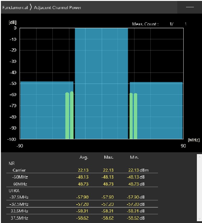
60MHz_30kHz_3670MHz-OFDM QPSK_RB81@40 -48.13,-48.73dB
