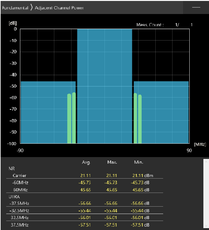
60MHz_30kHz_3670MHz-OFDM QPSK_RB162@0 -45.73,-45.65dB
