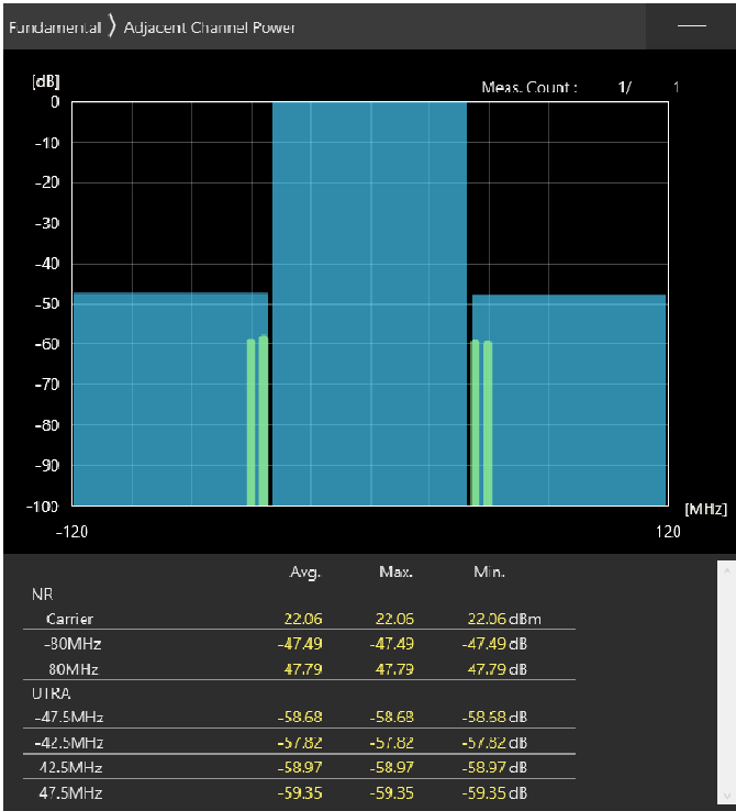
80MHz_30kHz_3660MHz-OFDM QPSK_RB108@54 -47.49,-47.79dB
