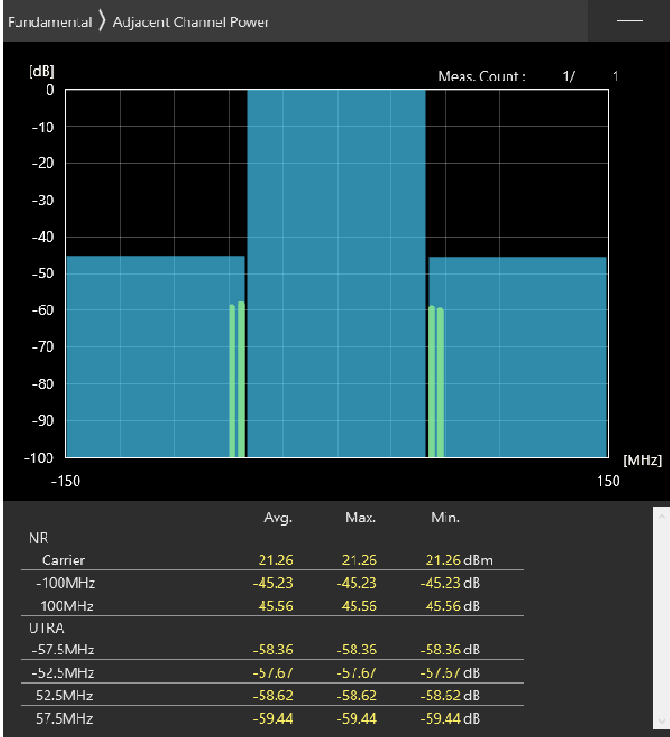
100MHz_30kHz_3650MHz-OFDM QPSK_RB135@67 -45.23,-45.56dB
