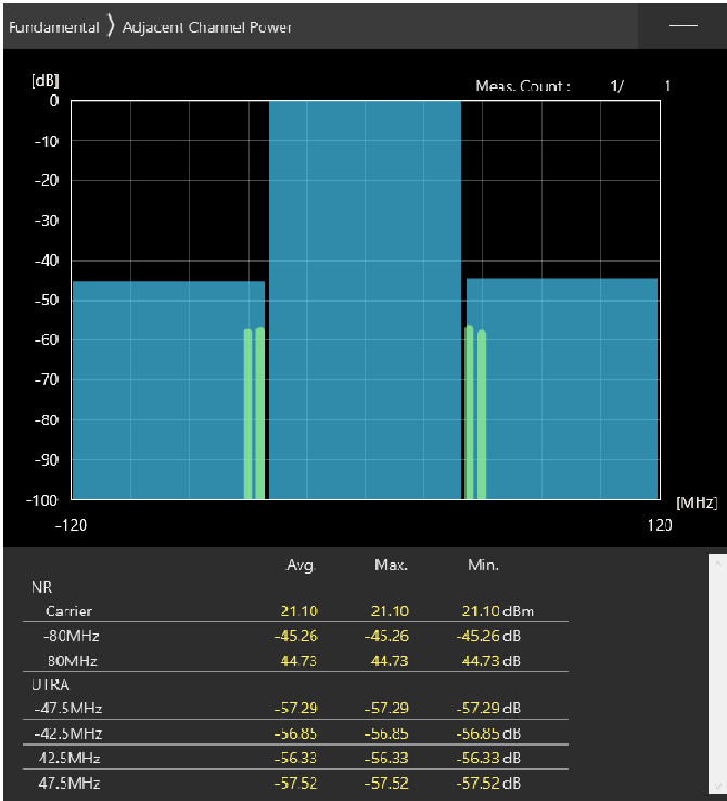
80MHz_30kHz_3660MHz-OFDM QPSK_RB216@0 -45.26,-44.73dB
