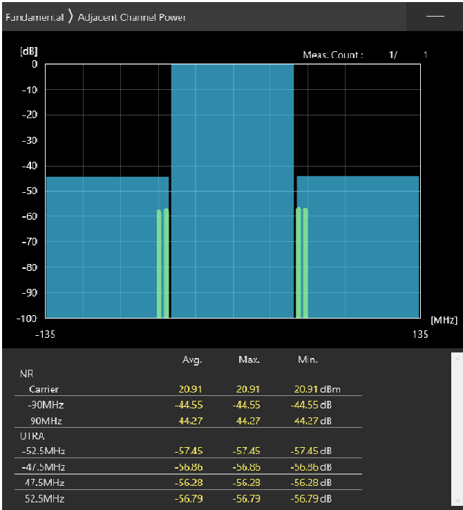
90MHz_30kHz_3595MHz-OFDM QPSK_RB243@0 -44.55,-44.27dB
