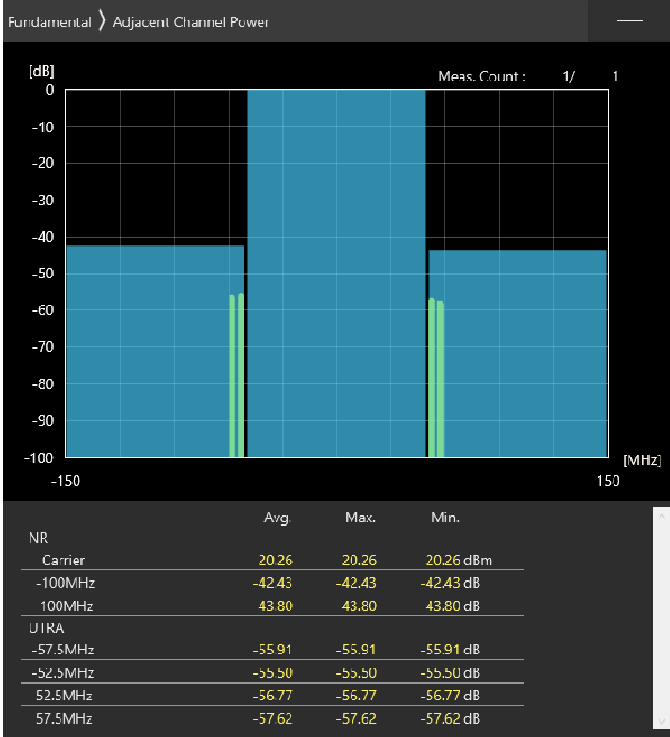
100MHz_30kHz_3650MHz-OFDM QPSK_RB270@0 -42.43,-43.8dB
