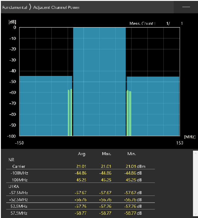
100MHz_30kHz_3600MHz-OFDM QPSK_RB135@67 -44.86,-45.25dB
