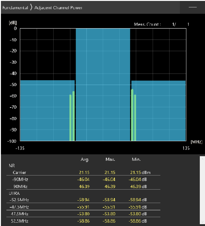
90MHz_30kHz_3655MHz-OFDM QPSK_RB1@244 -46.04,-46.39dB
