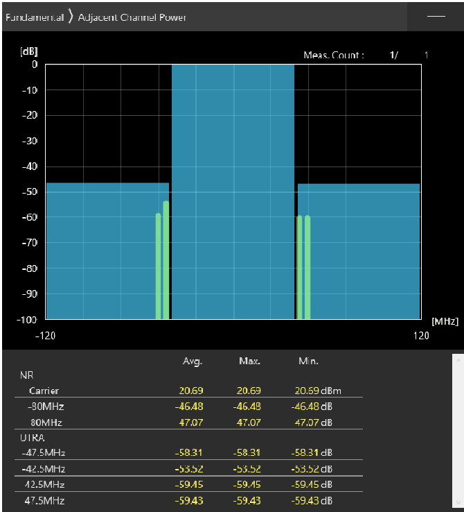
80MHz_30kHz_3590MHz-OFDM QPSK_RB1@0 -46.48,-47.07dB
