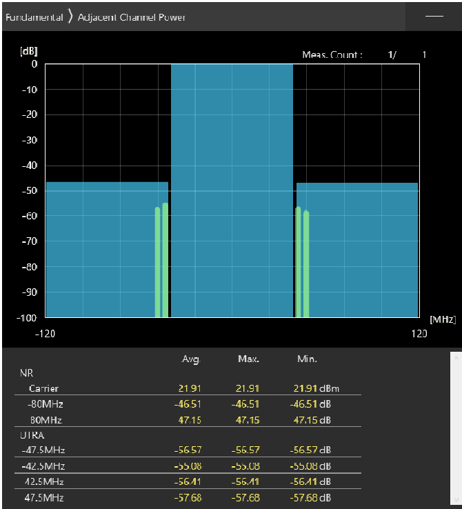
80MHz_30kHz_3590MHz-OFDM QPSK_RB108@54 -46.51,-47.15dB
