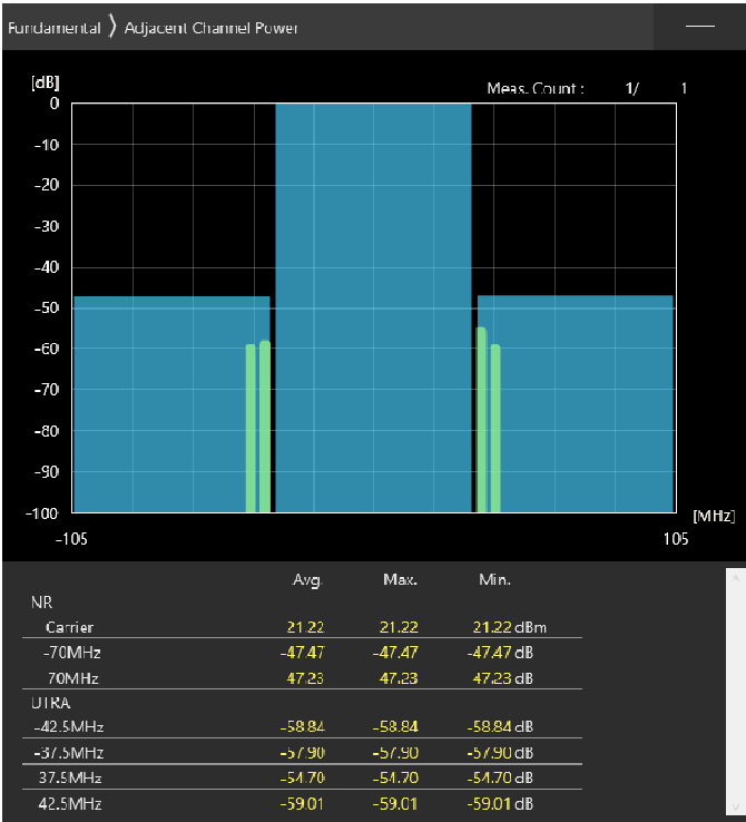
70MHz_30kHz_3665MHz-OFDM QPSK_RB1@188 -47.47,-47.23dB
