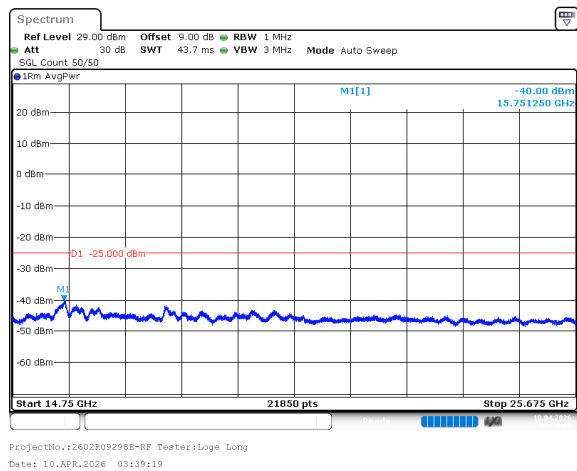
n7_5MHz_15kHz_2567.5MHz_DFT-s-OFDM QPSK_RB25@0 -40dBm
