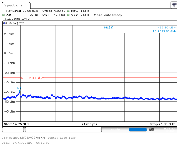
n7_10MHz_15kHz_2535MHz_DFT-s-OFDM QPSK_RB50@0 -39.60dBm
