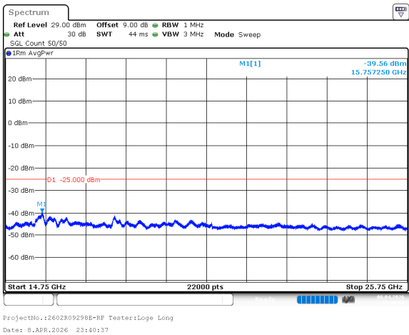
n38_10MHz_30kHz_2575MHz_DFT-s-OFDM QPSK_RB1@0 -39.56dBm
