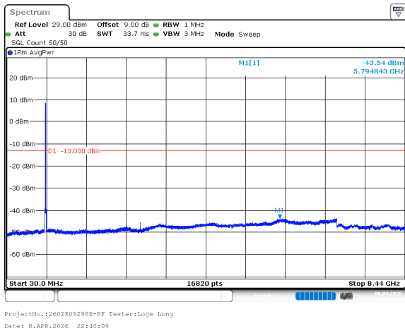
n5_10MHz_15kHz_844MHz_DFT-s-OFDM QPSK_RB50@0 -43.54dBm
