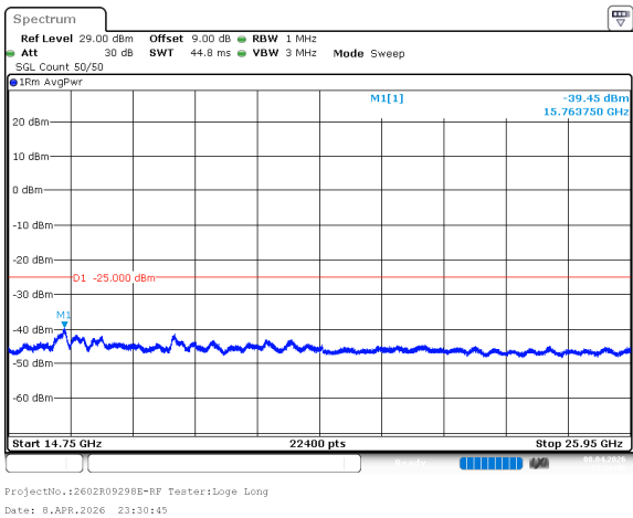
n38_5MHz_15kHz_2595MHz_DFT-s-OFDM QPSK_RB1@0 -39.45dBm
