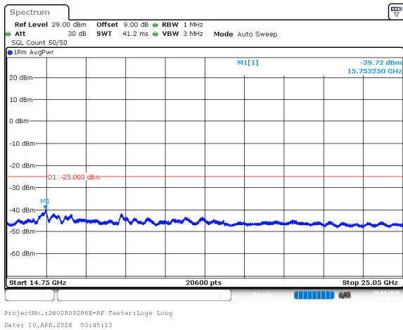
n7_10MHz_15kHz_2505MHz_DFT-s-OFDM QPSK_RB50@0 -39.72dBm
