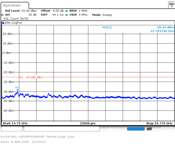
n38_15MHz_30kHz_2577.5MHz_DFT-s-OFDM QPSK_RB1@0 -39.44dBm
