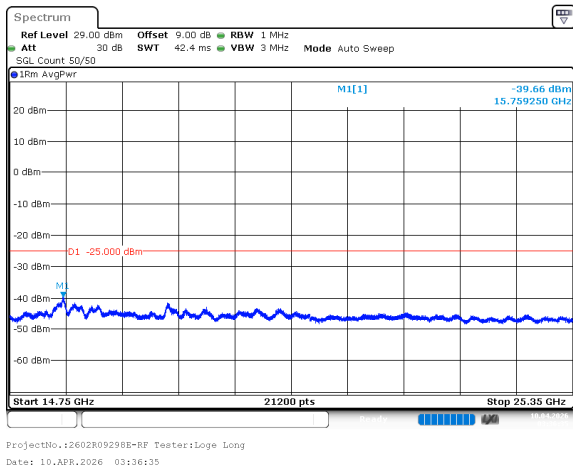
n7_5MHz_15kHz_2535MHz_DFT-s-OFDM QPSK_RB25@0 -39.66dBm
