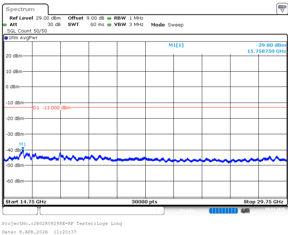
n77_3_70MHz_30kHz_3735MHz_DFT-s-OFDM QPSK_RB180@0 -39.80dBm
