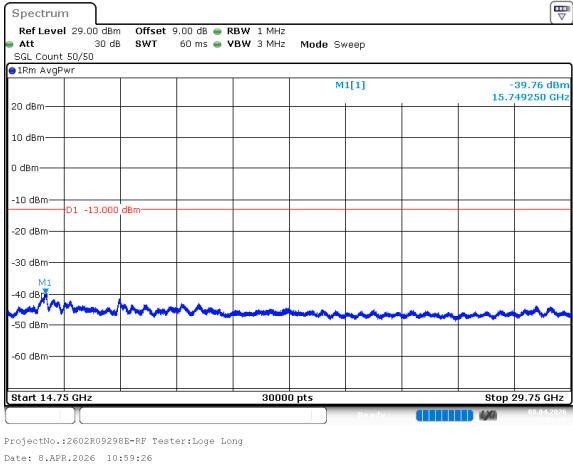
n77_3_50MHz_30kHz_3725MHz_DFT-s-OFDM QPSK_RB128@0 -39.76dBm
