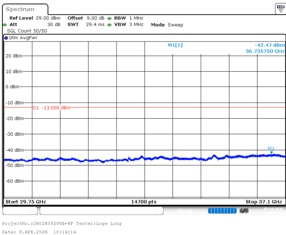
n77_3_20MHz_30kHz_3710MHz_DFT-s-OFDM QPSK_RB1@0 -42.47dBm
