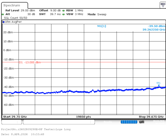
n77_3_25MHz_30kHz_3967.5MHz_DFT-s-OFDM QPSK_RB1@64 -39.50dBm
