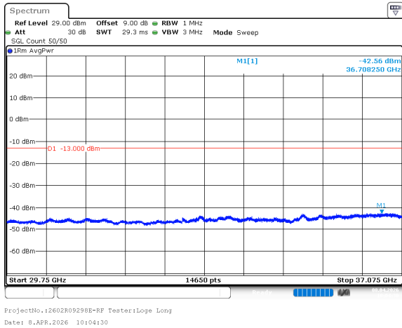
n77_3_15MHz_30kHz_3707.5MHz_DFT-s-OFDM QPSK_RB1@37 -42.56dBm
