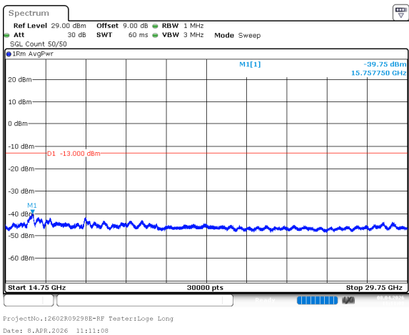
n77_3_60MHz_30kHz_3840MHz_DFT-s-OFDM QPSK_RB1@0 -39.75dBm
