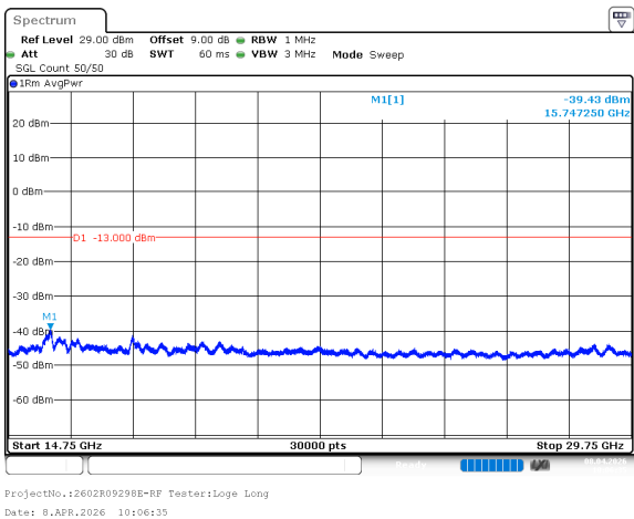
n77_3_15MHz_30kHz_3840MHz_DFT-s-OFDM QPSK_RB1@0 -39.43dBm
