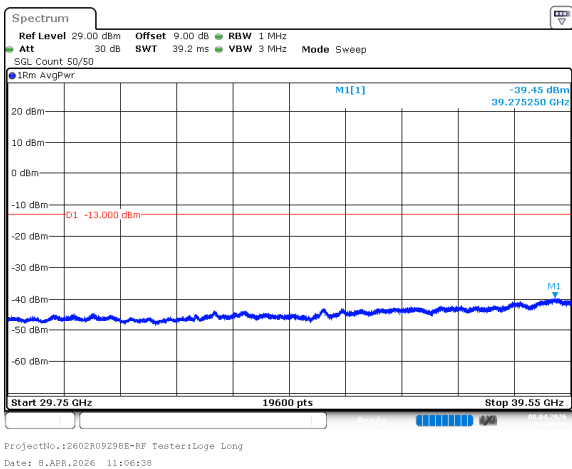
n77_3_50MHz_30kHz_3955MHz_DFT-s-OFDM QPSK_RB128@0 -39.45dBm
