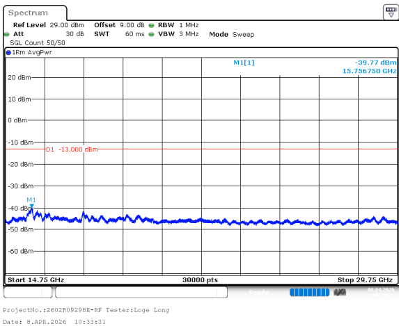
n77_3_25MHz_30kHz_3967.5MHz_DFT-s-OFDM QPSK_RB1@64 -39.77dBm
