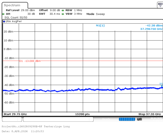
n77_3_70MHz_30kHz_3735MHz_DFT-s-OFDM QPSK_RB180@0 -42.38dBm
