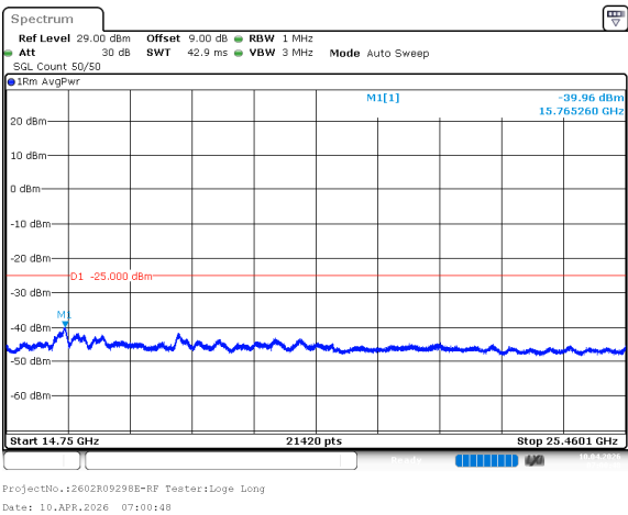
n41_100MHz_30kHz_2546.01MHz_DFT-s-OFDM QPSK_RB1@0 -39.96dBm
