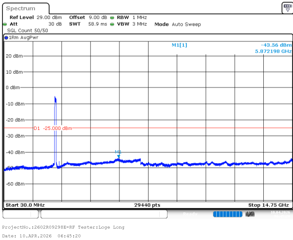
n41_90MHz_30kHz_2541MHz_DFT-s-OFDM QPSK_RB1@0 -43.60dBm
