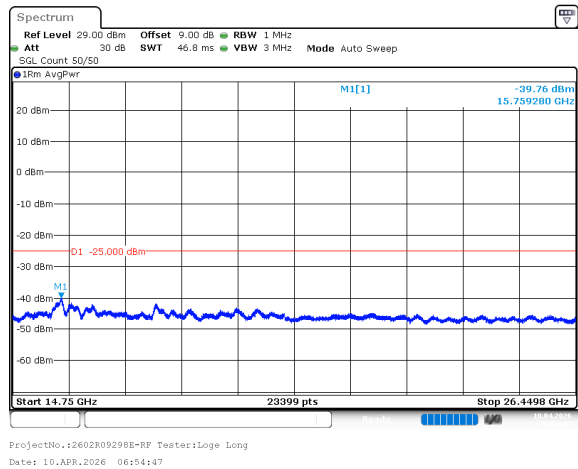
n41_90MHz_30kHz_2644.98MHz_DFT-s-OFDM QPSK_RB1@0 -39.76dBm
