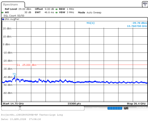
n41_100MHz_30kHz_2640MHz_DFT-s-OFDM QPSK_RB1@0 -39.78dBm
