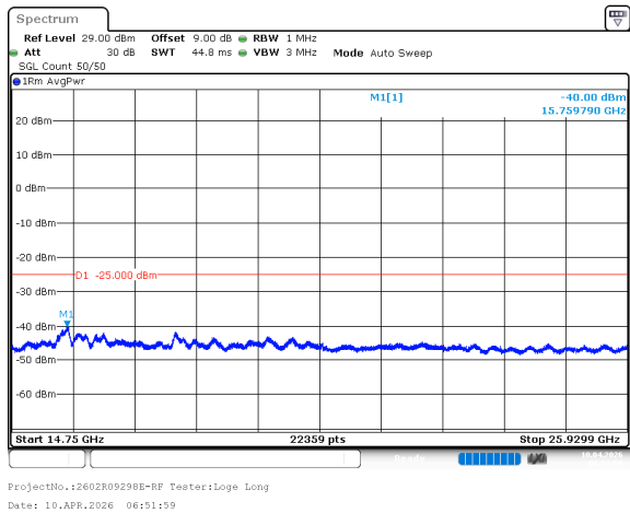
n41_90MHz_30kHz_2592.99MHz_DFT-s-OFDM QPSK_RB1@0 -40dBm
