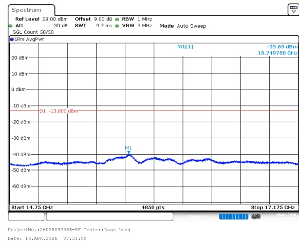
n66_15MHz_15kHz_1717.5MHz_DFT-s-OFDM QPSK_RB1@0 -39.69dBm
