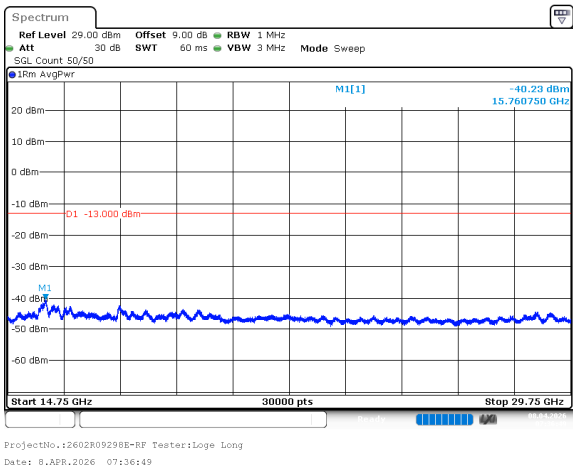
n77_1_20MHz_30kHz_3460MHz_DFT-s-OFDM QPSK_RB1@0 -40.23dBm
