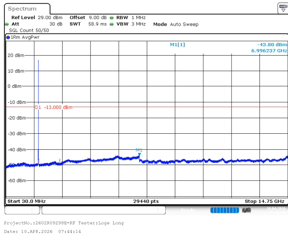
n66_20MHz_15kHz_1720MHz_DFT-s-OFDM QPSK_RB1@105 -43.80dBm
