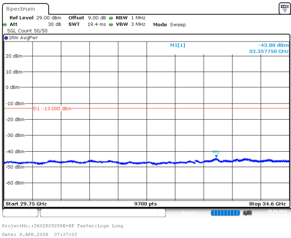
n77_1_20MHz_30kHz_3460MHz_DFT-s-OFDM QPSK_RB1@0 -43.88dBm
