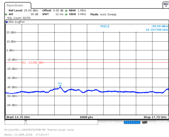
n66_10MHz_15kHz_1775MHz_DFT-s-OFDM QPSK_RB50@0 -40dBm
