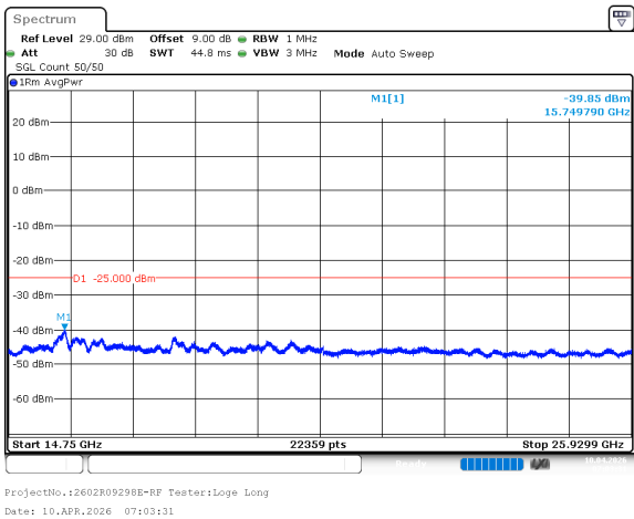
n41_100MHz_30kHz_2592.99MHz_DFT-s-OFDM QPSK_RB1@0 -39.85dBm
