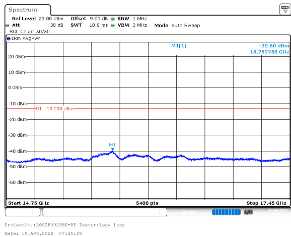
n66_20MHz_15kHz_1745MHz_DFT-s-OFDM QPSK_RB1@0 -39.60dBm
