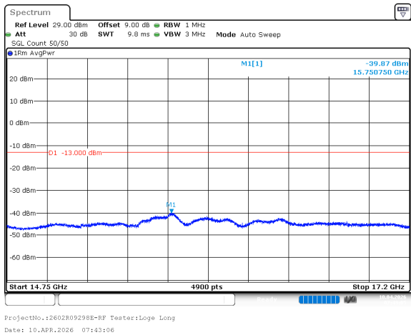
n66_20MHz_15kHz_1720MHz_DFT-s-OFDM QPSK_RB1@0 -39.87dBm
