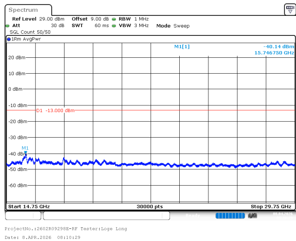
n77_1_40MHz_30kHz_3470MHz_DFT-s-OFDM QPSK_RB1@105 -40.14dBm
