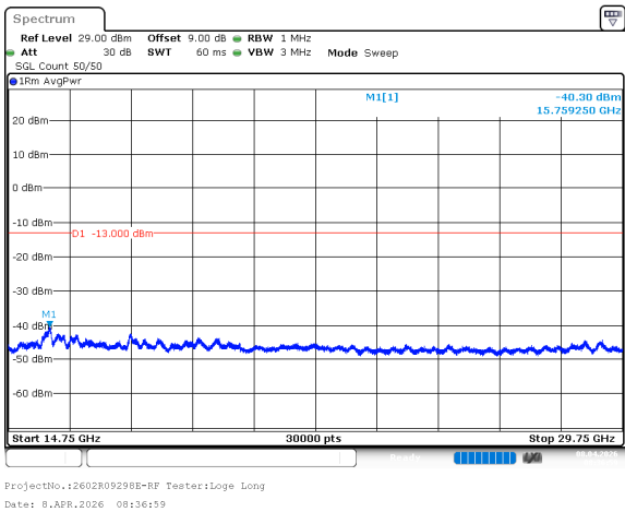
n77_1_60MHz_30kHz_3500MHz_DFT-s-OFDM QPSK_RB162@0 -40.30dBm
