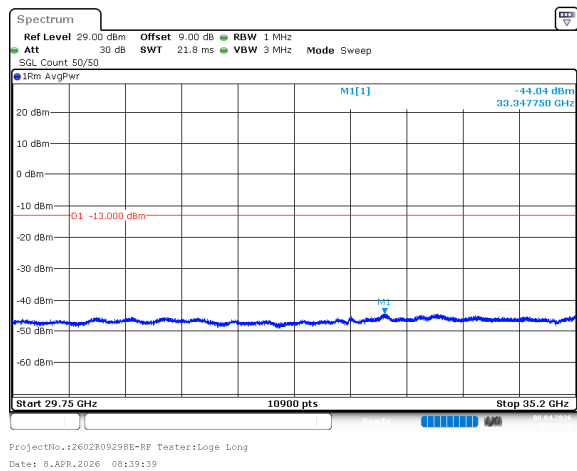
n77_1_60MHz_30kHz_3520MHz_DFT-s-OFDM QPSK_RB1@161 -44.04dBm
