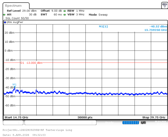
n77_1_60MHz_30kHz_3480MHz_DFT-s-OFDM QPSK_RB1@161 -40.52dBm
