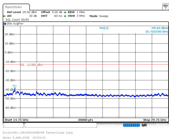
n77_3_10MHz_30kHz_3705MHz_DFT-s-OFDM QPSK_RB1@0 -39.63dBm
