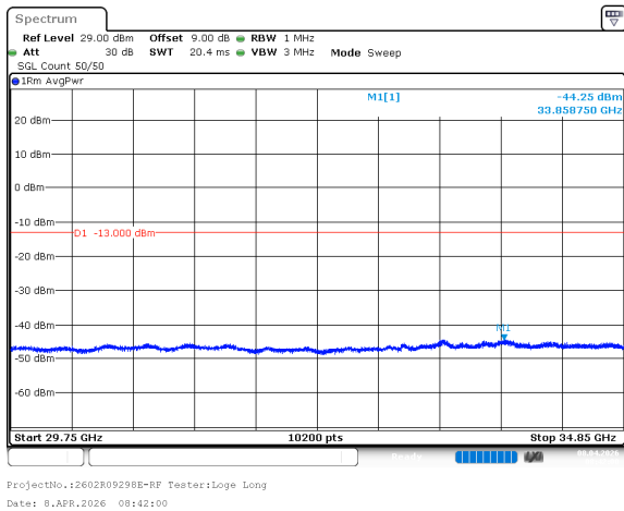
n77_1_70MHz_30kHz_3485MHz_DFT-s-OFDM QPSK_RB1@0 -44.25dBm
