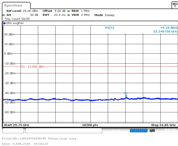
n77_1_70MHz_30kHz_3485MHz_DFT-s-OFDM QPSK_RB180@0 -44.19dBm
