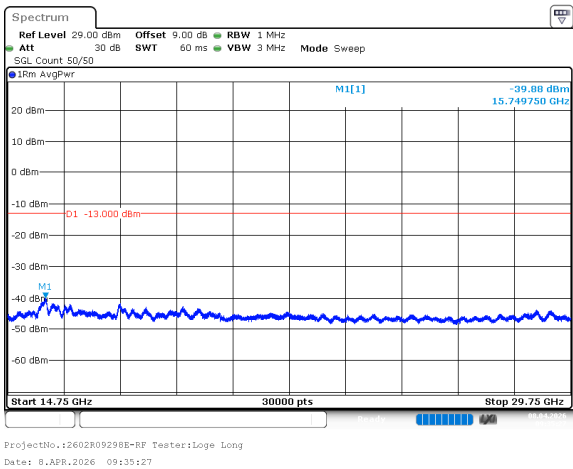
n77_1_90MHz_30kHz_3505MHz_DFT-s-OFDM QPSK_RB1@0 -39.88dBm
