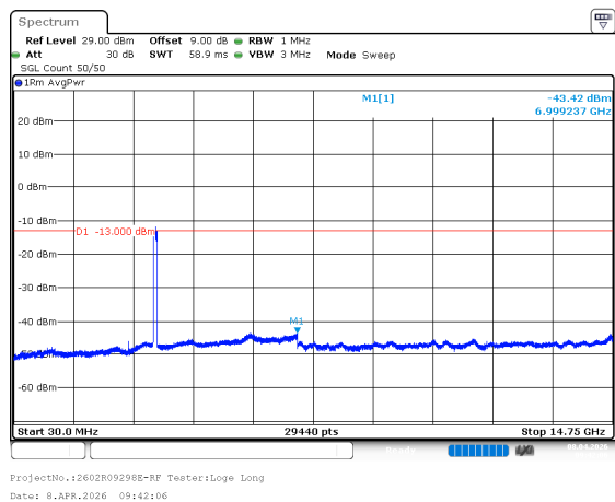
n77_1_100MHz_30kHz_3500MHz_DFT-s-OFDM QPSK_RB270@0 -43.42dBm
