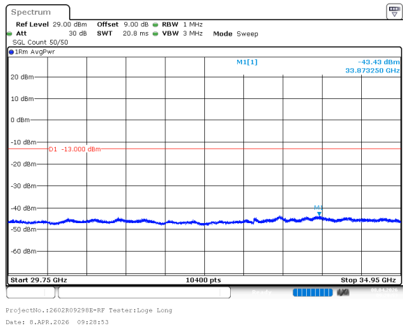
n77_1_90MHz_30kHz_3495MHz_DFT-s-OFDM QPSK_RB1@0 -43.43dBm
