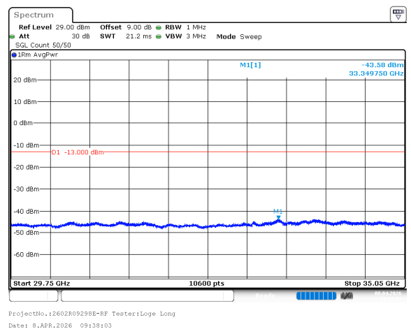
n77_1_90MHz_30kHz_3505MHz_DFT-s-OFDM QPSK_RB243@0 -43.58dBm
