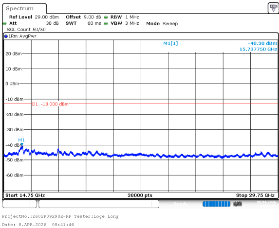
n77_1_70MHz_30kHz_3485MHz_DFT-s-OFDM QPSK_RB1@0 -40.30dBm
