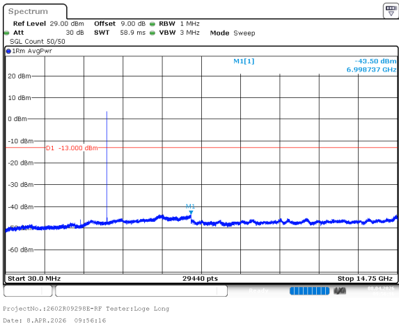
n77_3_10MHz_30kHz_3840MHz_DFT-s-OFDM QPSK_RB1@0 -41.67dBm
