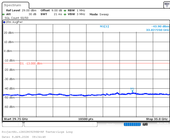
n77_1_60MHz_30kHz_3500MHz_DFT-s-OFDM QPSK_RB1@0 -43.90dBm
