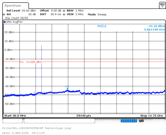
n77_1_40MHz_30kHz_3470MHz_DFT-s-OFDM QPSK_RB1@105 -44dBm
