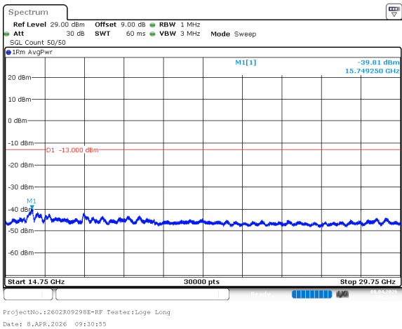
n77_1_90MHz_30kHz_3495MHz_DFT-s-OFDM QPSK_RB243@0 -39.81dBm
