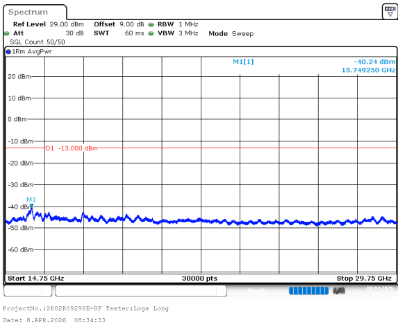
n77_1_60MHz_30kHz_3500MHz_DFT-s-OFDM QPSK_RB1@0 -40.24dBm
