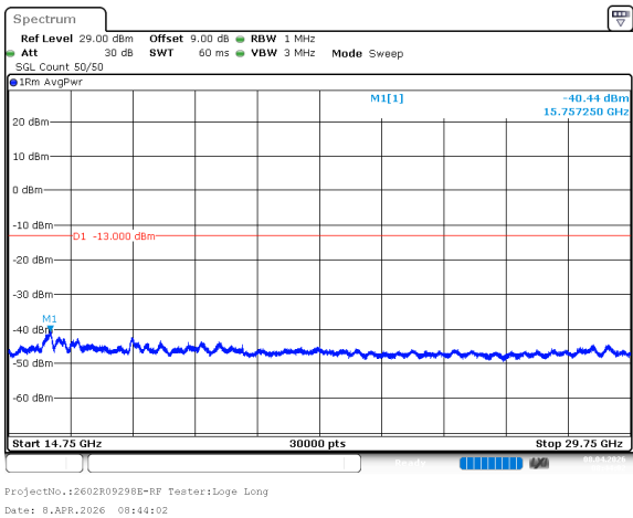
n77_1_70MHz_30kHz_3485MHz_DFT-s-OFDM QPSK_RB180@0 -40.44dBm
