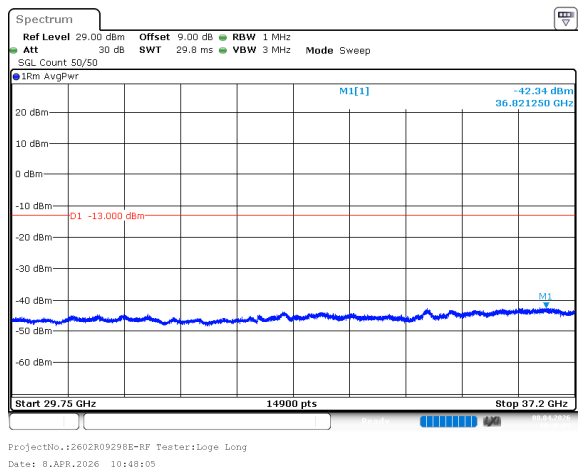
n77_3_40MHz_30kHz_3720MHz_DFT-s-OFDM QPSK_RB1@105 -42.34dBm
