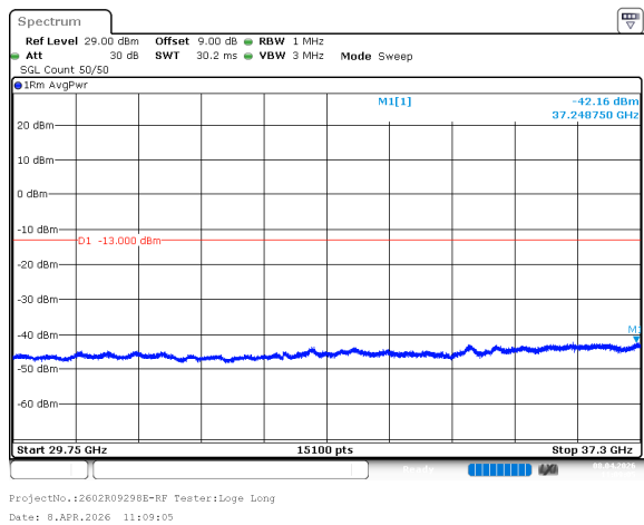
n77_3_60MHz_30kHz_3730MHz_DFT-s-OFDM QPSK_RB1@161 -42.16dBm
