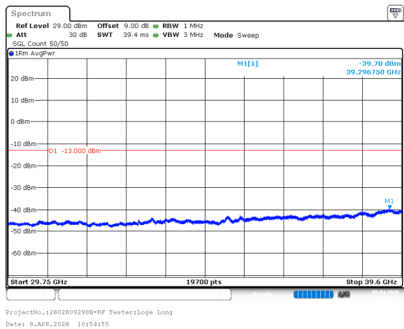
n77_3_40MHz_30kHz_3960MHz_DFT-s-OFDM QPSK_RB1@105 -39.70dBm
