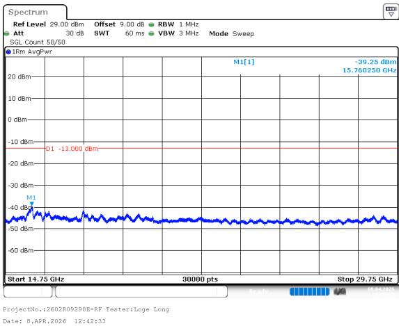
n78_1_30MHz_30kHz_3465MHz_DFT-s-OFDM QPSK_RB1@0 -39.25dBm
