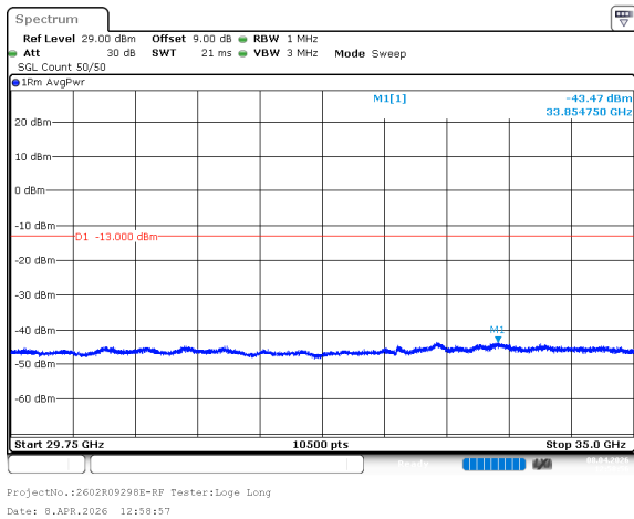
n78_1_40MHz_30kHz_3500MHz_DFT-s-OFDM QPSK_RB100@0 -43.47dBm
