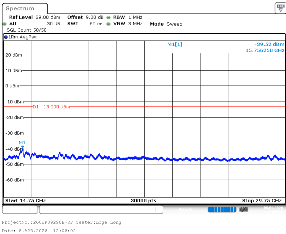
n78_1_10MHz_30kHz_3500MHz_DFT-s-OFDM QPSK_RB1@23 -39.52dBm
