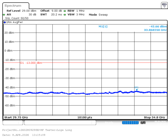
n78_1_60MHz_30kHz_3480MHz_DFT-s-OFDM QPSK_RB1@161 -43.66dBm
