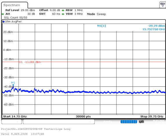
n78_1_50MHz_30kHz_3500MHz_DFT-s-OFDM QPSK_RB1@132 -39.29dBm
