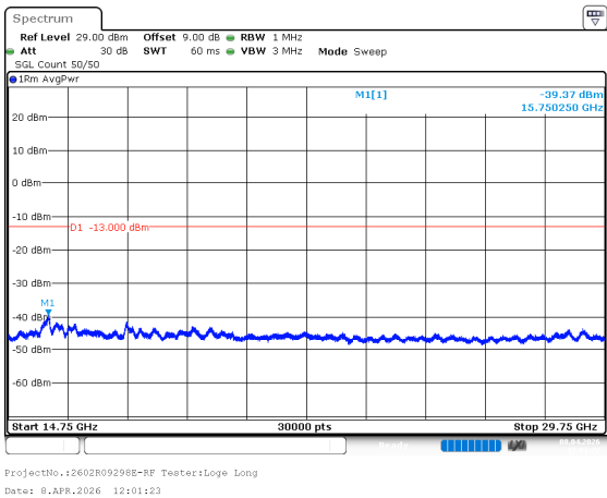
n78_1_10MHz_30kHz_3455MHz_DFT-s-OFDM QPSK_RB1@0 -39.37dBm
