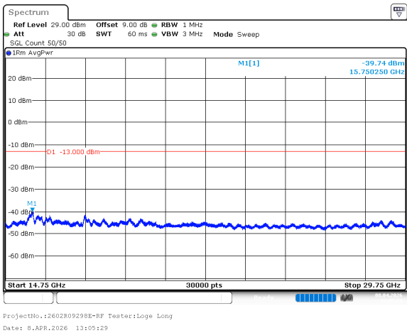
n78_1_50MHz_30kHz_3475MHz_DFT-s-OFDM QPSK_RB128@0 -39.74dBm
