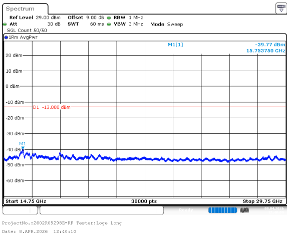
n78_1_25MHz_30kHz_3537.5MHz_DFT-s-OFDM QPSK_RB1@64 -39.77dBm
