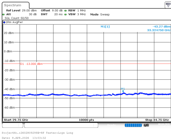
n78_1_50MHz_30kHz_3475MHz_DFT-s-OFDM QPSK_RB1@0 -43.27dBm
