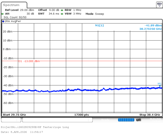
n77_3_100MHz_30kHz_3840MHz_DFT-s-OFDM QPSK_RB270@0 -41.89dBm
