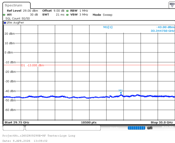
n78_1_50MHz_30kHz_3500MHz_DFT-s-OFDM QPSK_RB1@132 -43dBm
