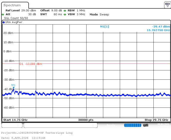
n78_1_15MHz_30kHz_3542.5MHz_DFT-s-OFDM QPSK_RB1@37 -39.47dBm
