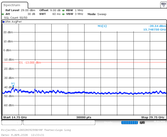
n78_1_25MHz_30kHz_3462.5MHz_DFT-s-OFDM QPSK_RB1@64 -39.54dBm
