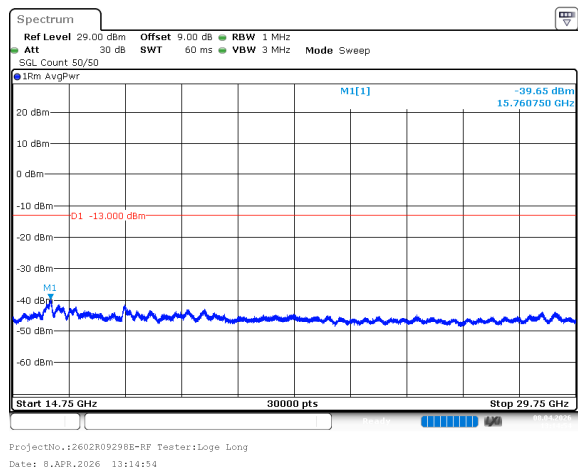
n78_1_60MHz_30kHz_3480MHz_DFT-s-OFDM QPSK_RB1@161 -39.65dBm
