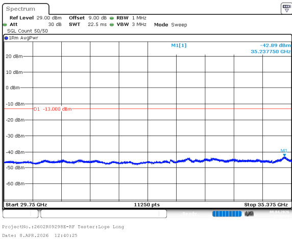
n78_1_25MHz_30kHz_3537.5MHz_DFT-s-OFDM QPSK_RB1@64 -42.89dBm
