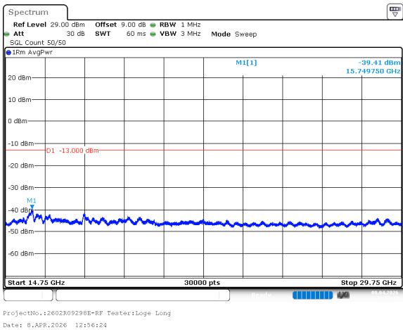
n78_1_40MHz_30kHz_3500MHz_DFT-s-OFDM QPSK_RB1@0 -39.41dBm
