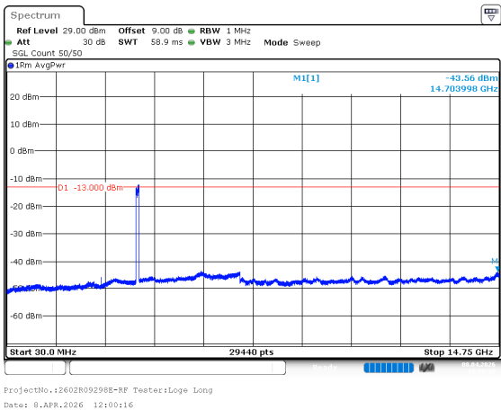
n77_3_100MHz_30kHz_3930MHz_DFT-s-OFDM QPSK_RB270@0 -43.56dBm
