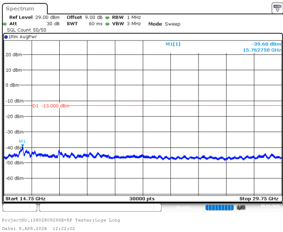
n78_1_20MHz_30kHz_3460MHz_DFT-s-OFDM QPSK_RB1@0 -39.68dBm
