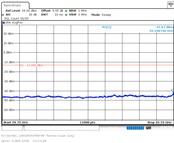
n78_1_50MHz_30kHz_3525MHz_DFT-s-OFDM QPSK_RB128@0 -42.67dBm
