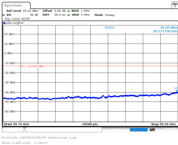
n77_3_90MHz_30kHz_3935MHz_DFT-s-OFDM QPSK_RB1@0 -39.60dBm
