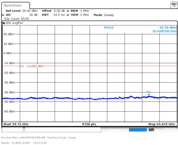
n78_1_25MHz_30kHz_3462.5MHz_DFT-s-OFDM QPSK_RB1@64 -43.39dBm
