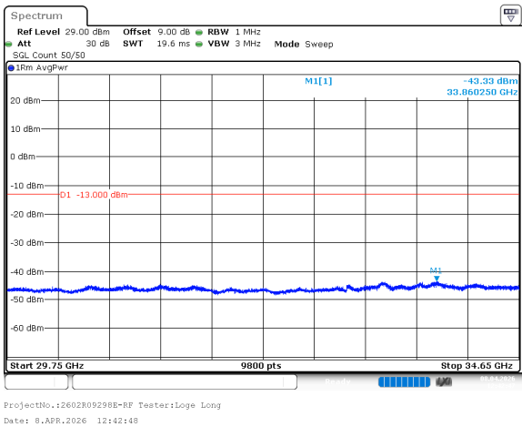
n78_1_30MHz_30kHz_3465MHz_DFT-s-OFDM QPSK_RB1@0 -43.33dBm
