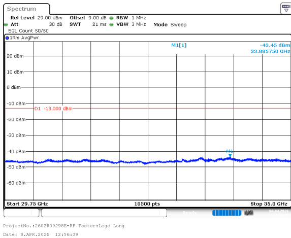
n78_1_40MHz_30kHz_3500MHz_DFT-s-OFDM QPSK_RB1@0 -43.45dBm
