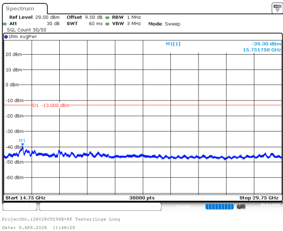
n77_3_90MHz_30kHz_3935MHz_DFT-s-OFDM QPSK_RB1@0 -39.30dBm
