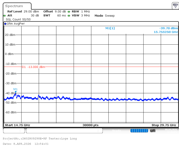
n78_1_40MHz_30kHz_3470MHz_DFT-s-OFDM QPSK_RB1@105 -39.70dBm
