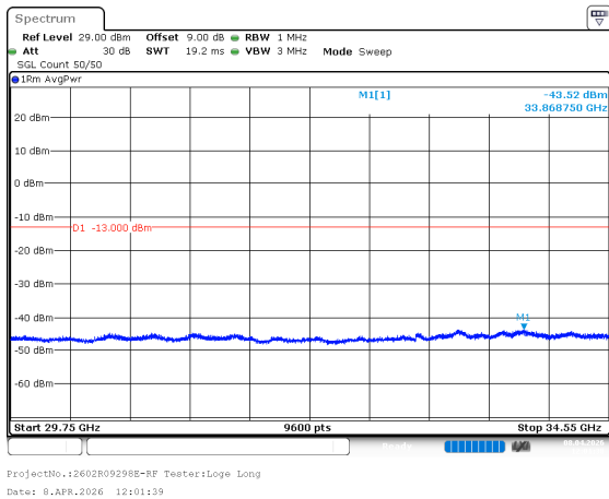
n78_1_10MHz_30kHz_3455MHz_DFT-s-OFDM QPSK_RB1@0 -43.52dBm
