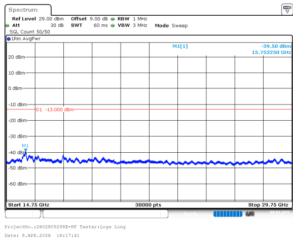
n78_3_80MHz_30kHz_3760MHz_DFT-s-OFDM QPSK_RB1@216 -39.50dBm
