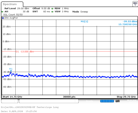
n78_3_50MHz_30kHz_3725MHz_DFT-s-OFDM QPSK_RB1@0 -39.53dBm
