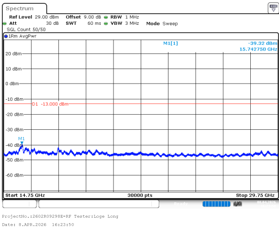
n78_3_90MHz_30kHz_3745MHz_DFT-s-OFDM QPSK_RB1@0 -39.32dBm
