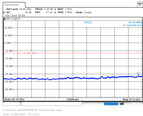
n78_3_40MHz_30kHz_3750MHz_DFT-s-OFDM QPSK_RB1@0 -42.20dBm
