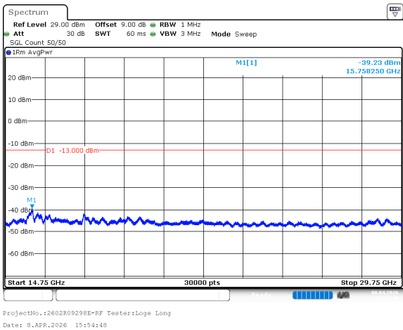
n78_3_70MHz_30kHz_3735MHz_DFT-s-OFDM QPSK_RB1@0 -39.23dBm
