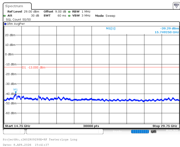
n78_3_60MHz_30kHz_3730MHz_DFT-s-OFDM QPSK_RB1@161 -39.29dBm
