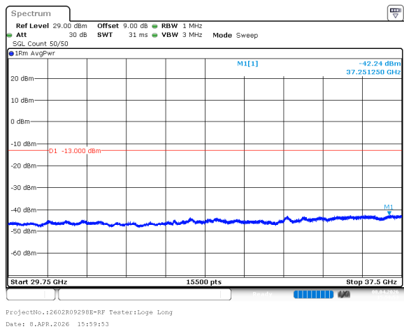
n78_3_70MHz_30kHz_3750MHz_DFT-s-OFDM QPSK_RB1@188 -42.24dBm
