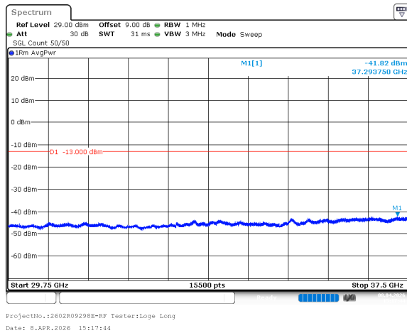
n78_3_40MHz_30kHz_3750MHz_DFT-s-OFDM QPSK_RB100@0 -41.82dBm
