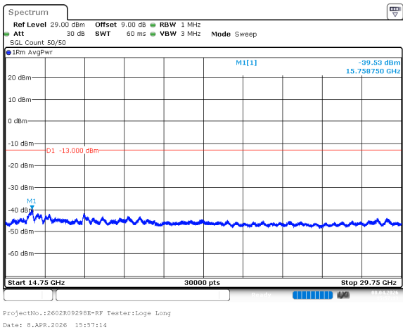
n78_3_70MHz_30kHz_3735MHz_DFT-s-OFDM QPSK_RB180@0 -39.53dBm
