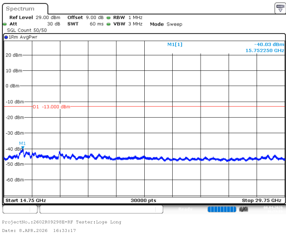
n78_3_90MHz_30kHz_3755MHz_DFT-s-OFDM QPSK_RB243@0 -40.03dBm
