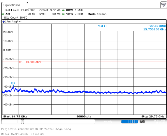
n78_3_50MHz_30kHz_3775MHz_DFT-s-OFDM QPSK_RB128@0 -39.63dBm
