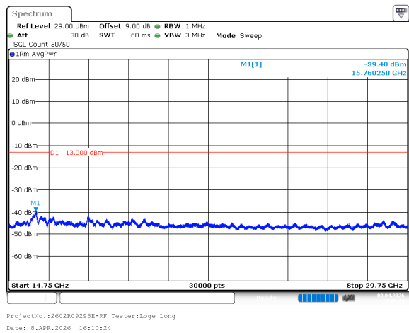
n78_3_80MHz_30kHz_3740MHz_DFT-s-OFDM QPSK_RB1@216 -39.40dBm
