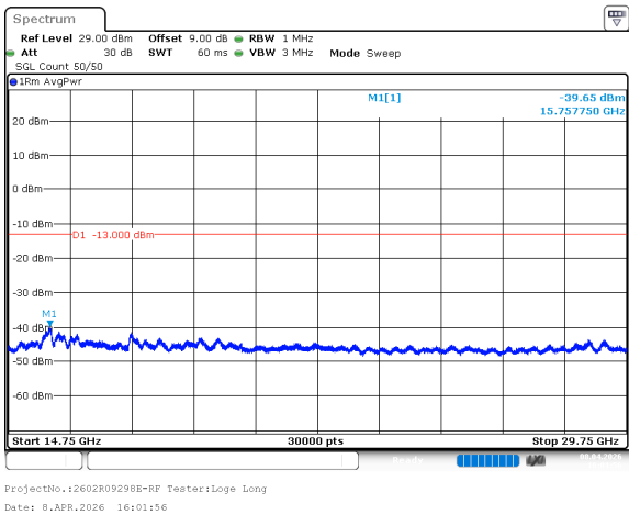
n78_3_70MHz_30kHz_3765MHz_DFT-s-OFDM QPSK_RB1@0 -39.65dBm
