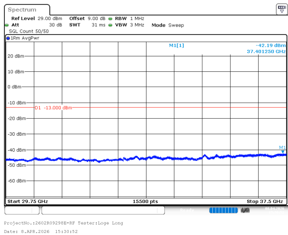
n78_3_50MHz_30kHz_3750MHz_DFT-s-OFDM QPSK_RB1@132 -42.19dBm
