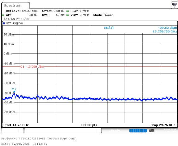
n78_3_60MHz_30kHz_3750MHz_DFT-s-OFDM QPSK_RB1@0 -39.63dBm
