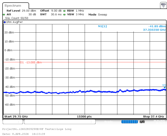
n78_3_80MHz_30kHz_3740MHz_DFT-s-OFDM QPSK_RB1@216 -41.85dBm
