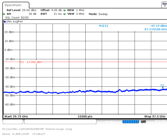
n78_3_60MHz_30kHz_3750MHz_DFT-s-OFDM QPSK_RB162@0 -42.12dBm
