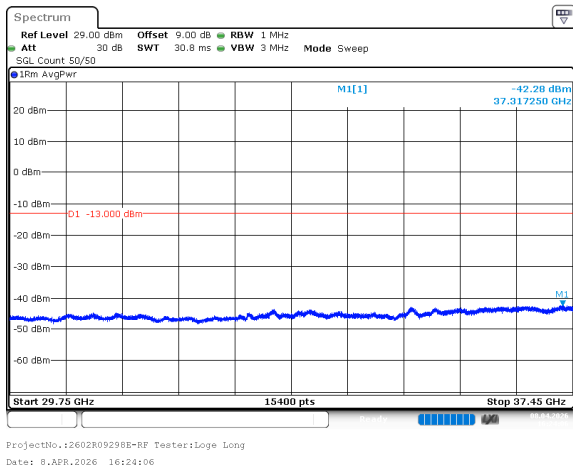
n78_3_90MHz_30kHz_3745MHz_DFT-s-OFDM QPSK_RB1@0 -42.28dBm
