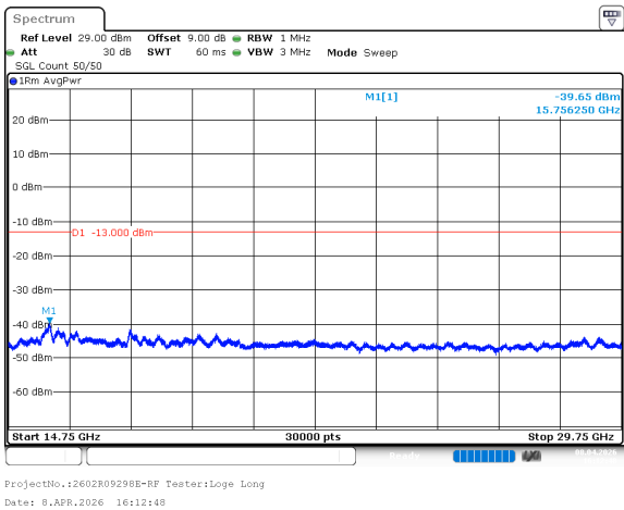
n78_3_80MHz_30kHz_3750MHz_DFT-s-OFDM QPSK_RB1@0 -39.65dBm
