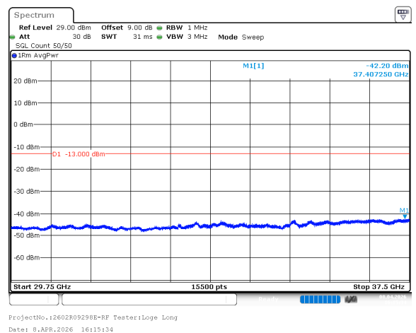
n78_3_80MHz_30kHz_3750MHz_DFT-s-OFDM QPSK_RB216@0 -42.20dBm
