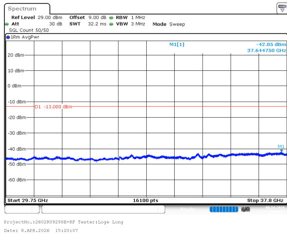
n78_3_40MHz_30kHz_3780MHz_DFT-s-OFDM QPSK_RB1@105 -42.05dBm
