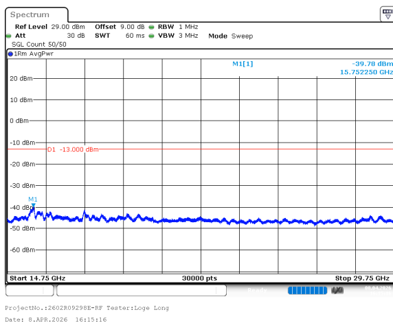
n78_3_80MHz_30kHz_3750MHz_DFT-s-OFDM QPSK_RB216@0 -39.78dBm
