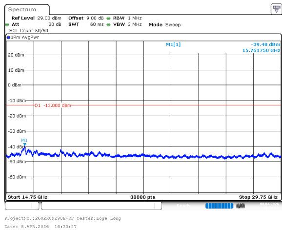
n78_3_90MHz_30kHz_3755MHz_DFT-s-OFDM QPSK_RB1@0 -39.48dBm
