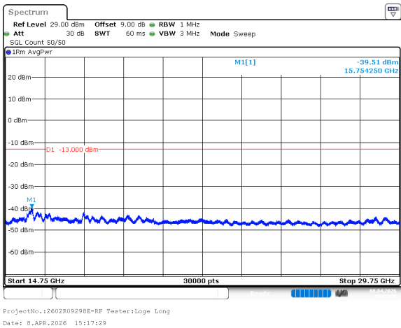
n78_3_40MHz_30kHz_3750MHz_DFT-s-OFDM QPSK_RB100@0 -39.51dBm
