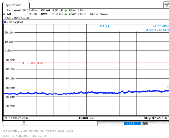
n78_3_90MHz_30kHz_3745MHz_DFT-s-OFDM QPSK_RB243@0 -42.30dBm
