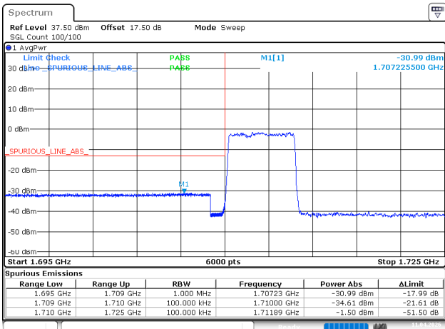
5MHz_Low_QPSK_25@0
