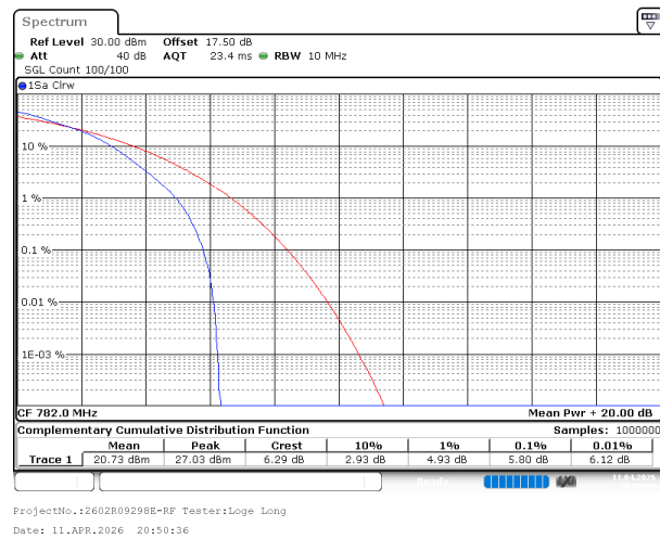
10MHz_Middle_16QAM_50@0
