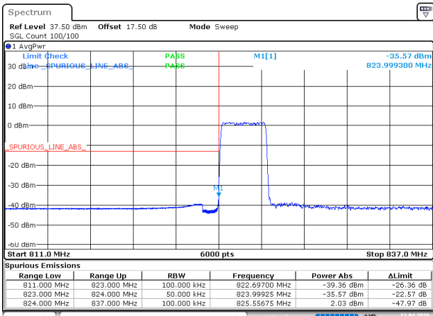
3MHz_Low_16QAM_15@0
