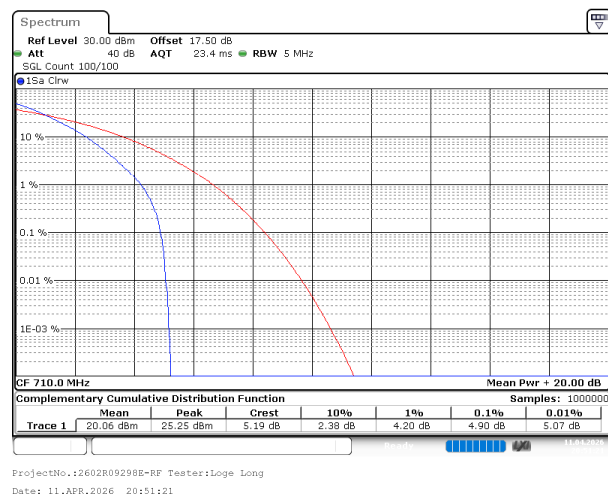
5MHz_Middle_QPSK_25@0
