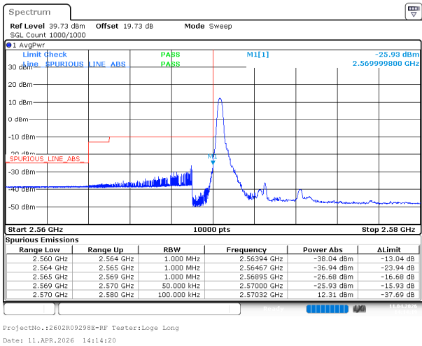
5MHz_Low_QPSK_1@0
