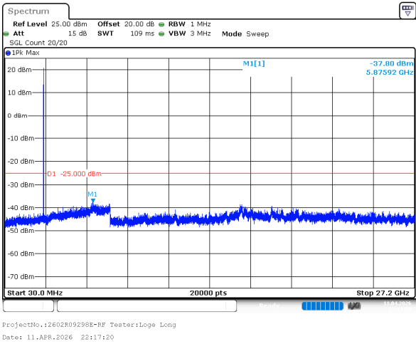
10MHz_Low_QPSK_1@0(30MHz~27.2GHz)
