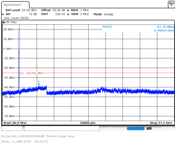
10MHz_Middle_QPSK_1@0(30MHz~27.2GHz)
