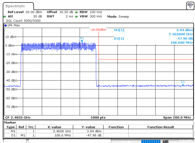
3EDR_DH1_Hopping_Upper
