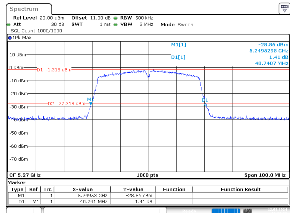
n40_5270MHz_Chain 0
