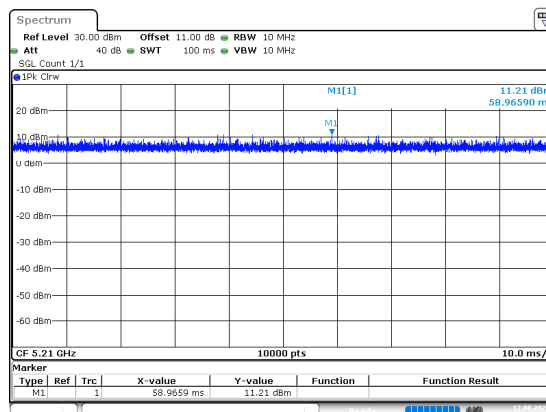
ac80_5210MHz_Chain 0
