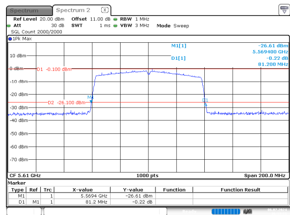
ac80_5610MHz_Chain 0
