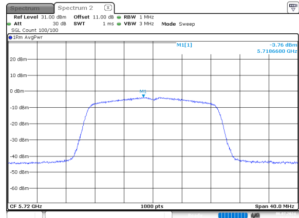
n20_5720MHz_Chain 0
