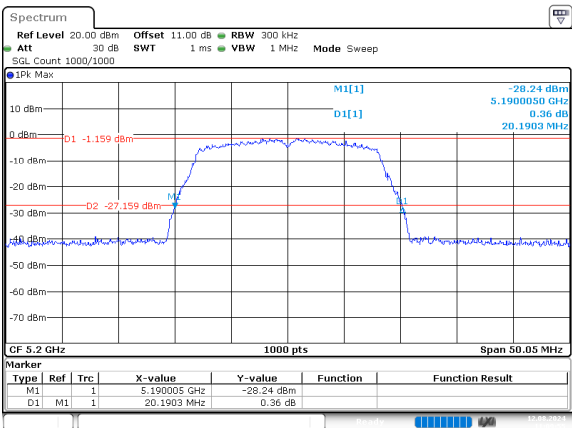
a_5200MHz_Chain 0
