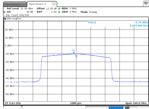
ac80_5610MHz_Chain 0
