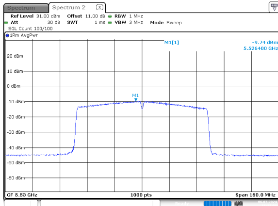
ac80_5530MHz_Chain 0
