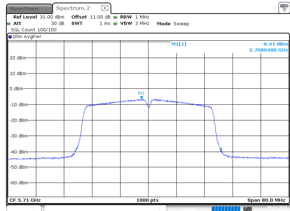
n40_5710MHz_Chain 0
