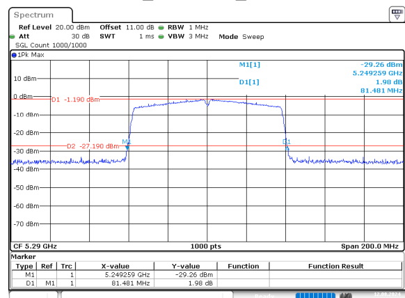
ac80_5290MHz_Chain 0
