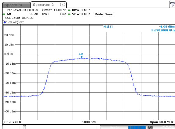
n20_5700MHz_Chain 0
