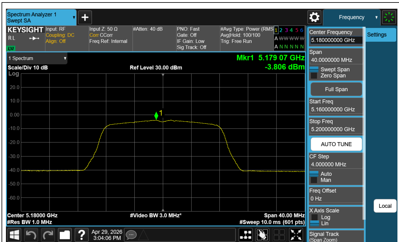
802.11a OFDM 5180MHz
