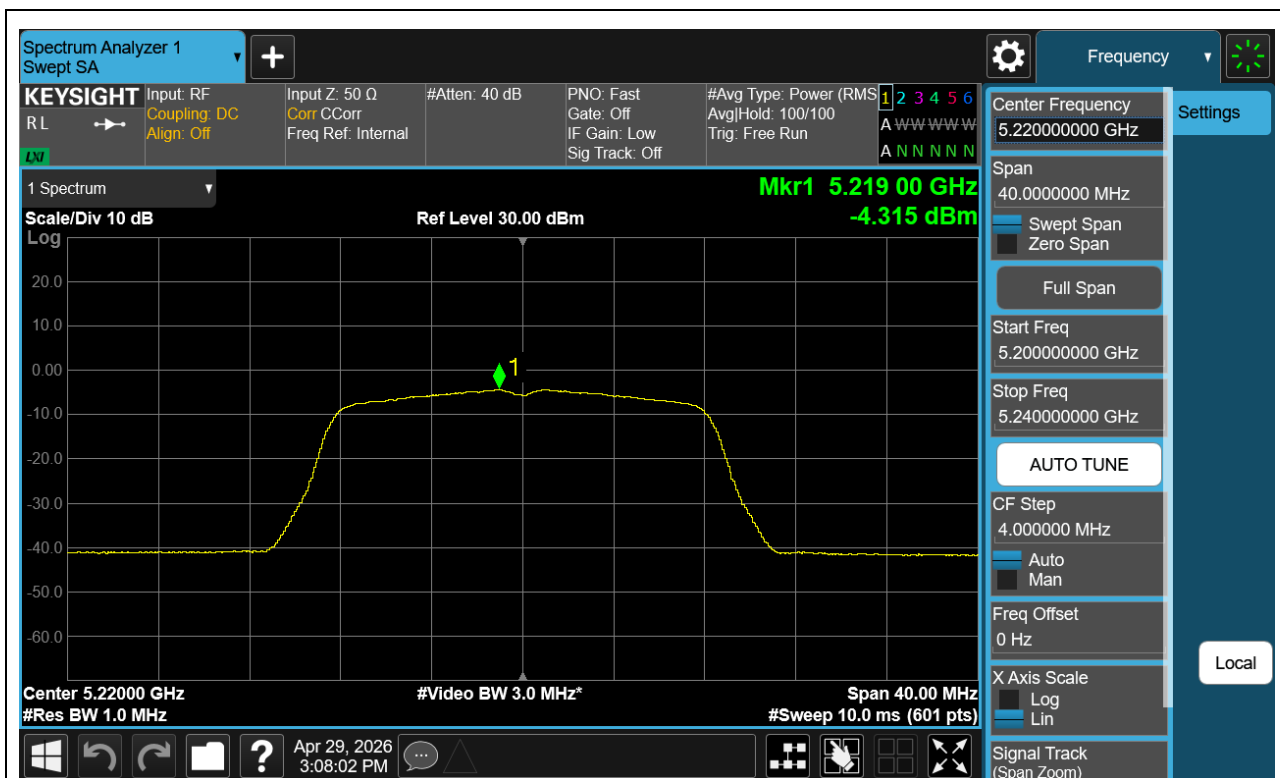
802.11a OFDM 5220MHz
