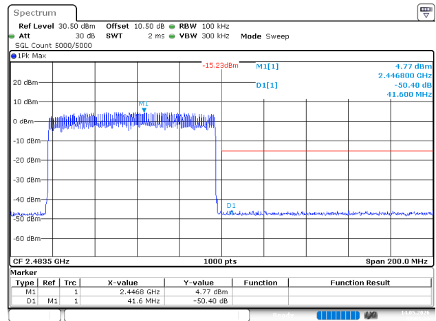
2EDR_DH1_Hopping_Upper
