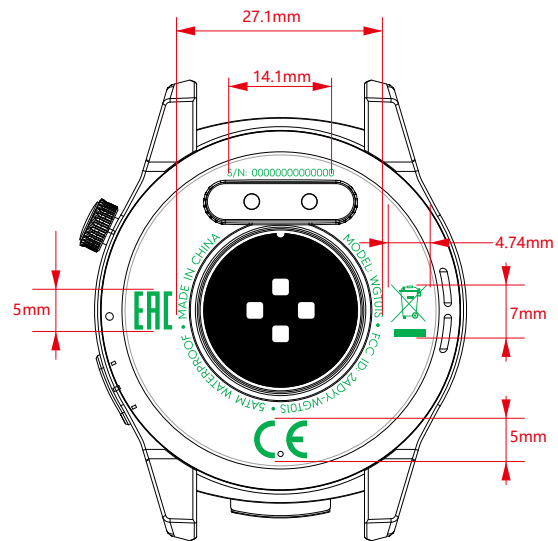
镭雕位置及尺寸
