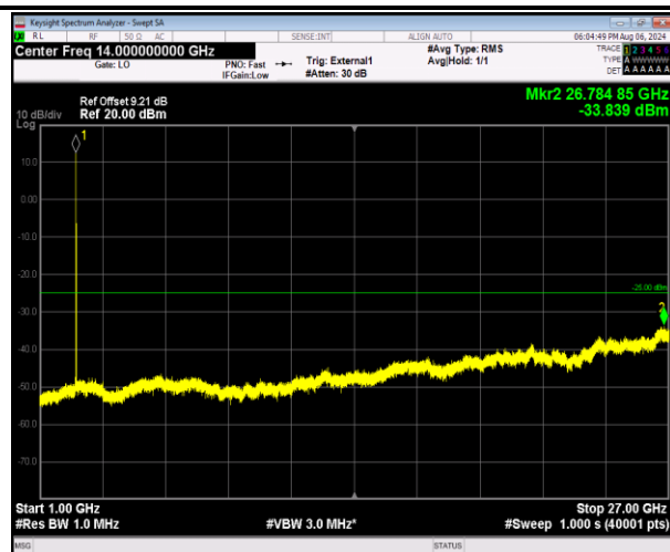
41-41-20MHz-5MHz-QPSK-QPSK-39750-39867-1RB#0-1RB#24-1000~27000MHz-PASS
