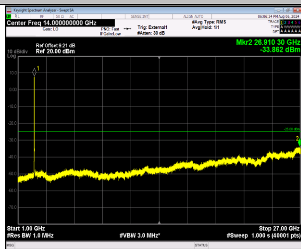
41-41-20MHz-5MHz-QPSK-QPSK-39750-39867-100RB#0-25RB#0-1000~27000MHz-PASS
