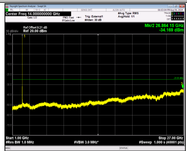
41-41-20MHz-5MHz-QPSK-QPSK-39750-39867-1RB#99-0 RB#0-1000~27000MHz-PASS
