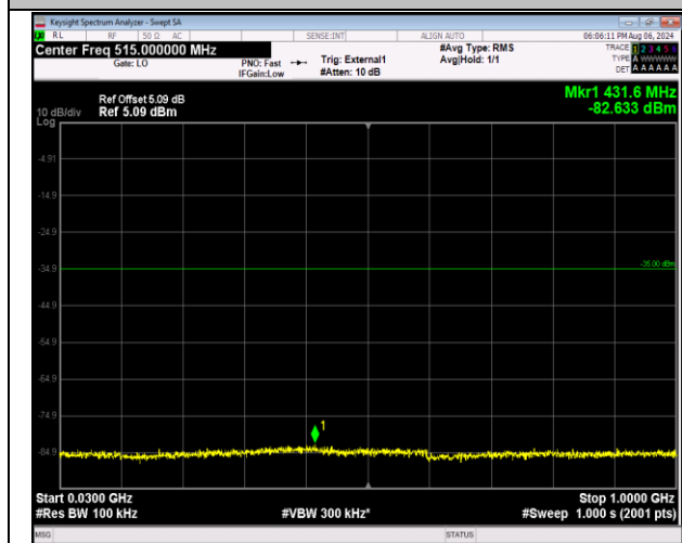
41-41-20MHz-5MHz-QPSK-QPSK-39750-39867-100RB#0-25RB#0-30~1000MHz-PASS
