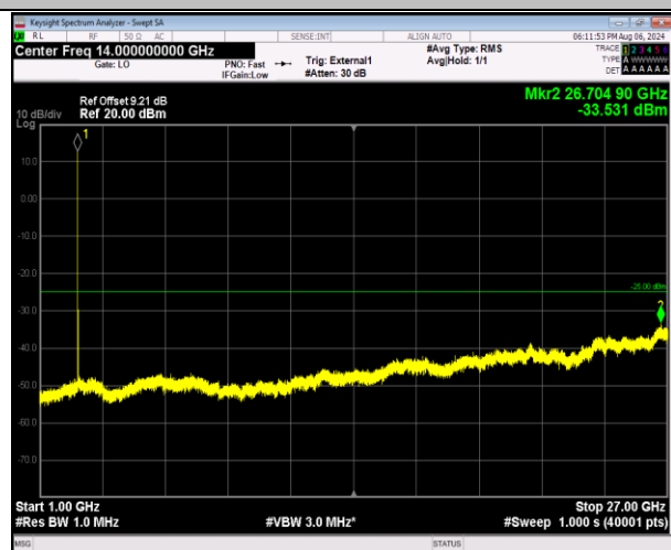
41-41-20MHz-5MHz-QPSK-QPSK-40595-40712-1RB#0-1RB#24-1000~27000MHz-PASS
