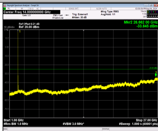
41-41-5MHz-20MHz-QPSK-QPSK-39683-39800-1RB#0-0R B#0-1000~27000MHz-PASS
