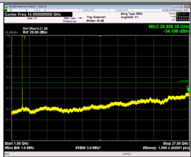
41-41-20MHz-5MHz-QPSK-QPSK-40595-40712-1RB#0-0RB#0-1000~27000MHz-PASS
