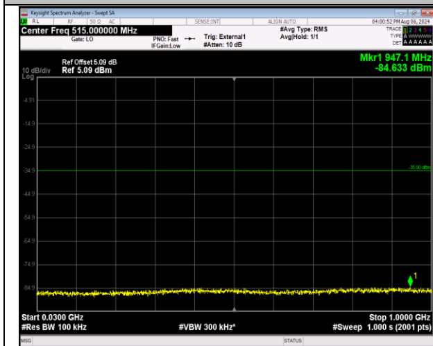
41-41-5MHz-20MHz-QPSK-QPSK-40528-40645-1RB#0- 1RB#99-30~1000MHz-PASS
