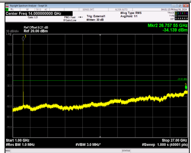
41-41-5MHz-20MHz-QPSK-QPSK-40528-40645-1RB#0-1R B#99-1000~27000MHz-PASS
