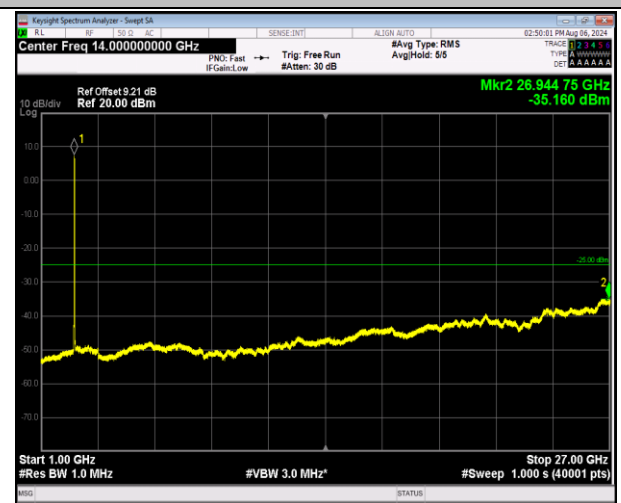
7-7-20MHz-20MHz-QPSK-QPSK-21001-21199-100RB#0-1 00RB#0-1000~27000MHz-PASS
