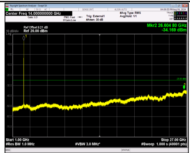
41-41-5MHz-20MHz-QPSK-QPSK-41373-41490-25RB#0-1 00RB#0-1000~27000MHz-PASS
