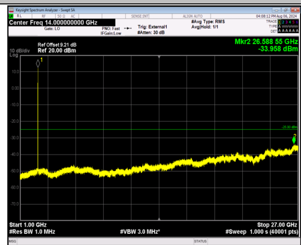
41-41-5MHz-20MHz-QPSK-QPSK-41373-41490-1RB#0-1RB#99-1000~27000MHz-PASS
