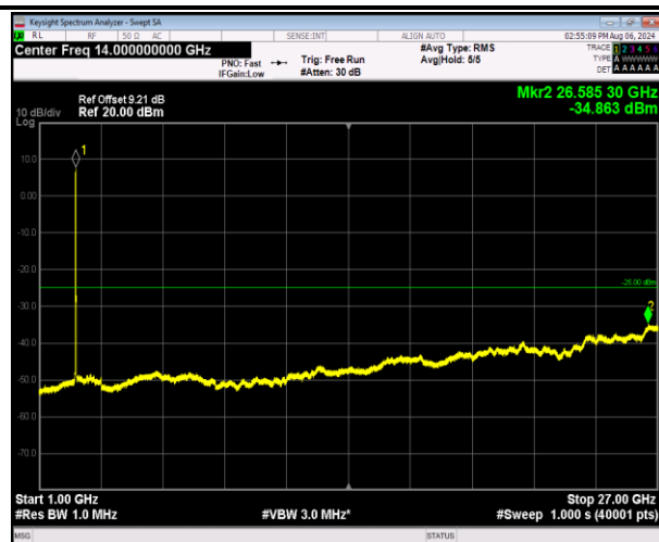
7-7-20MHz-20MHz-QPSK-QPSK-21152-21350-100RB#0-1 00RB#0-1000~27000MHz-PASS
