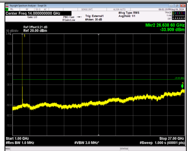
41-41-20MHz-5MHz-QPSK-QPSK-39750-39867-1RB#0-0R B#0-1000~27000MHz-PASS
