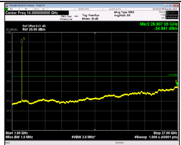
7-7-20MHz-10MHz-QPSK-QPSK-21251-21395-100RB#0-5 ORB#0-1000~27000MHz-PASS
