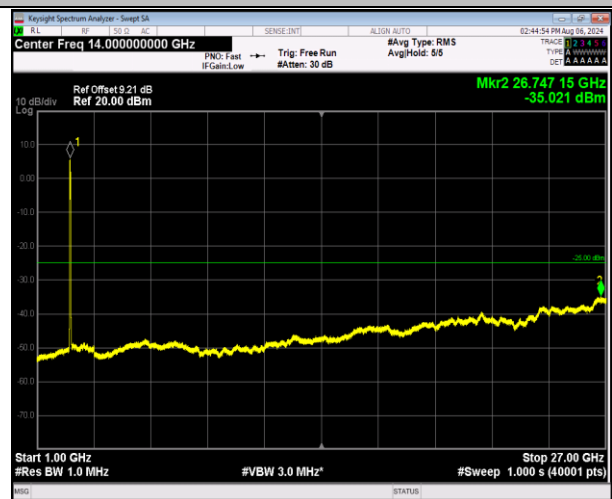
7-7-20MHz-20MHz-QPSK-QPSK-20850-21048-100RB#0-100RB#0-1000~27000MHz-PASS
