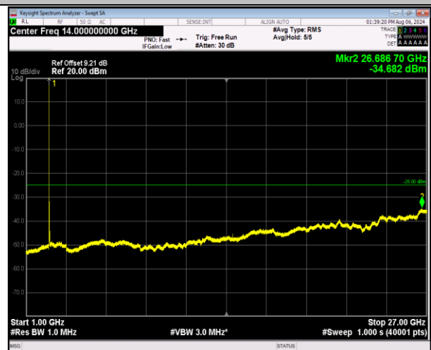
7-7-20MHz-10MHz-QPSK-QPSK-20850-20994-1RB#0-0-1000~27000MHz-PASS
