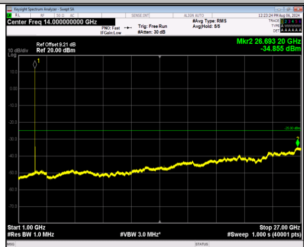
7-7-10MHz-20MHz-QPSK-QPSK-21006-21150-1RB#0-1RB#99-1000~27000MHz-PASS
