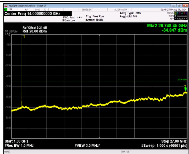
7-7-20MHz-10MHz-QPSK-QPSK-21251-21395-1RB#0-0RB #0-1000~27000MHz-PASS
