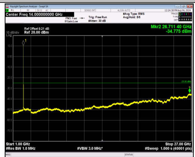
7-7-10MHz-20MHz-QPSK-QPSK-21006-21150-50RB#0-100RB#0-1000~27000MHz-PASS
