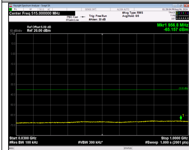
7-7-20MHz-10MHz-QPSK-QPSK-20850-20994-1RB#0-0-30~1000MHz-PASS
