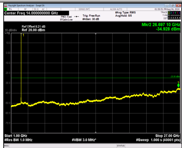
7-7-20MHz-10MHz-QPSK-QPSK-21251-21395-1RB#99-0R B#0-1000~27000MHz-PASS
