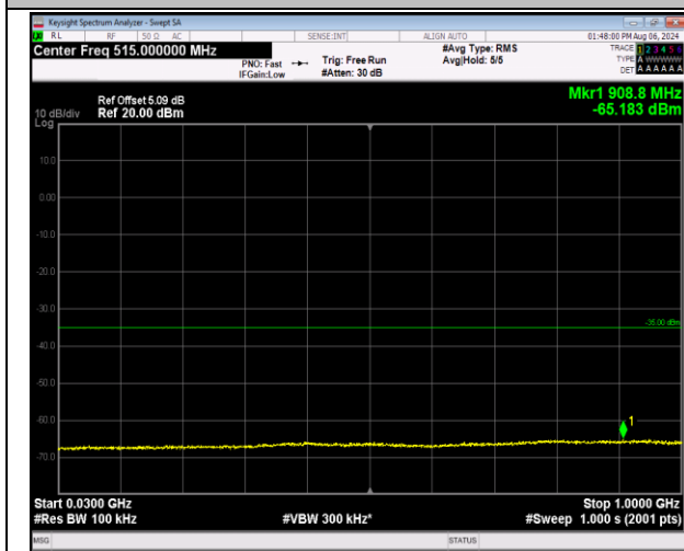
7-7-20MHz-10MHz-QPSK-QPSK-21051-21195-100RB#0 -50RB#0-30~1000MHz-PASS
