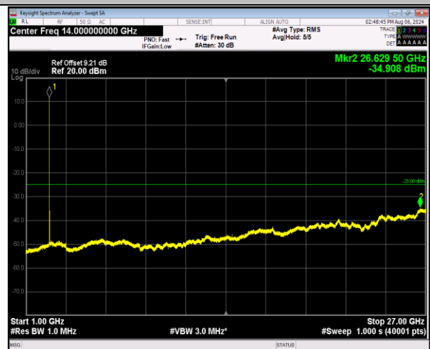
7-7-20MHz-20MHz-QPSK-QPSK-21001-21199-1RB#0-1RB#99-1000~27000MHz-PASS
