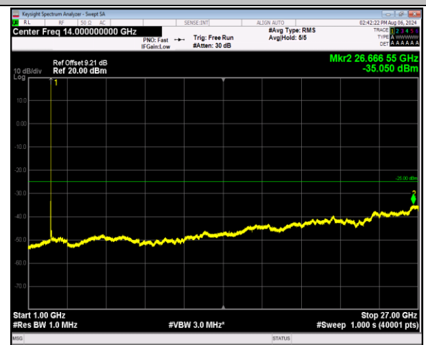
7-7-20MHz-20MHz-QPSK-QPSK-20850-21048-1RB#99-0R B#0-1000~27000MHz-PASS
