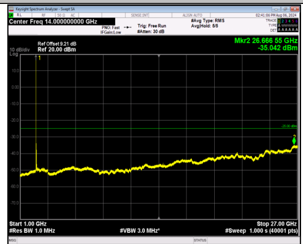
7-7-20MHz-20MHz-QPSK-QPSK-20850-21048-1RB#0-0RB#0-1000~27000MHz-PASS
