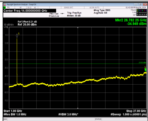
7-7-20MHz-10MHz-QPSK-QPSK-20850-20994-100RB#0-5 ORB#0-1000~27000MHz-PASS
