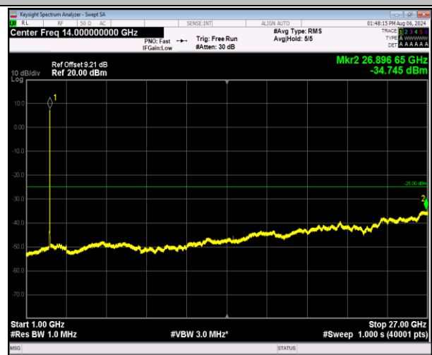
7-7-20MHz-10MHz-QPSK-QPSK-21051-21195-100RB#0-5 ORB#0-1000~27000MHz-PASS
