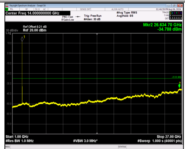
7-7-20MHz-10MHz-QPSK-QPSK-21051-21195-1RB#0-1RB#49-1000~27000MHz-PASS
