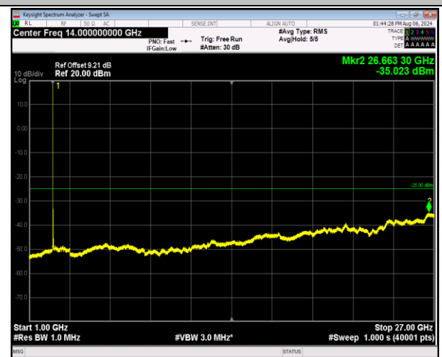
7-7-20MHz-10MHz-QPSK-QPSK-21051-21195-1RB#0-0RB #0-1000~27000MHz-PASS
