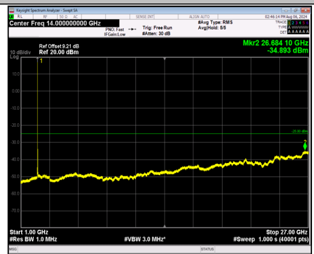
7-7-20MHz-20MHz-QPSK-QPSK-21001-21199-1RB#0-0RB #0-1000~27000MHz-PASS
