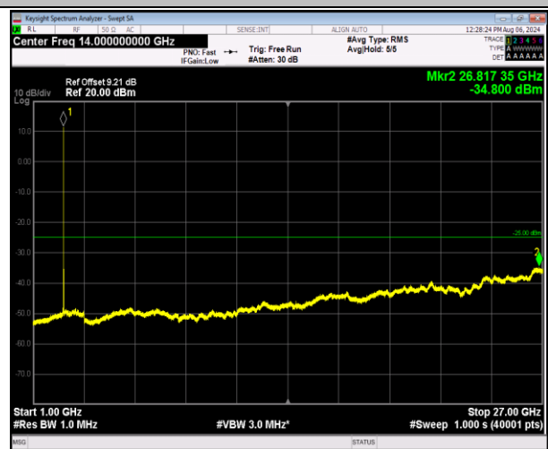
7-7-10MHz-20MHz-QPSK-QPSK-21206-21350-1RB#0-1RB #99-1000~27000MHz-PASS
