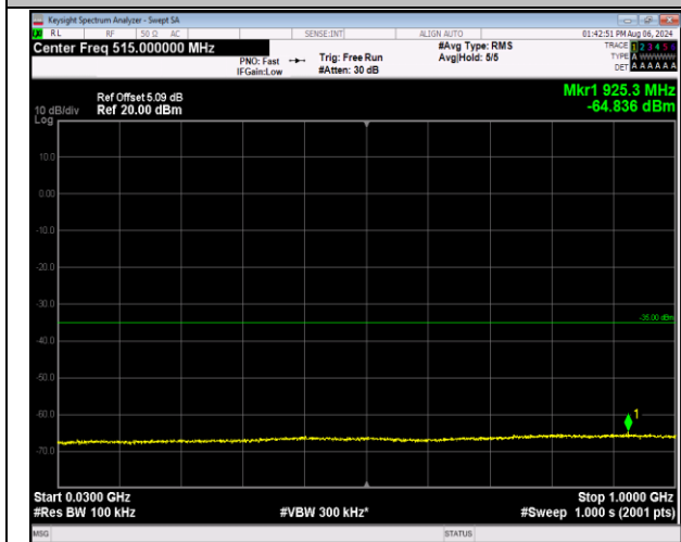
7-7-20MHz-10MHz-QPSK-QPSK-20850-20994-100RB#0 -50RB#0-30~1000MHz-PASS
