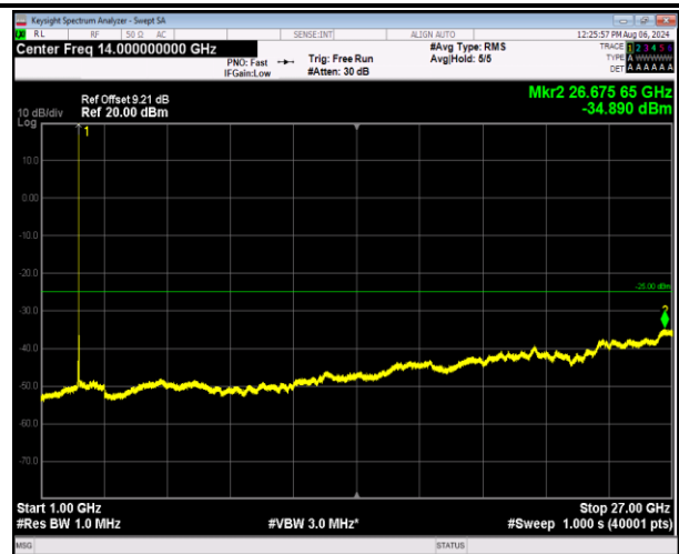
7-7-10MHz-20MHz-QPSK-QPSK-21206-21350-1RB#0-0RB #0-1000~27000MHz-PASS
