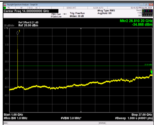
7-7-20MHz-10MHz-QPSK-QPSK-20850-20994-1RB#0-1RB #49-1000~27000MHz-PASS
