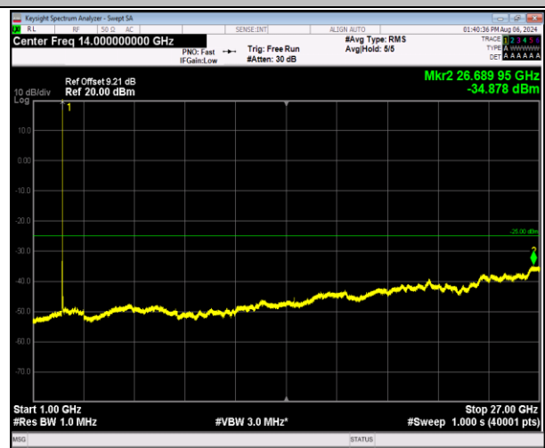
7-7-20MHz-10MHz-QPSK-QPSK-20850-20994-1RB#99-0R B#0-1000~27000MHz-PASS
