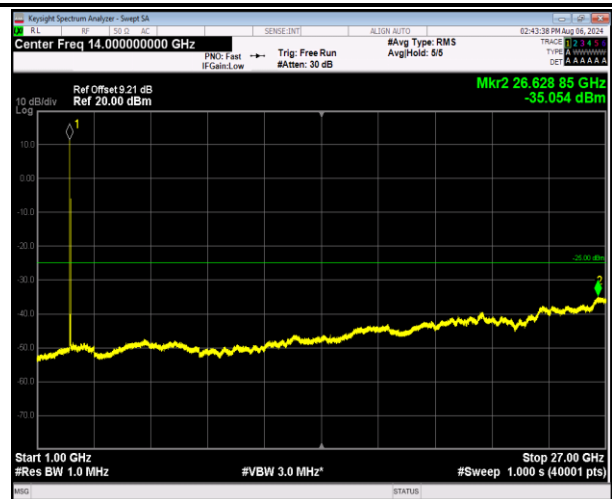
7-7-20MHz-20MHz-QPSK-QPSK-20850-21048-1RB#0-1RB #99-1000~27000MHz-PASS
