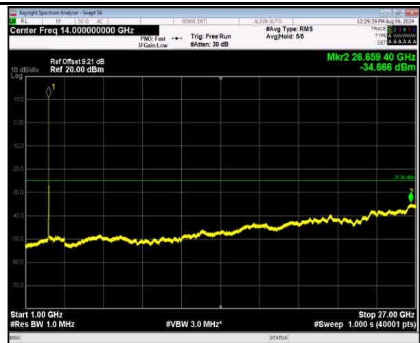
7-7-10MHz-20MHz-QPSK-QPSK-21206-21350-50RB#0-100RB#0-1000~27000MHz-PASS
